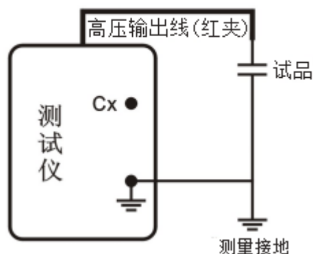
图 12 反接法
