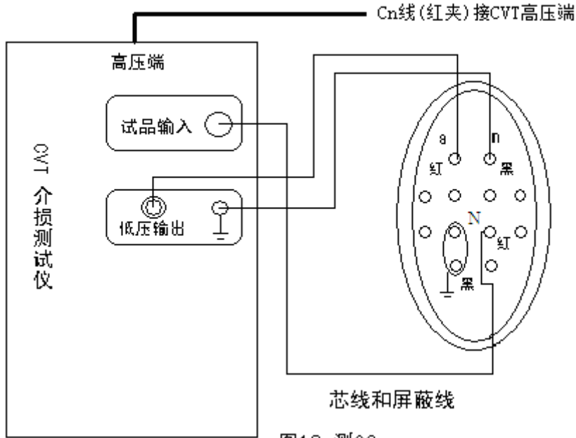
图13 测C2
