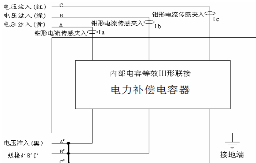
三相III型联接被试电容接线图 (10)
