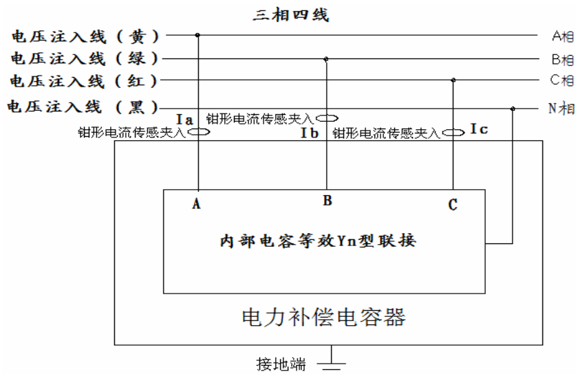
Yn 形联接被试电容接线图 (7)
