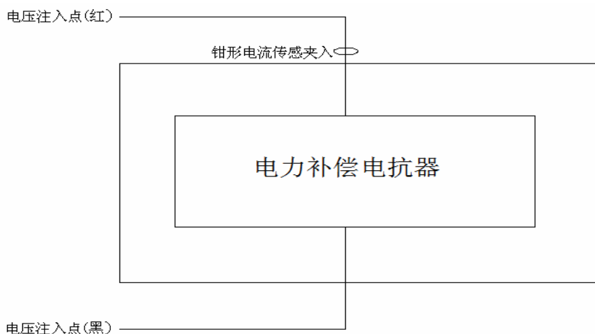
被试电抗器电感接线图 (11)
