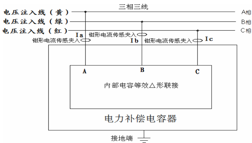
△形联接被试电容接线图
