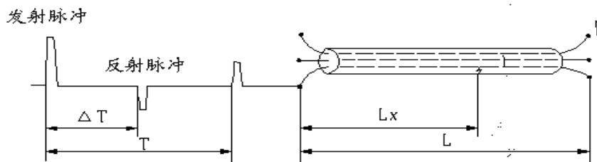
低压脉冲测试原理图
