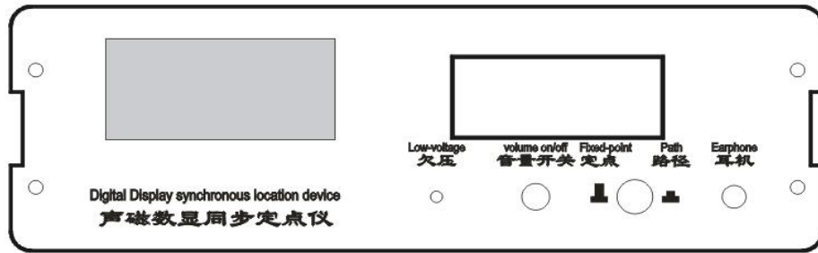
前面板示意图
