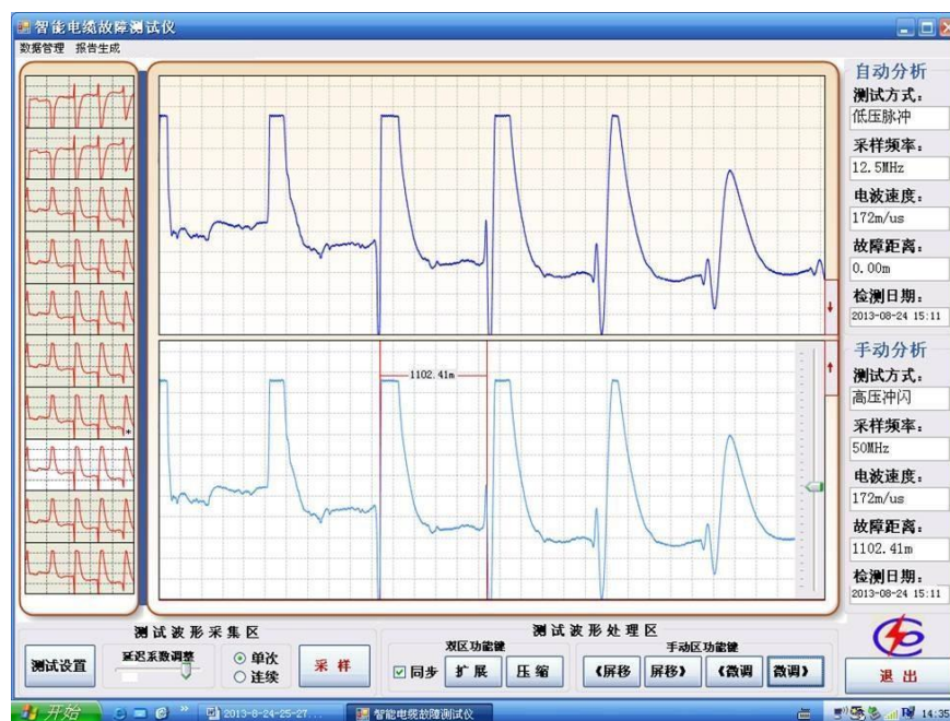
图 20 仪器在冲闪法时故障点的测试波形
