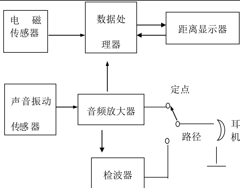
图 24 原理框图
