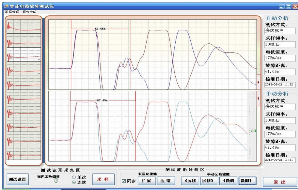
图 19 仪器在多次脉冲法测试某一近始端故障时得波形
