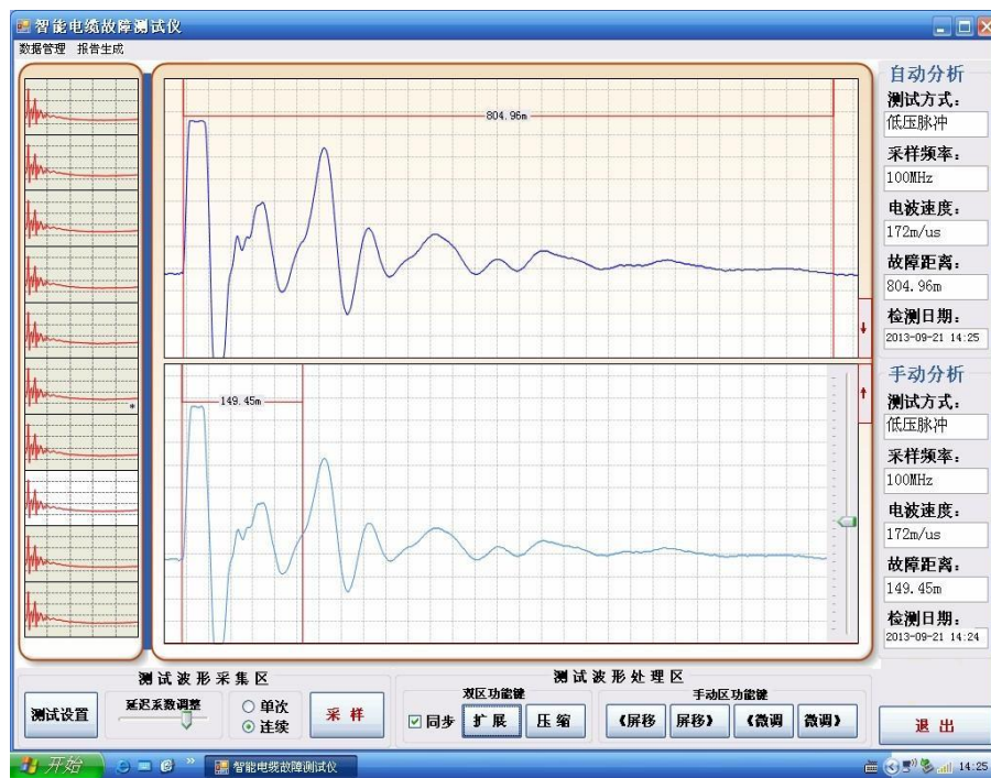
图 17 仪器在多次脉冲法时手动去卡的一个电缆全长的测试波形
