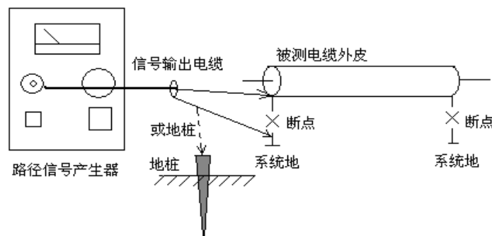
图 26 仪器连线示意图
