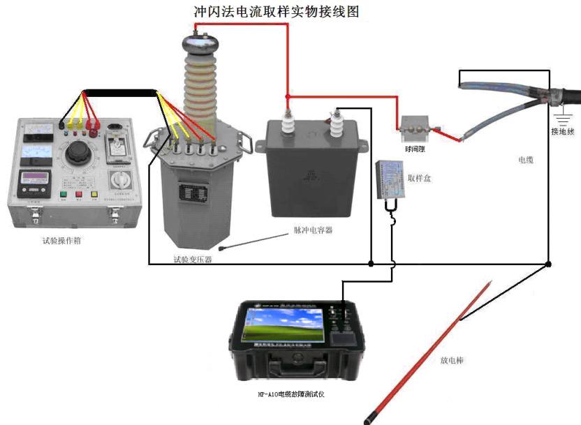
图 21 冲闪法现场故障测试接线示意图（配试验变压器现场）
