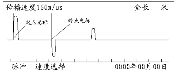
低压脉冲测短路、低阻故障波形
