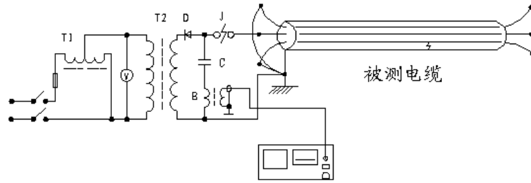
冲闪法电流取样原理图
