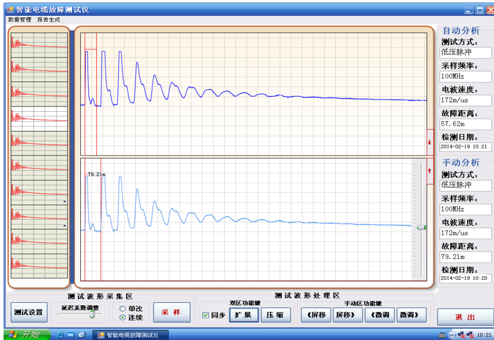
图 10 低压脉冲法测得开路故障或开路全长波形
