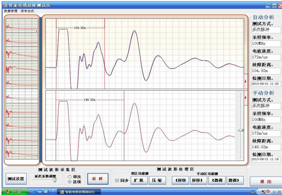
图 14 仪器在多次脉冲法时延迟系数过大的测试波形
