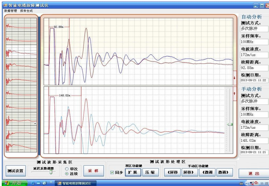
图 16 仪器在多次脉冲法时压缩的多次脉冲波形
