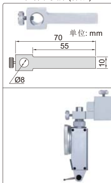
杠杆表支架(标配)
