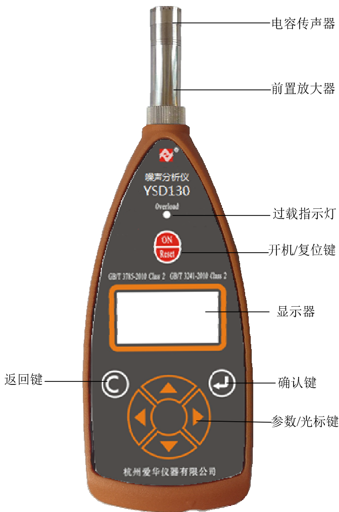
图 3-1 主机正面
