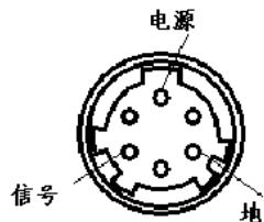
图 3-3 X9 插座
