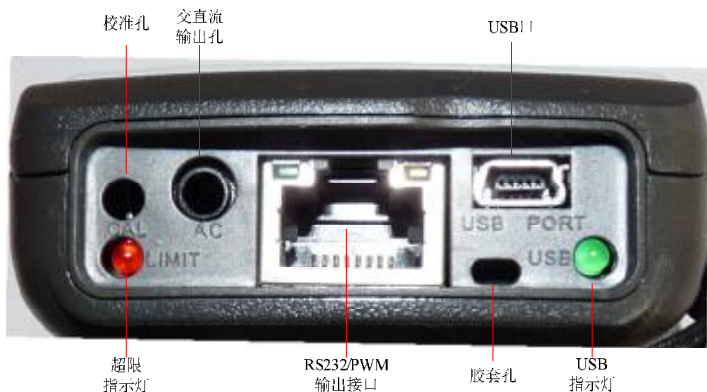
图 3-4 接口
