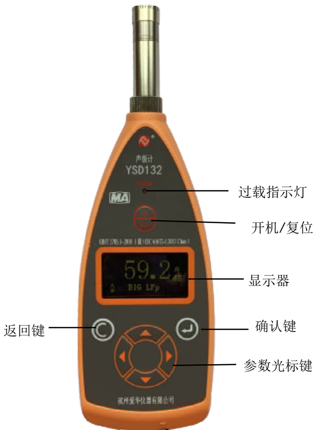
图 3-1 主机正面
