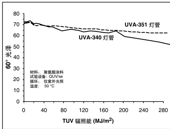
图7-波长对聚氨酯涂料失光的影响。在相同焦耳数下, 不同光谱功率分布的灯管并不总是引起不同的失光速率。
