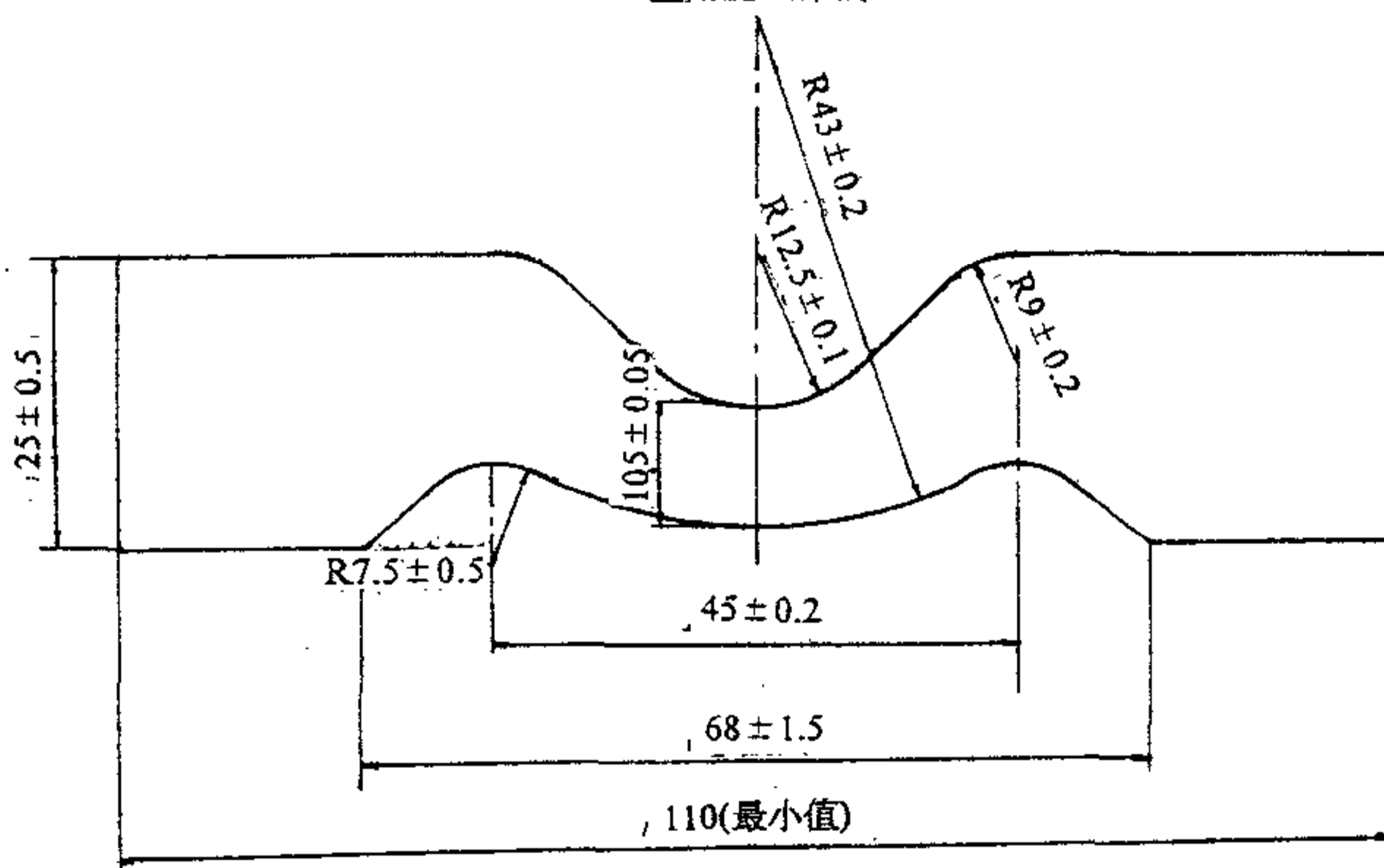
图3 新月型试样裁刀
