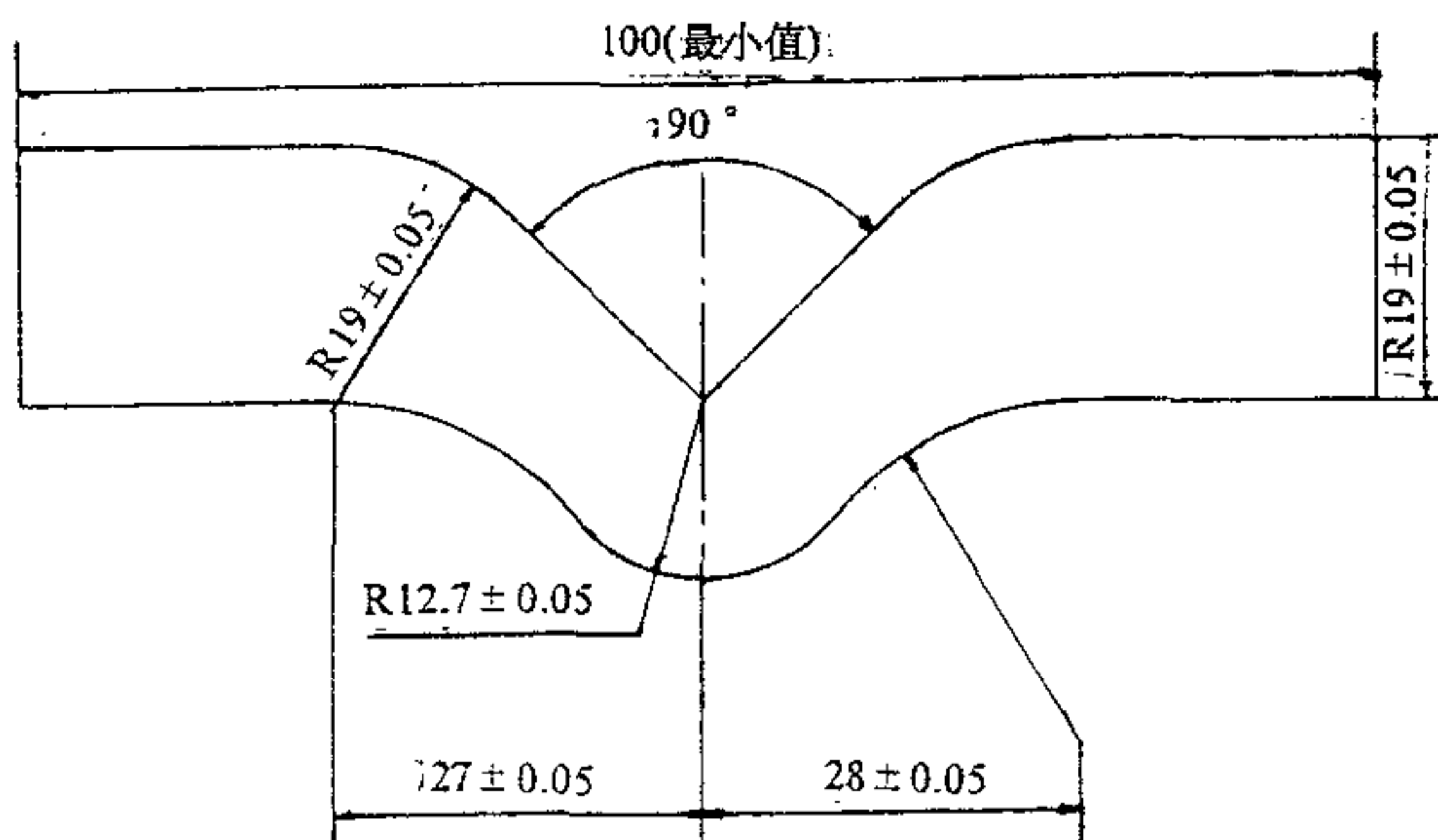
图2 直角型试样裁刀
