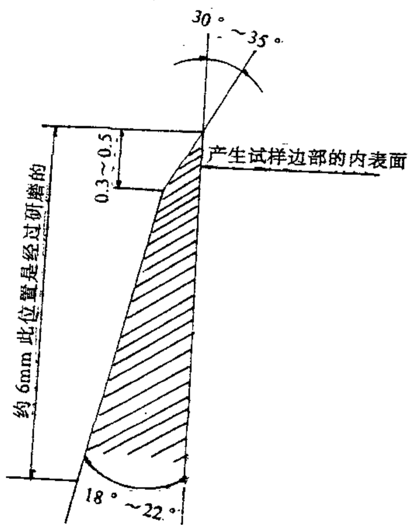
图4 裁刀的研磨部位及刃口角度
