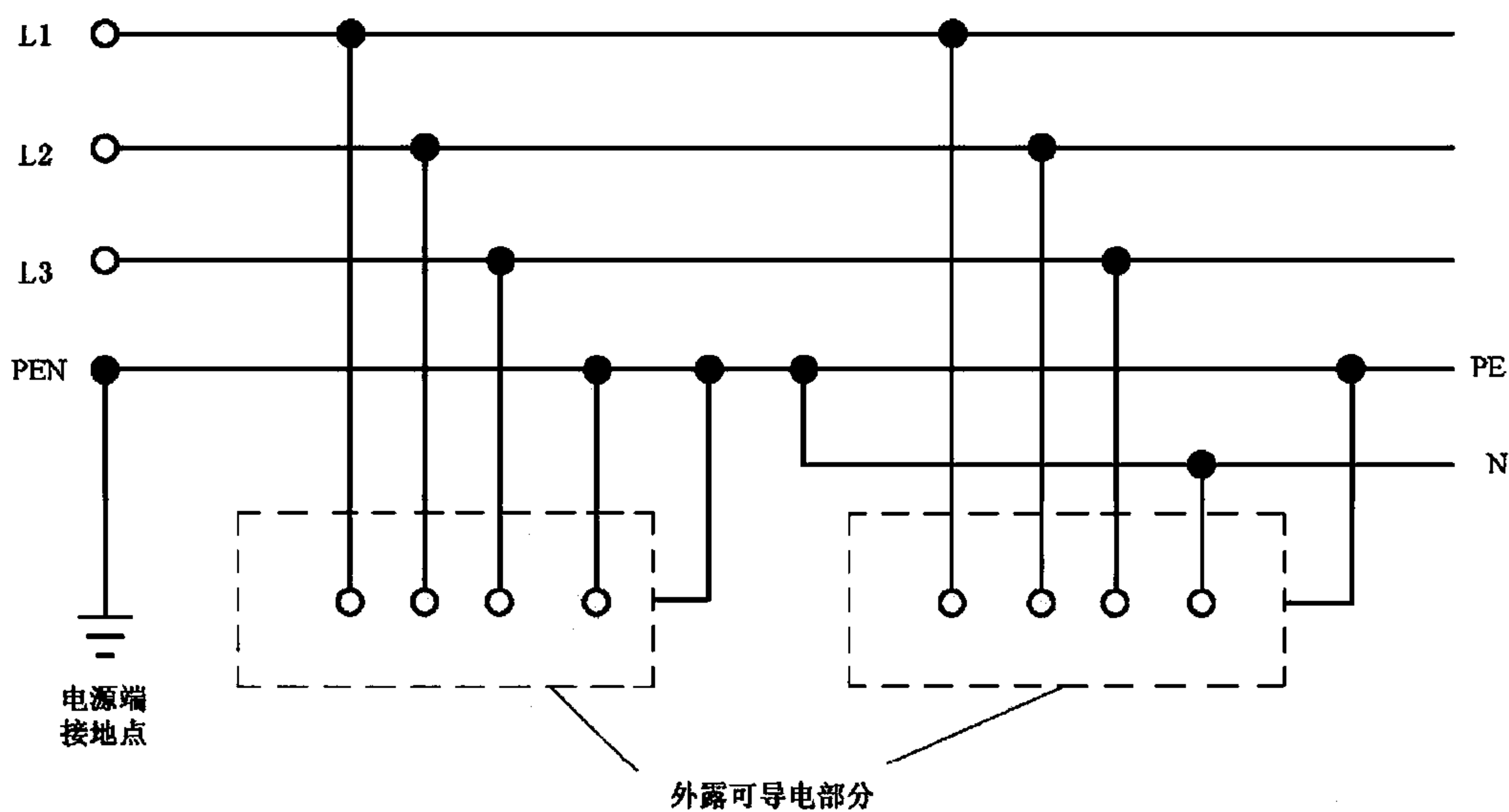
图 3 TN-C-S 系统
