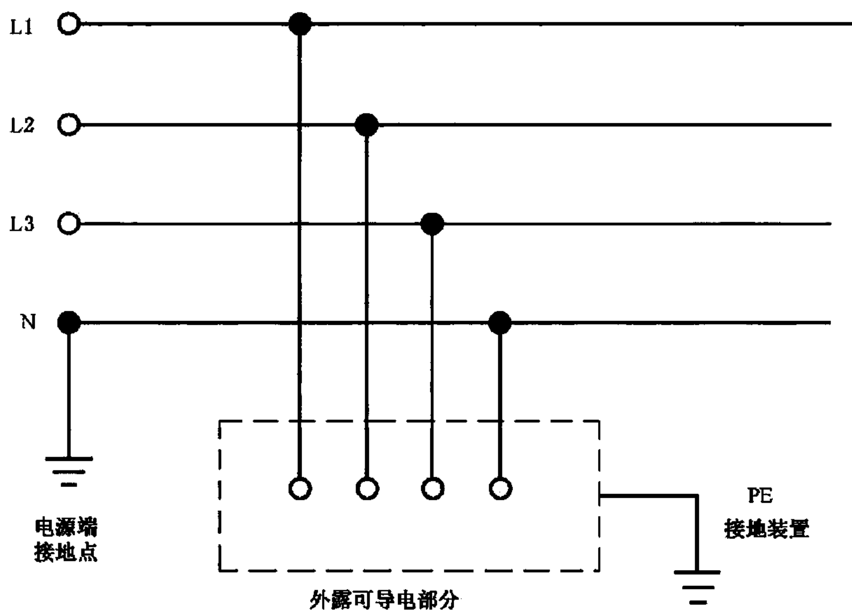
图 4 TT 系统
