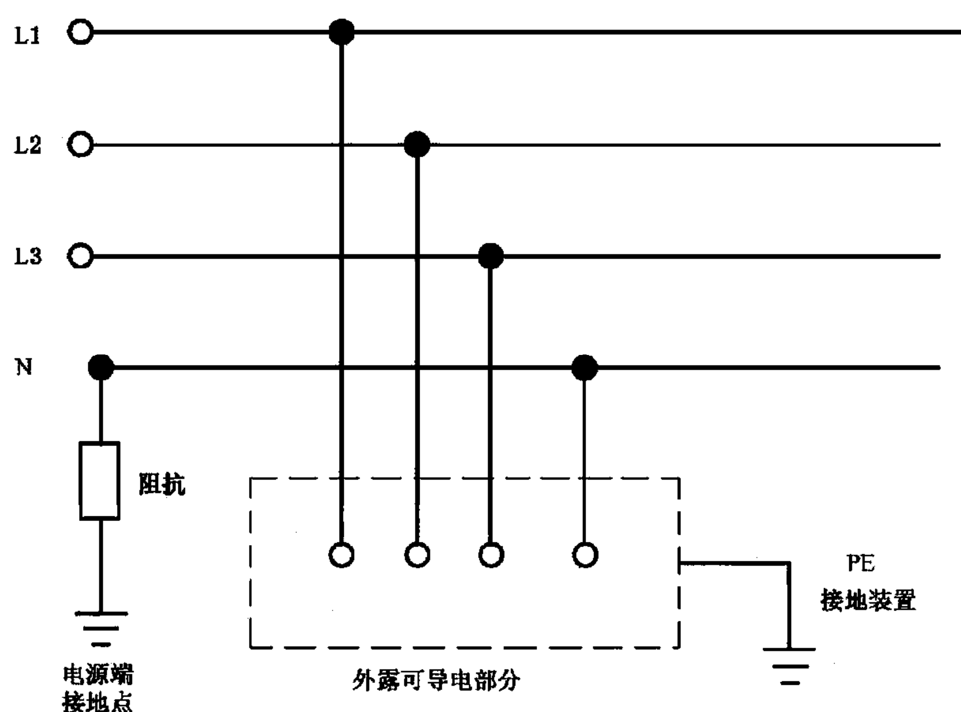
图 5 IT 系统
