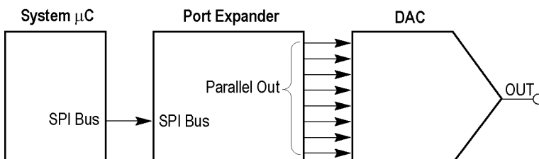
图 2: 混合信号链框图
