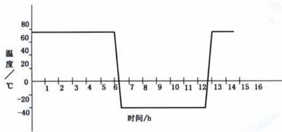
图 1 温度循环流程示意图
