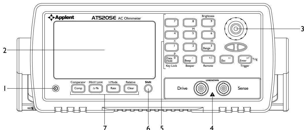
图 3-1 前面板
