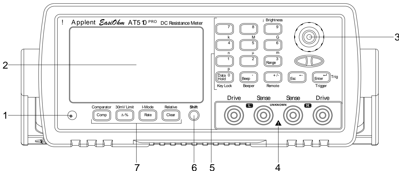
图 3-1 前面板
