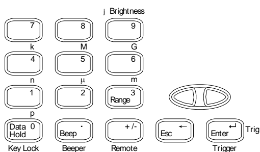
图 3-3 键区二
