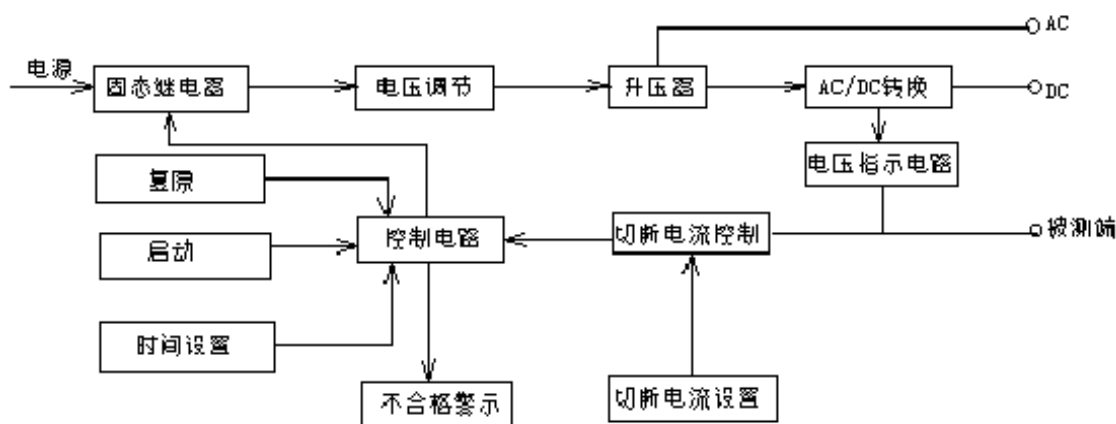
5-1 框图
