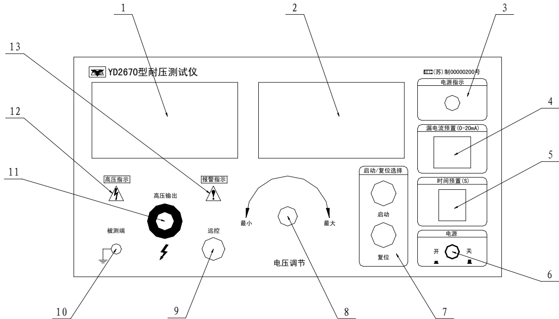
2670 前面板图
