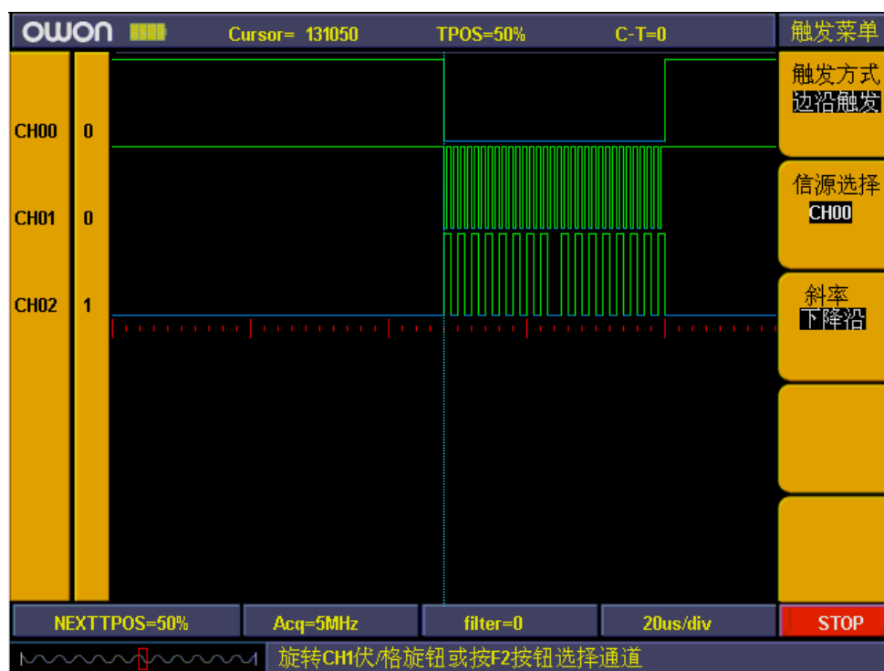
图81：边沿触发设置
