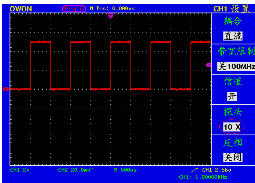
图 23: 调节探头比例
