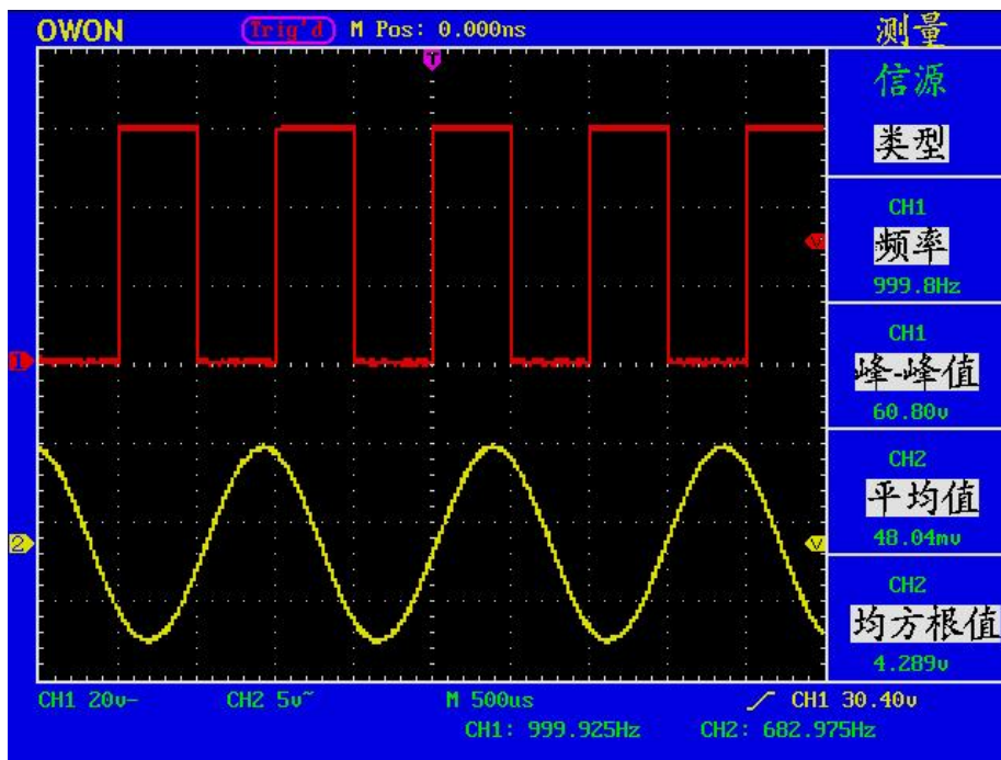
图69：自动测量
