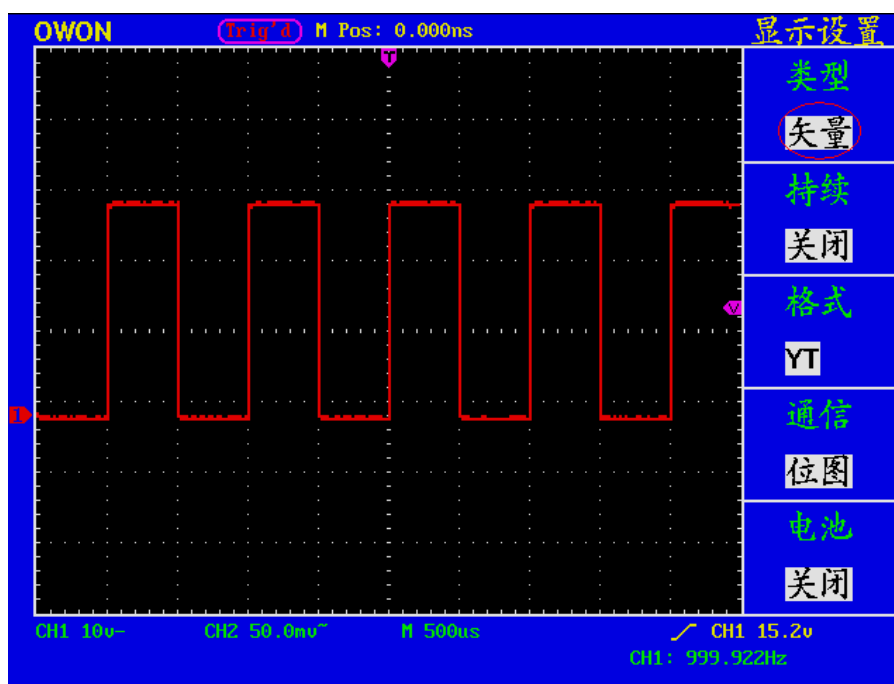
图 57: 矢量显示类型
