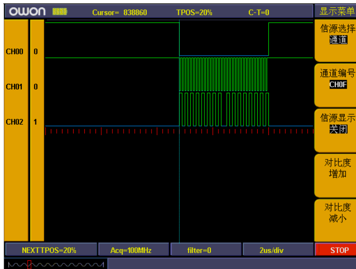
图15: 显示设置
