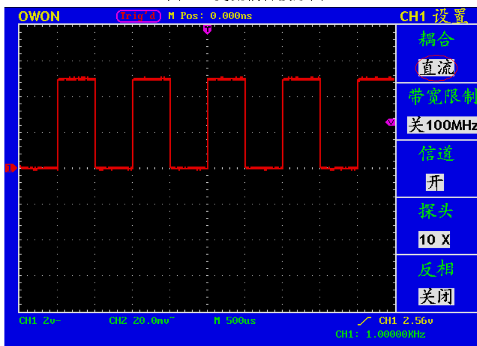
图 22：直流耦合波形图
