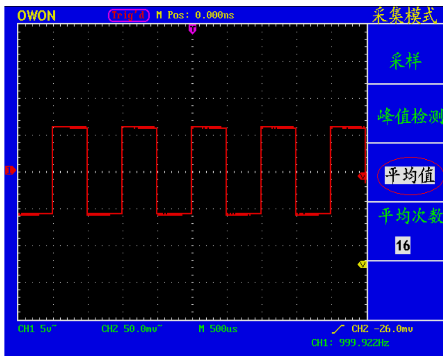
图55: 平均次数为16次平均值方式，去除噪声后的显示波形。
