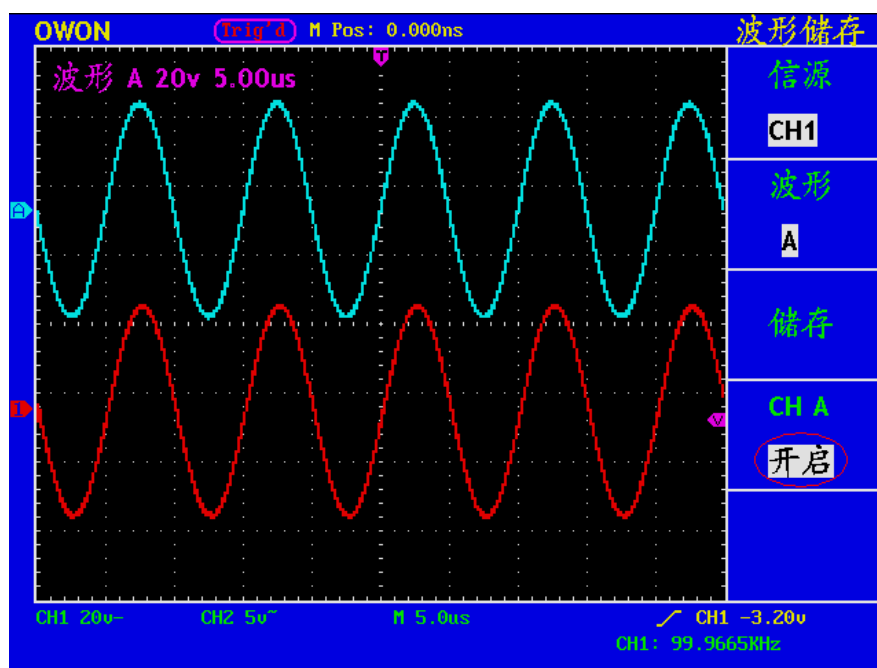
图63：波形储存
