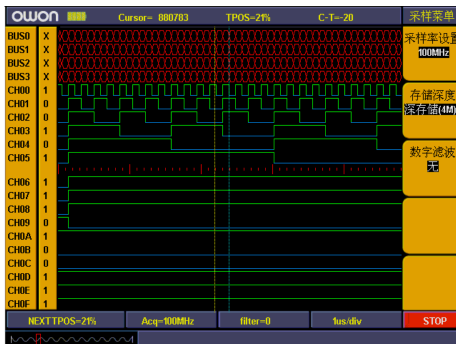
图79:采样设置
