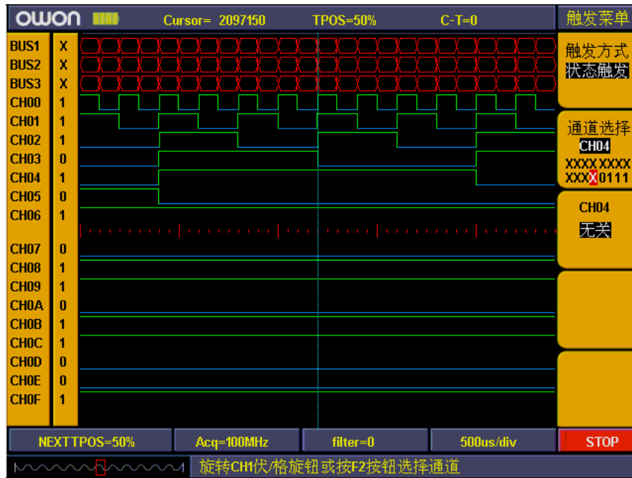
图85：状态触发
