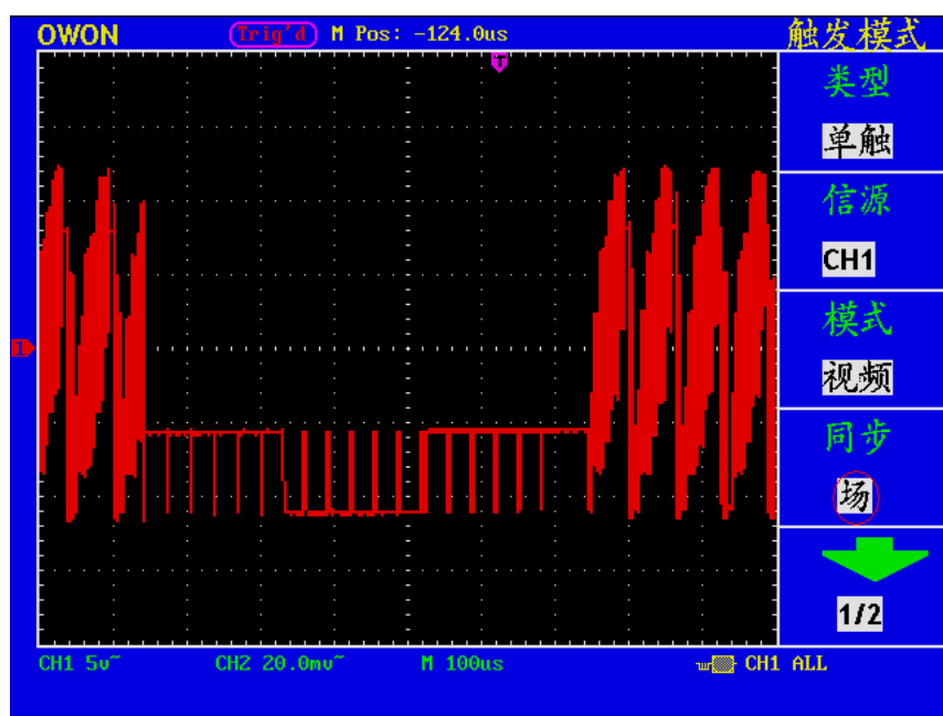
图 114 视频场触发波形
