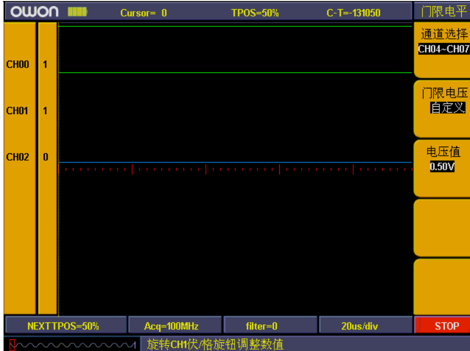
图 93：门限电平自定义设置
