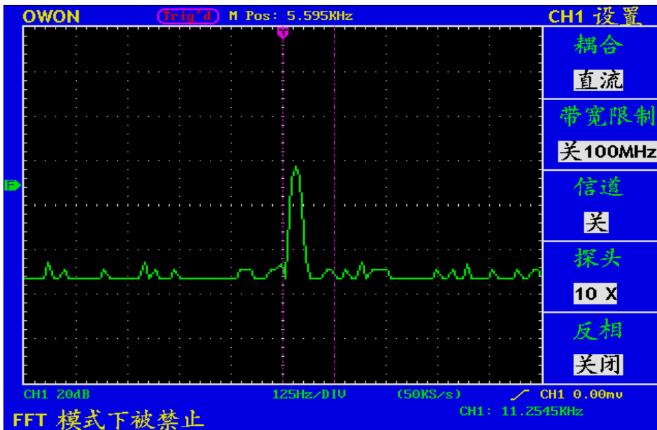
图23 CH1/2通道在FFT模式下被禁止
