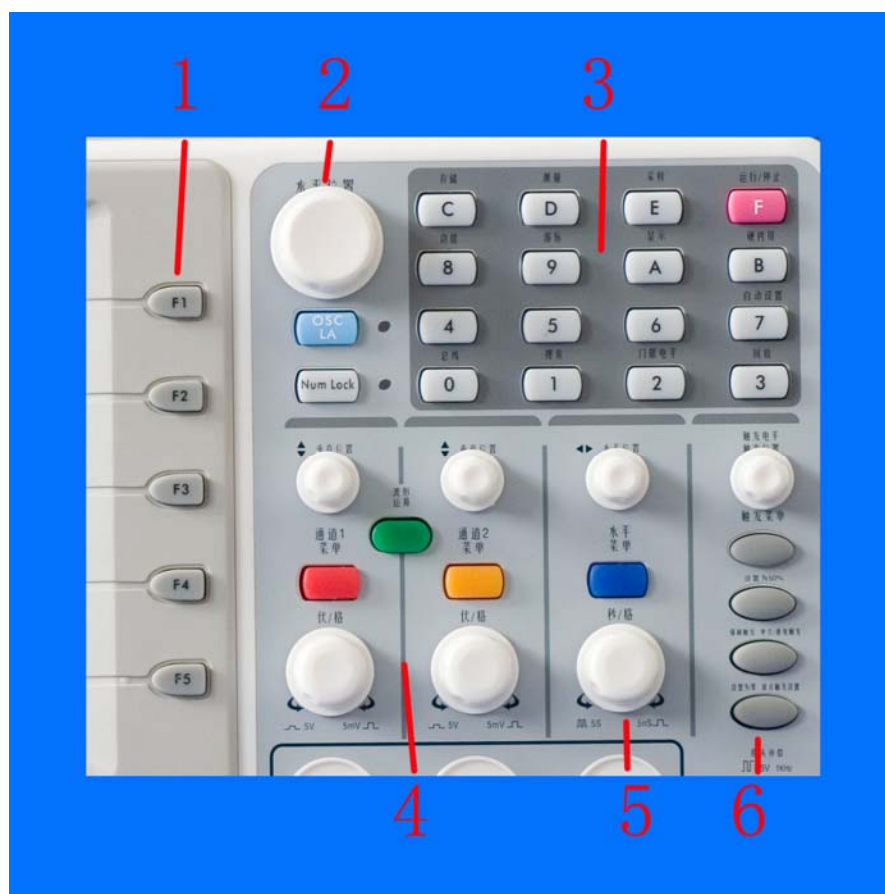
图 2 按键和旋钮控制区说明图
