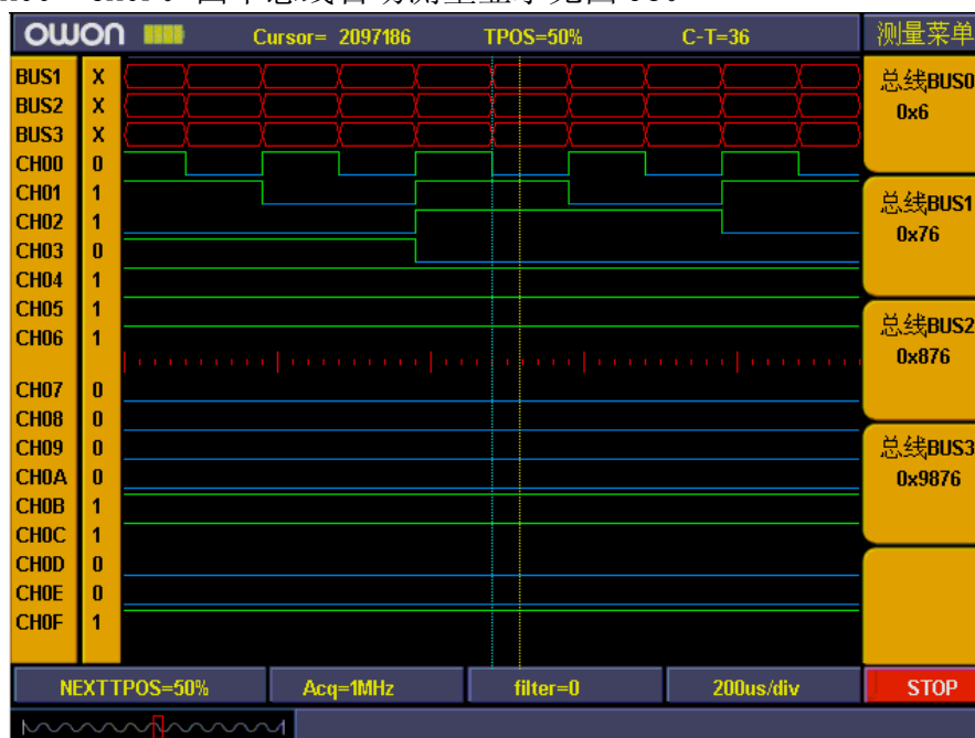
图 98：总线测量
