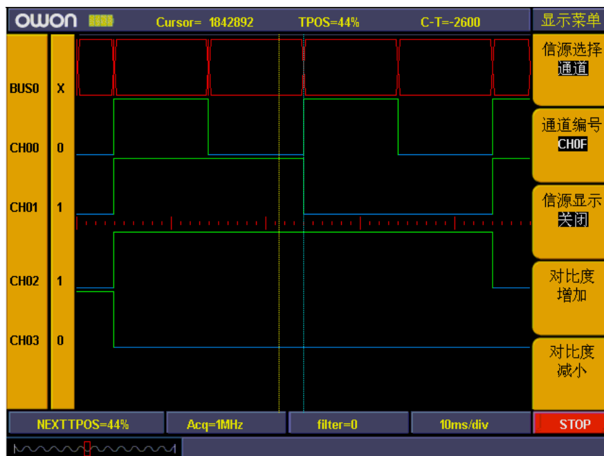
图 95: 显示设置
