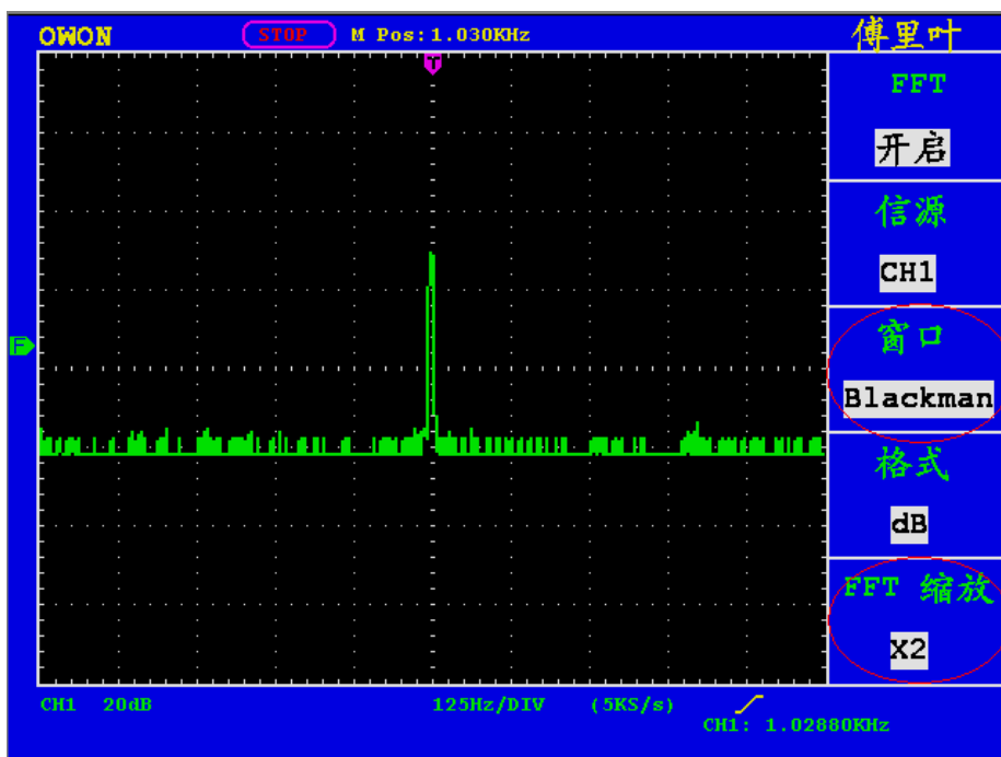
图28. BLACKMAN窗
