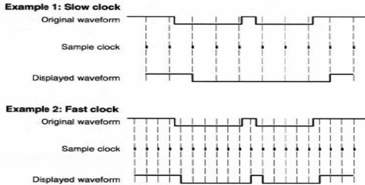
图18：采样与记录波形的关系
