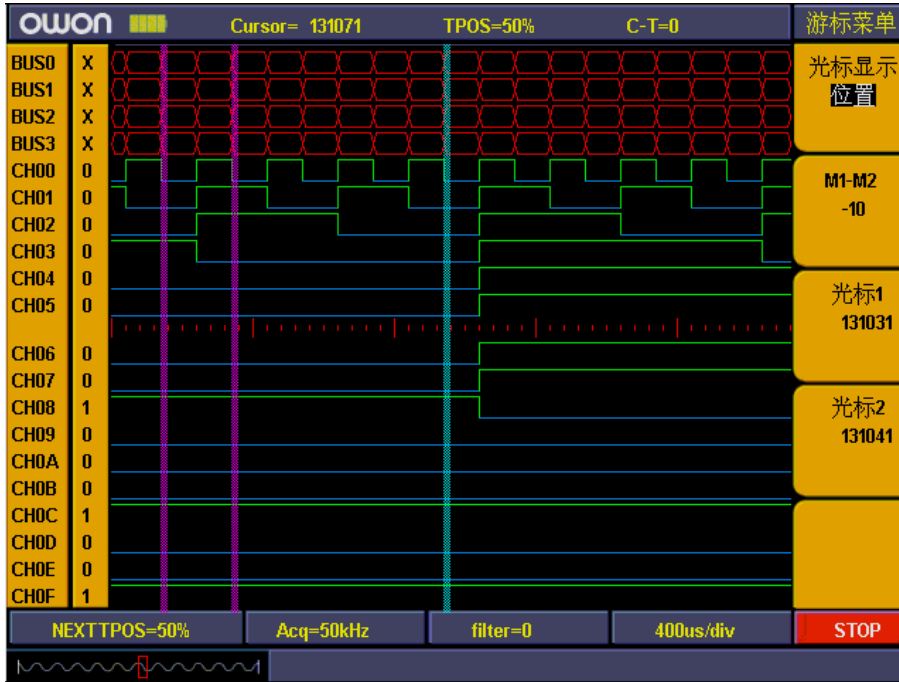
图 107：光标位置测量
