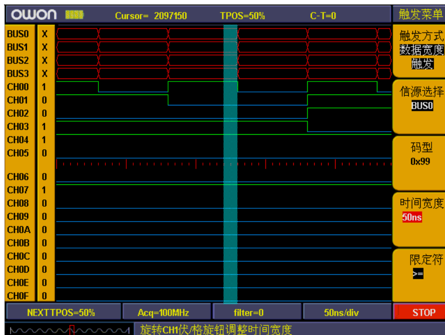
图91：数据宽度触发
