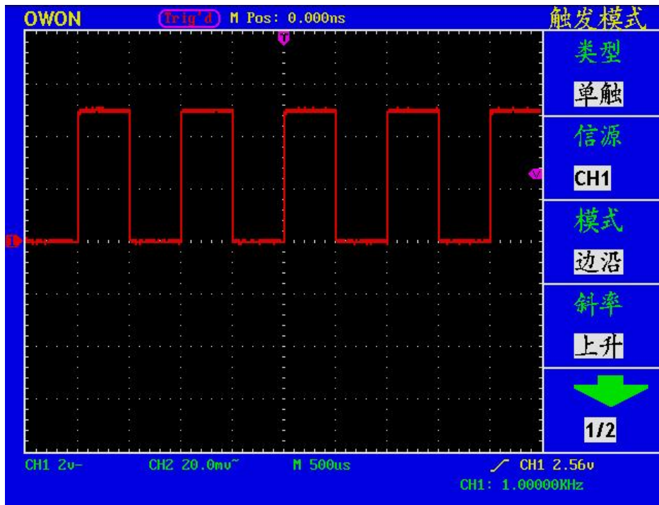
图 4：自动设置
