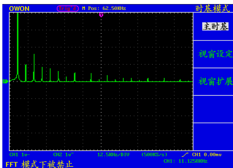
图36 FFT模式下视窗设定被禁止
