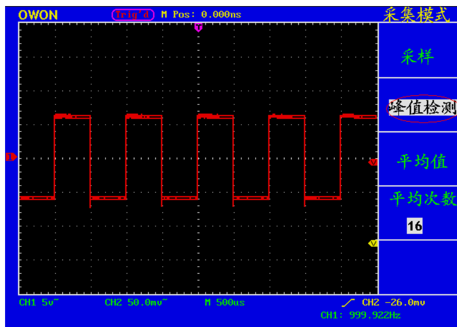
图 53: 峰值检测方式，可检测到方波下降沿的毛刺，噪声比较大。
