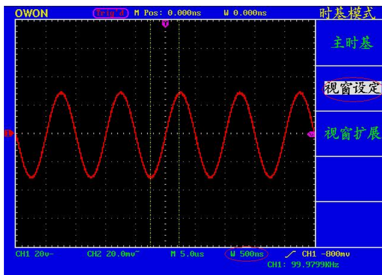
图 35 视窗设定
