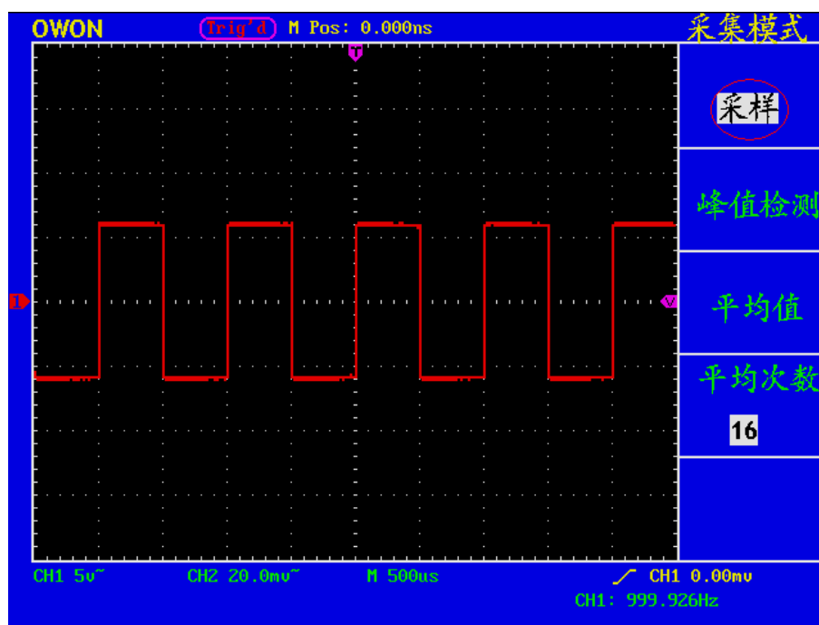
图 54: 普通采样方式显示，检测不到毛刺。
