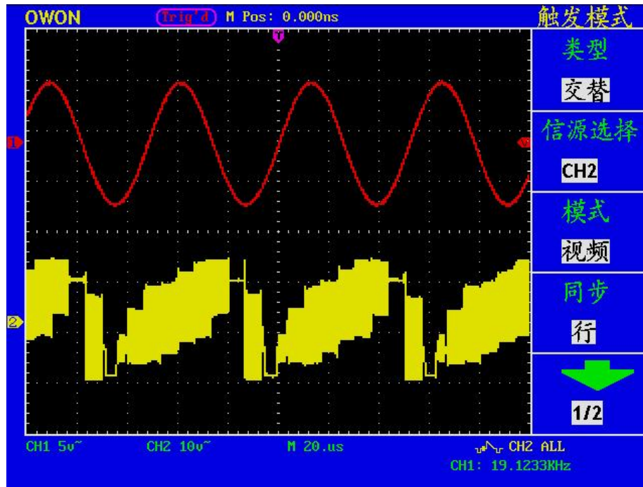
图 51: 交替触发波形
