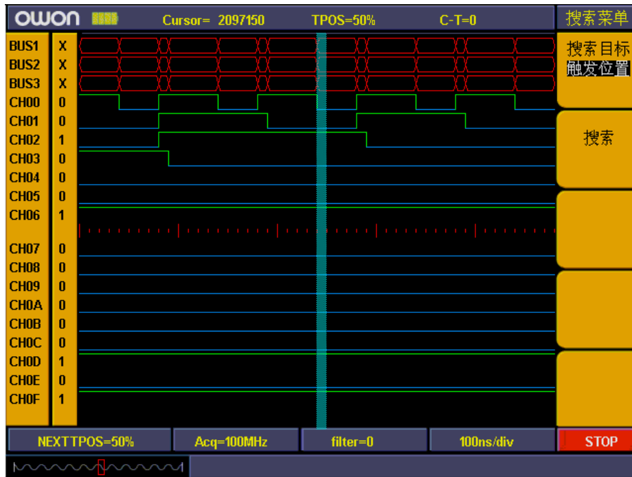
图 95：搜索触发位置
