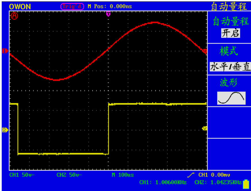
图 77: 自动量程 水平/垂直模式单周期波形图
