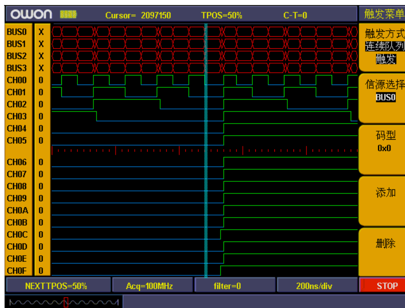
图87：连续队列触发
