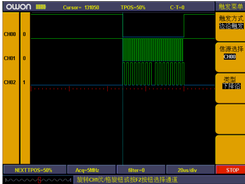
图16:边沿触发设置
