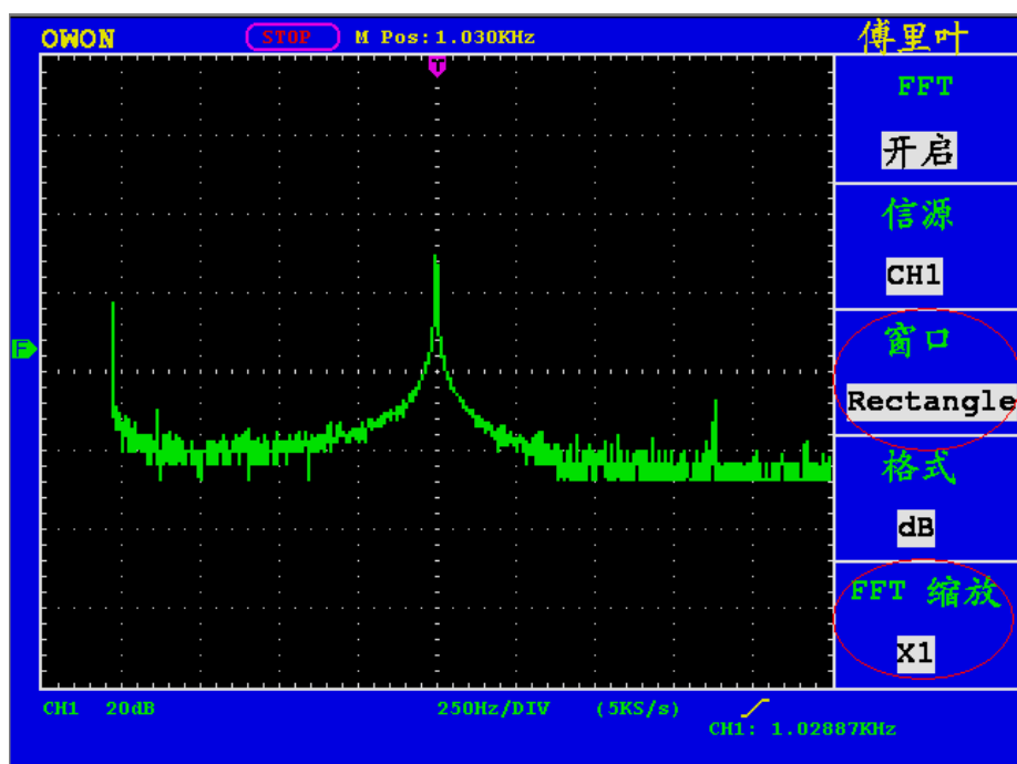
图30. RECTANGLE 窗
