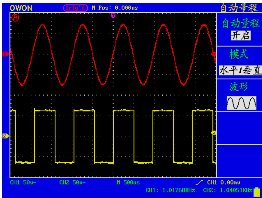
图 76：自动量程 水平/垂直模式多周期波形图
