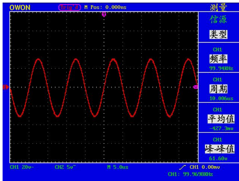
图108：自动测量波形
