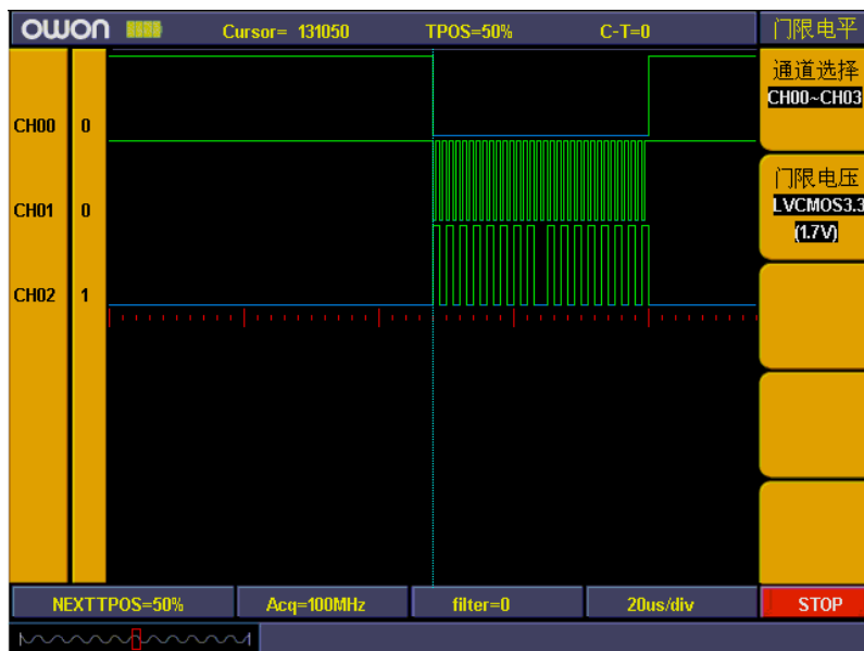
图17:门限电平设置
