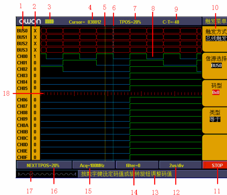
图 12: 逻辑分析仪用户界面
