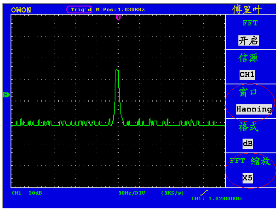
图29. HANNING 窗
