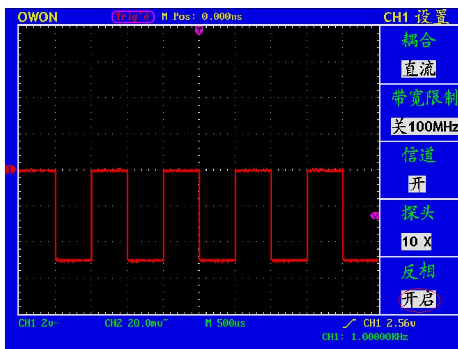
图 26: 反相的波形
