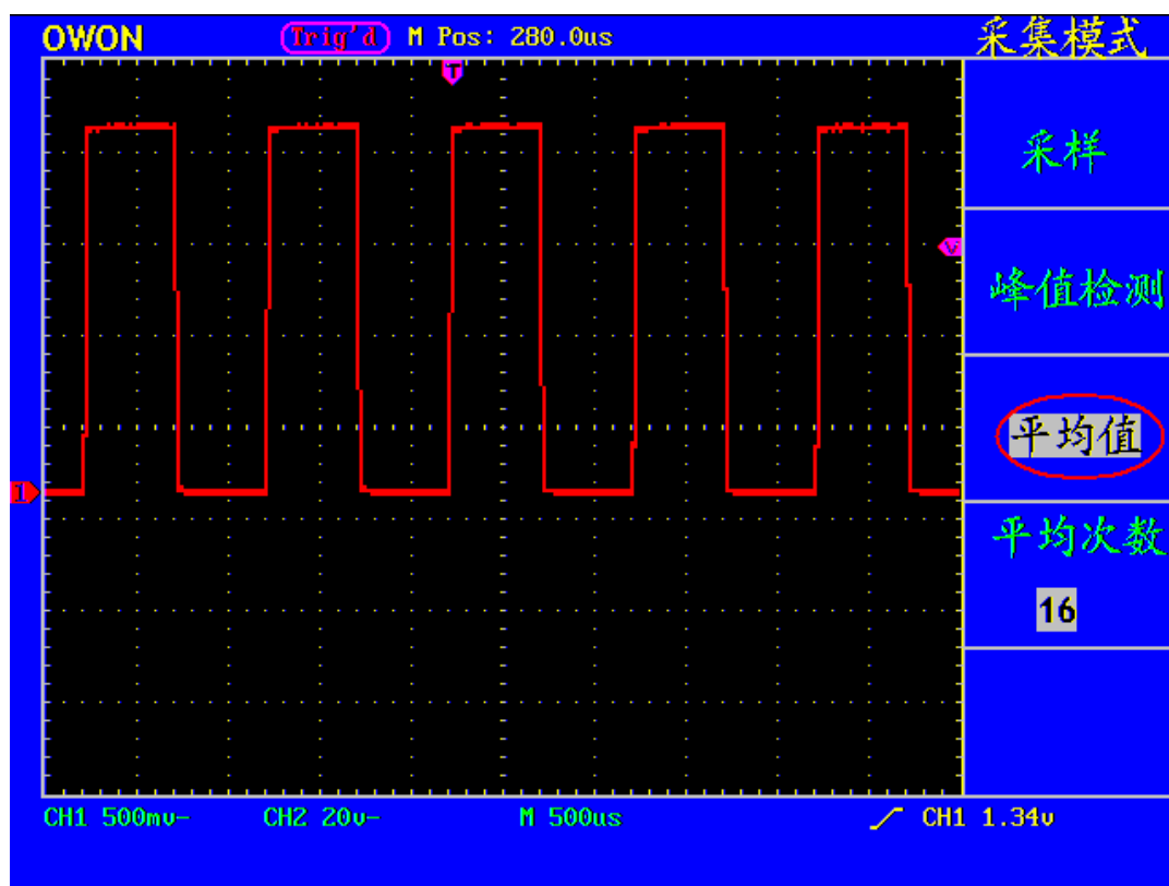
图 46: 平均次数为16次平均值方式, 去除噪声后的显示波形。
