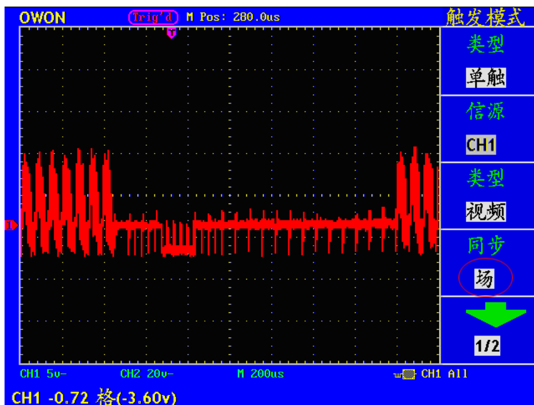
图 70 视频场触发波形
