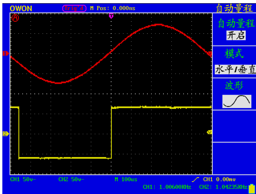
图 63 自动量程---水平/垂直模式单周期波形图
