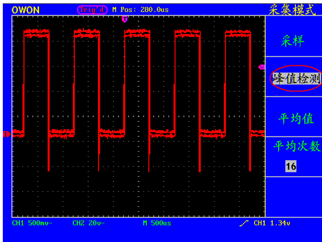
图 44: 峰值检测方式, 可检测到方波下降沿的毛刺, 噪声比较大。
