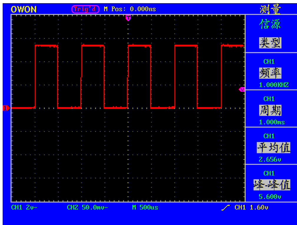
图 64: 自动测量波形
