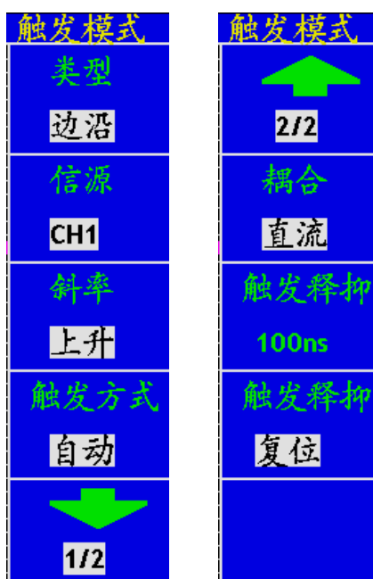
图30：边沿触发菜单
