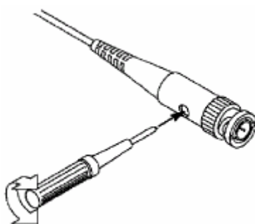
图 8：探头调整
