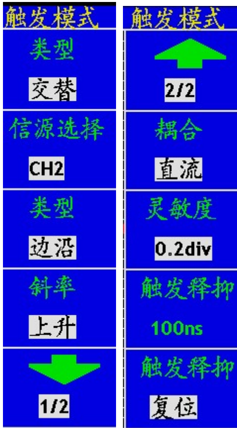
图40：交替边沿触发菜单
