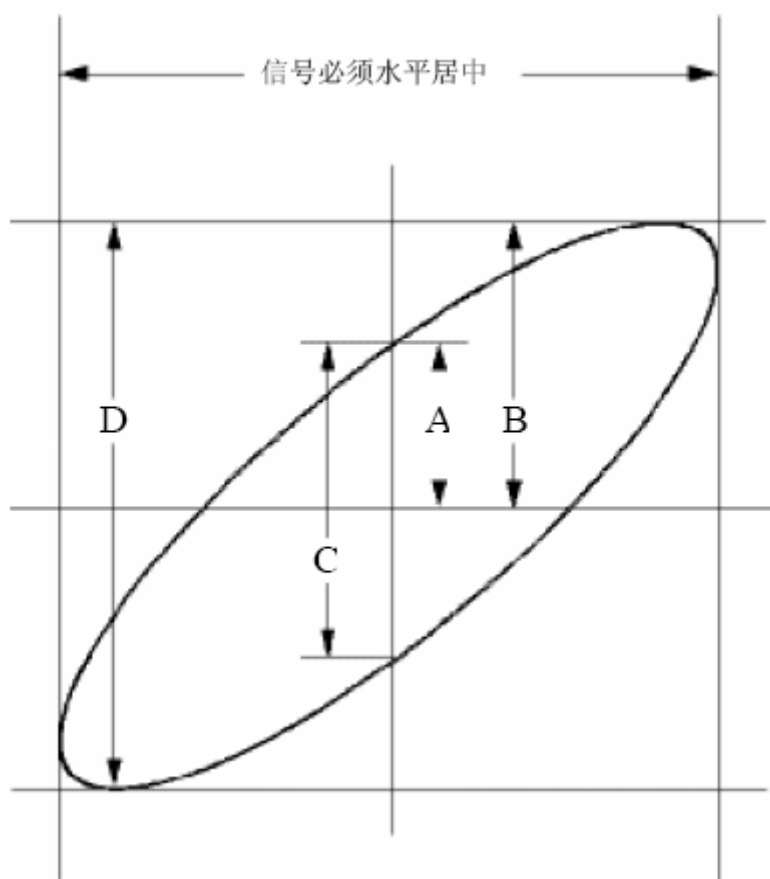
图 69 李沙育 (Lissajous) 图形
