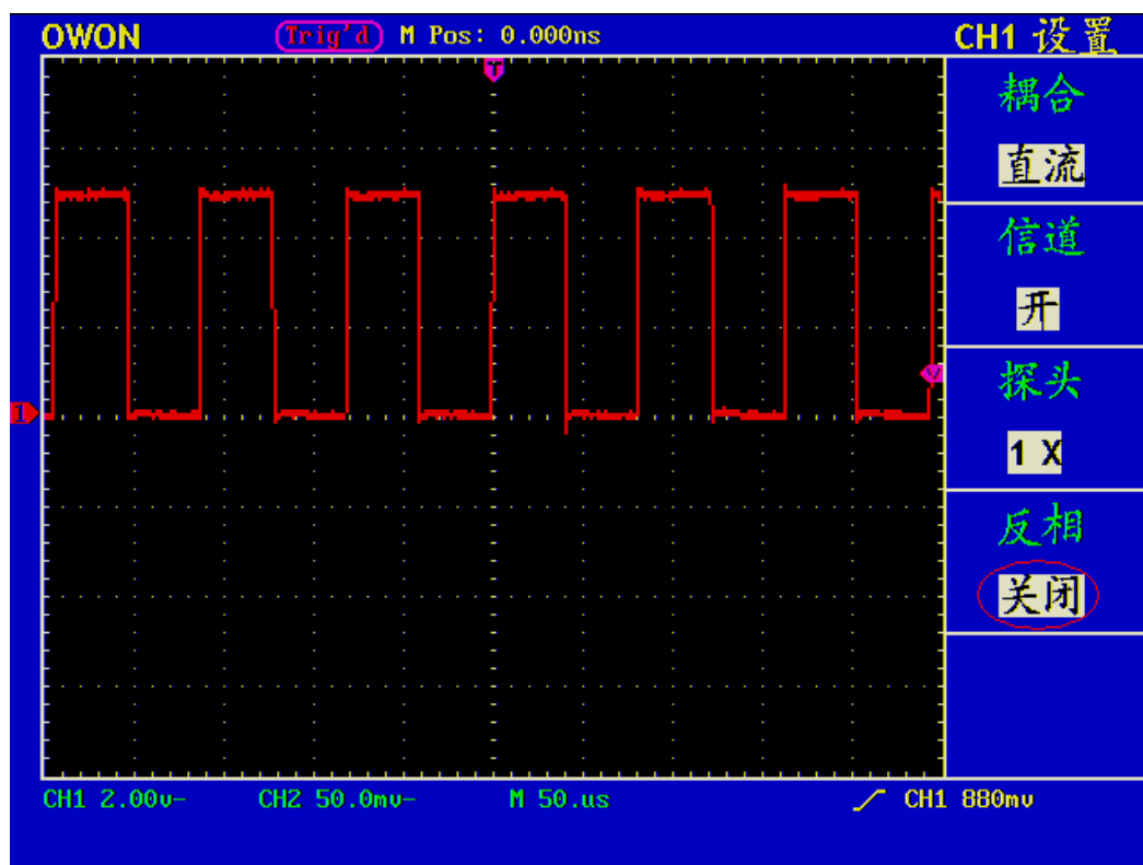
图 18 未反相的波形
