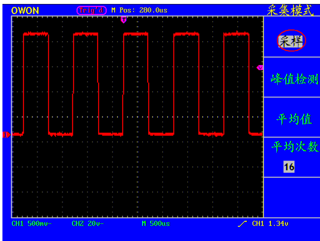
图 45: 普通采样方式显示, 检测不到毛刺。
