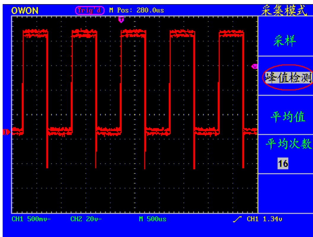
图 67： 含噪声信号的波形
