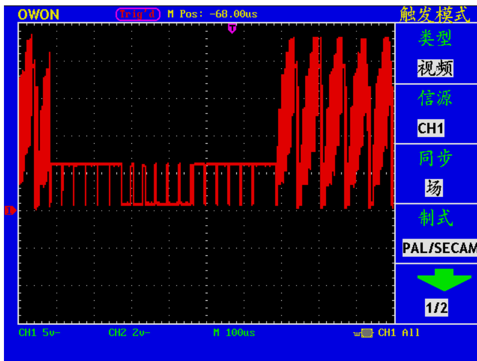
图 34 视频场触发波形
