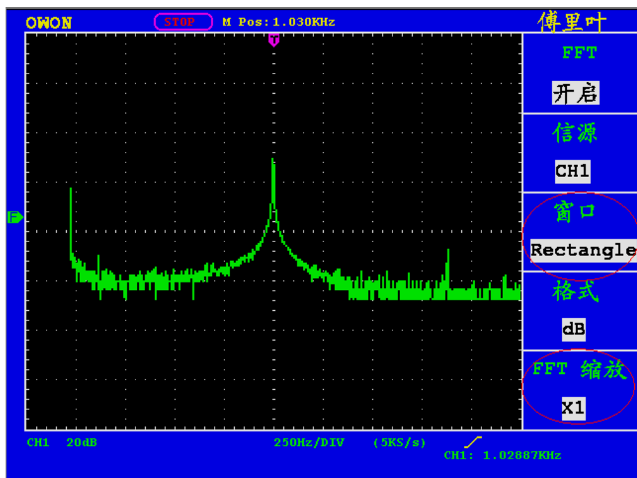
图23. Rectangle窗
