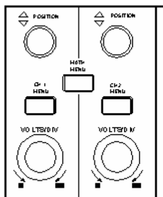
图 11：垂直控制区
