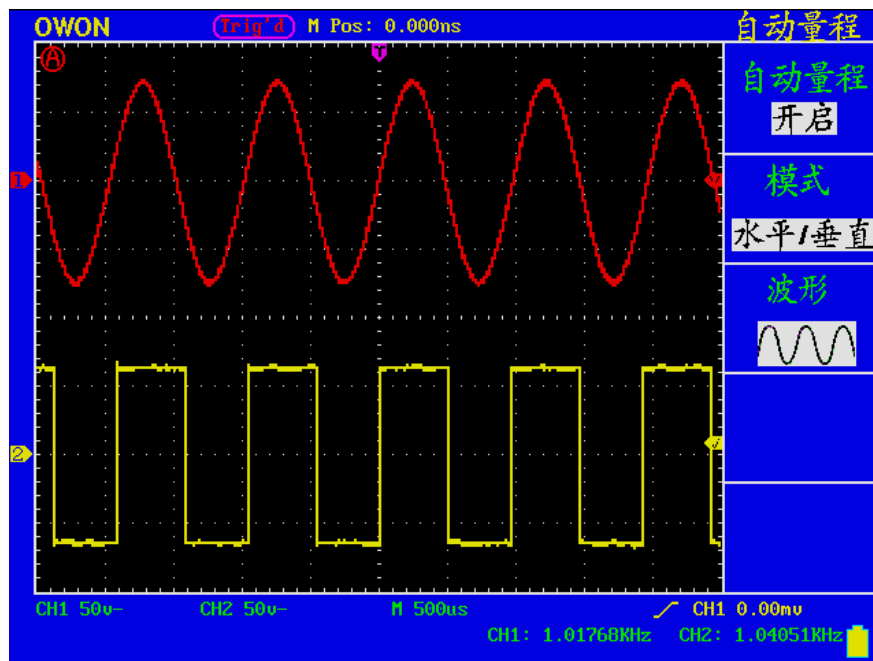
图 62 自动量程---水平/垂直模式多周期波形图
