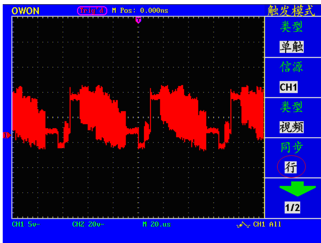
图 71 视频行触发波形
