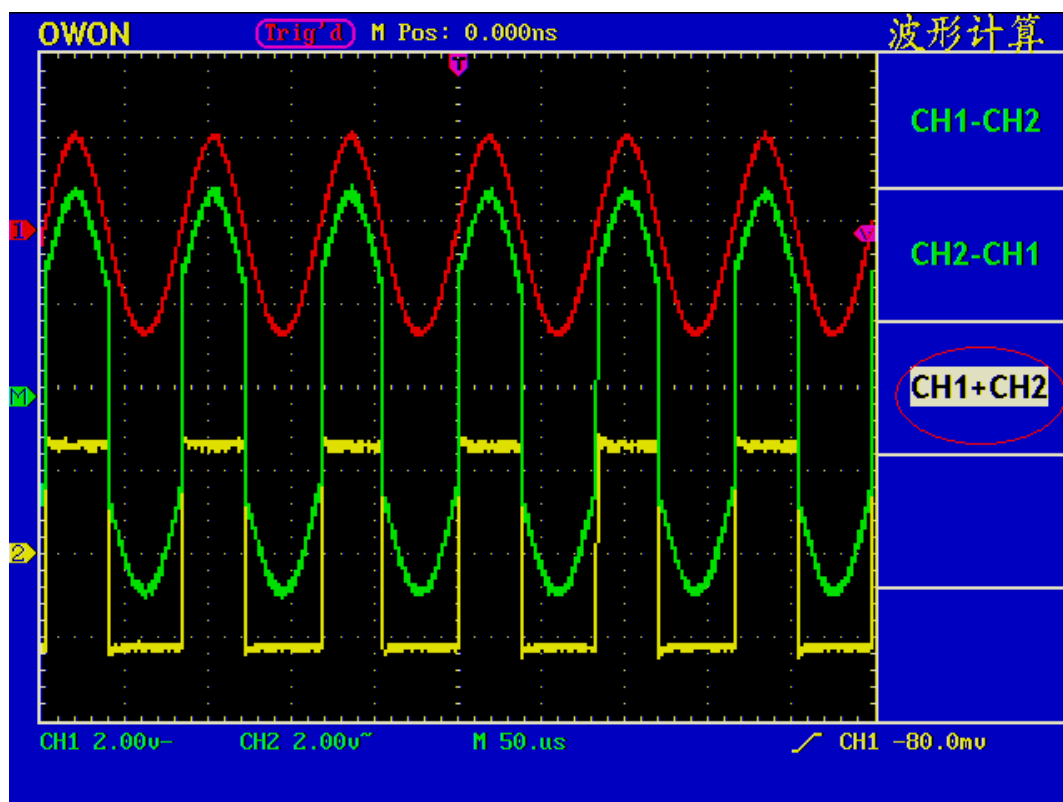
图 20 CH1+CH2 数学运算波形
