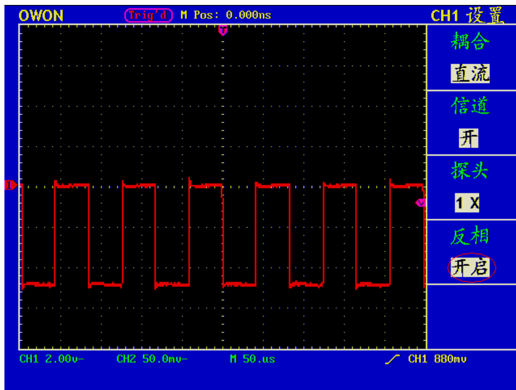
图 19 反相的波形
