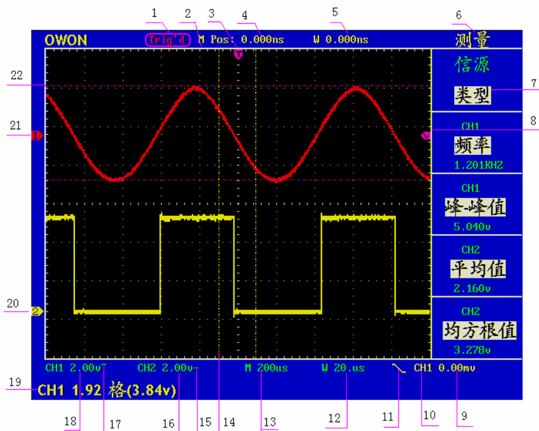
图 3 显示界面说明图
