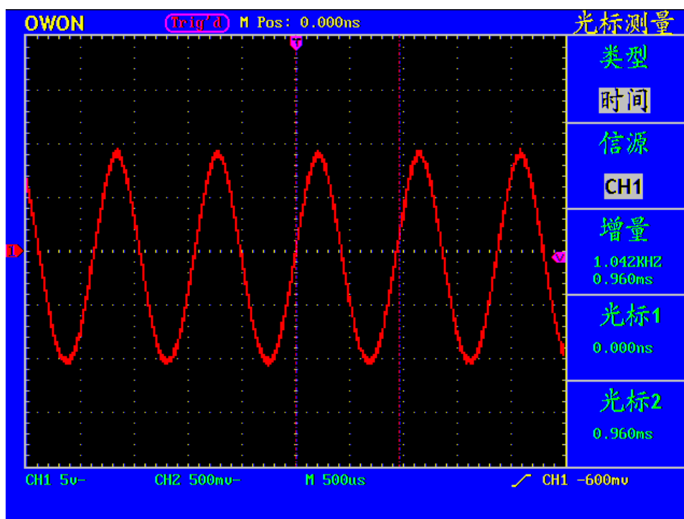
图61： 时间光标测量波形
