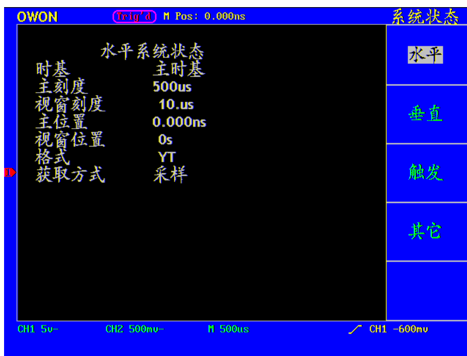
图56：水平系统状态
