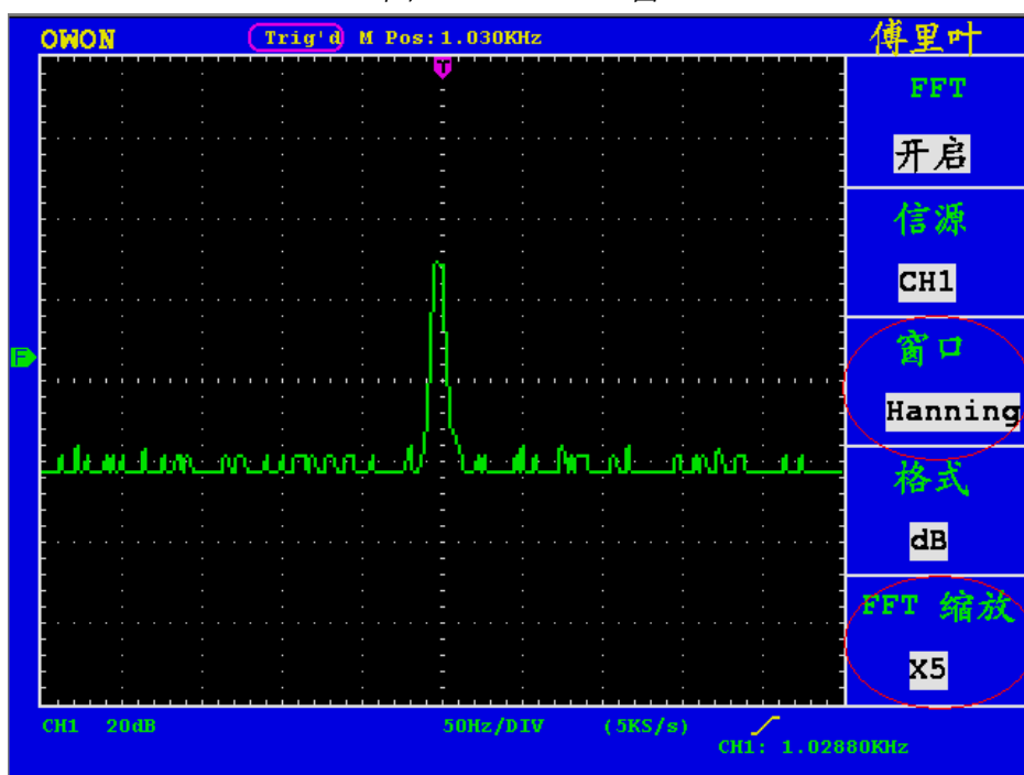
图22. Hanning窗
