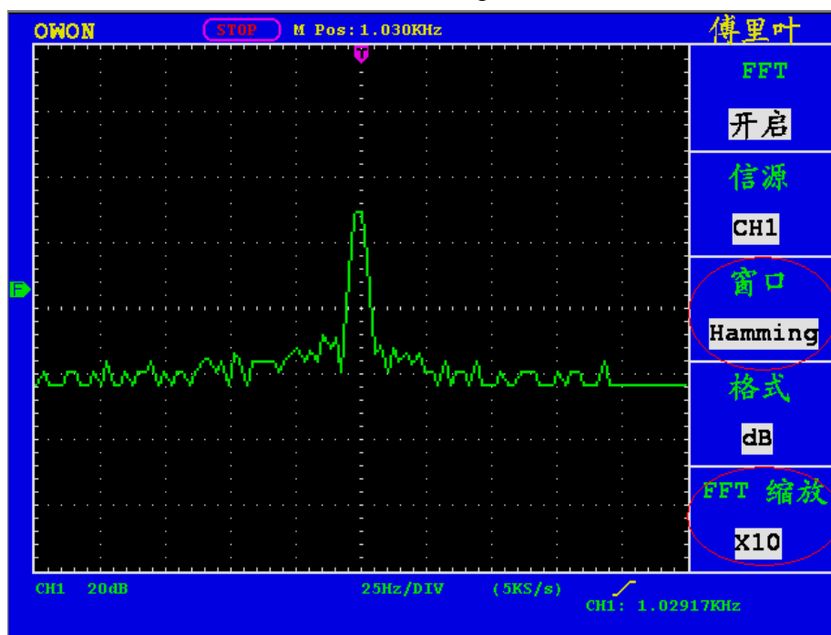
图24. Hamming窗
