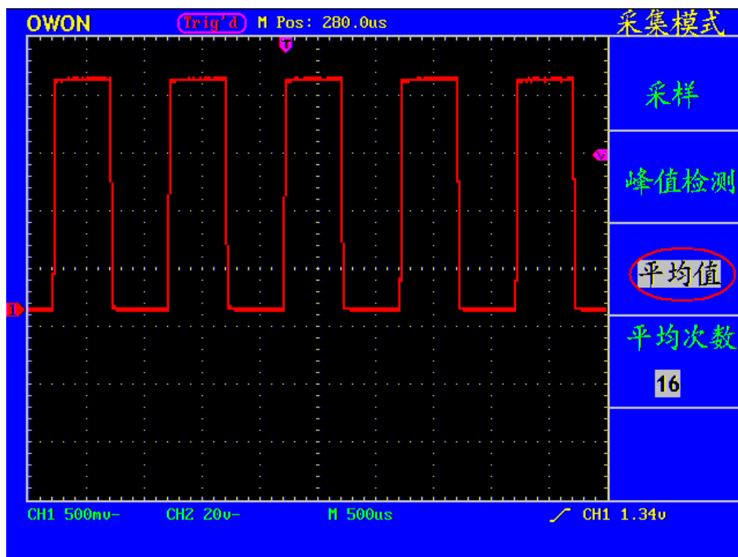
图 68: 去除噪声信号的波形
