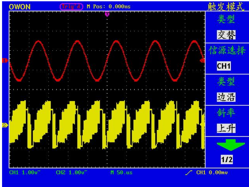
图42: 交替触发波形
