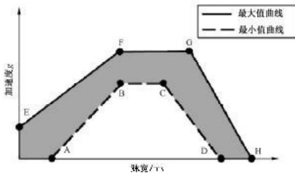
图 4 机械冲击脉冲容差范围示意图
