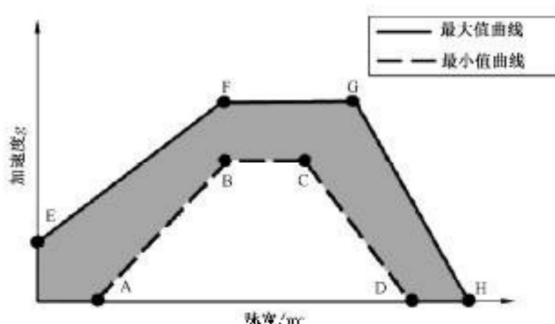
图5 模拟碰撞脉冲容差范围示意图
