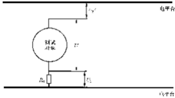
图 B.2 绝缘电阻测量步骤 2
