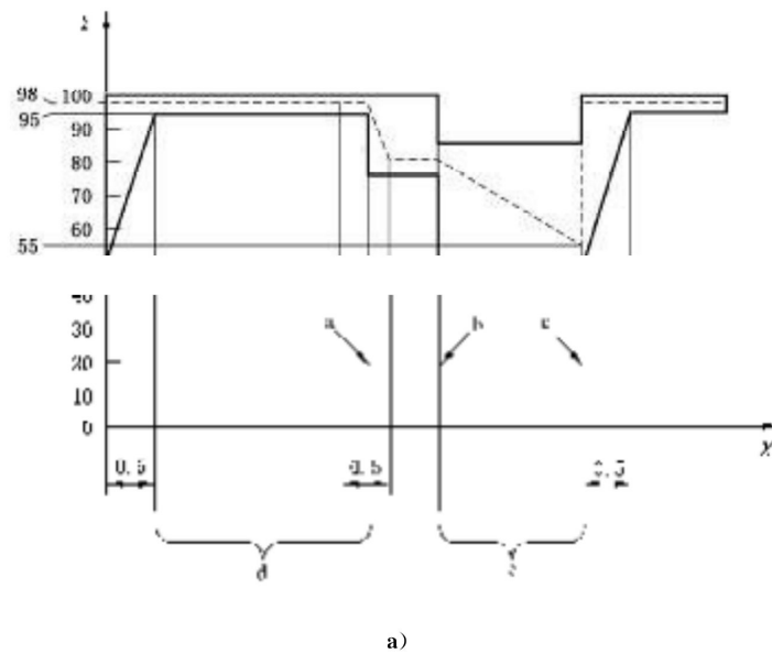
图 8 温湿度循环
