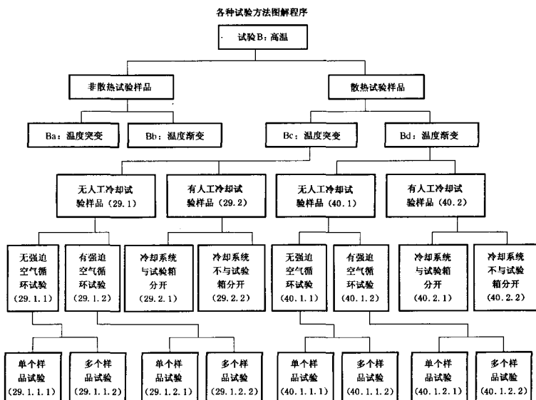
图 1 高温试验方法分类的方框图
