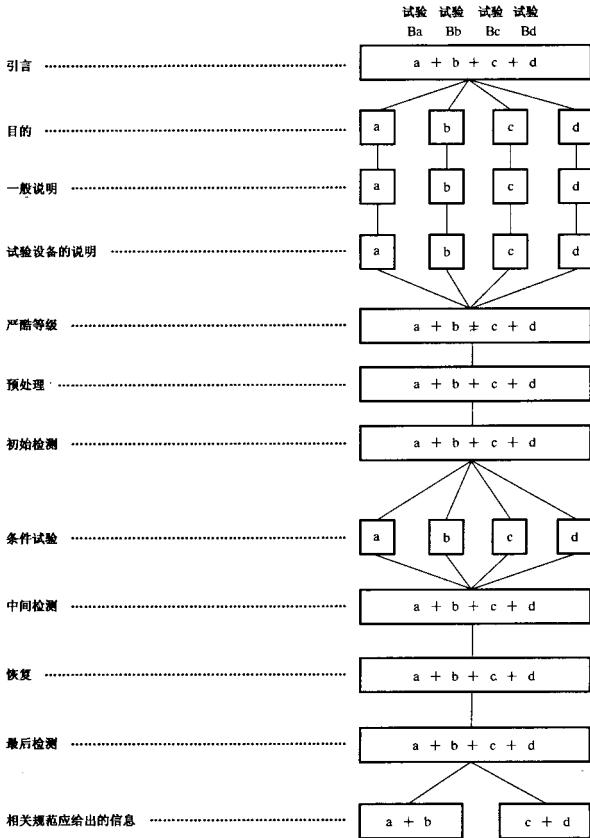
图 2 试验 B: 高温试验的方框图
