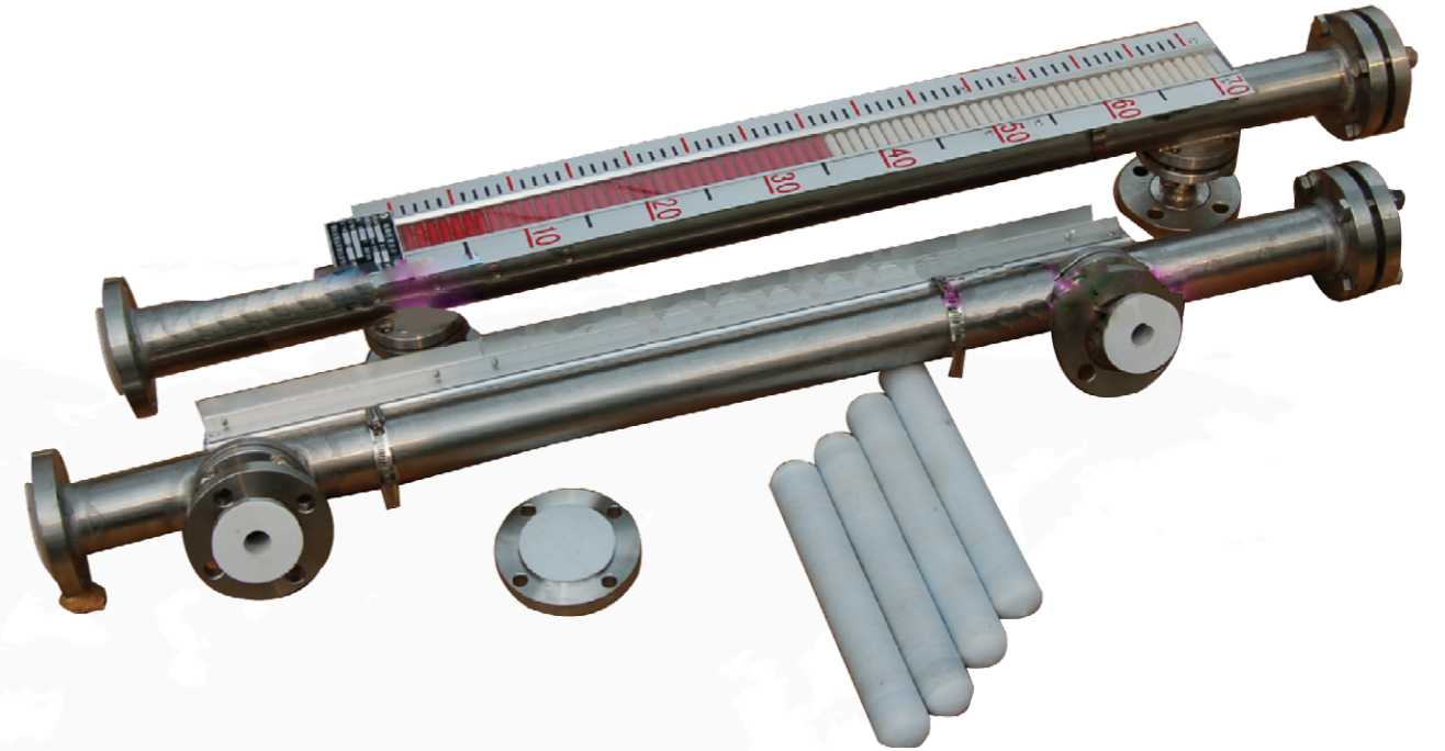
图一：侧装
