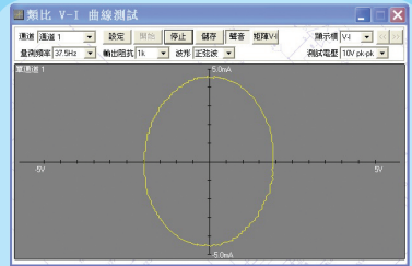
电容的V-I曲线图
