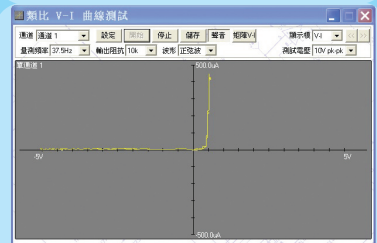
二极管的V-I曲线图
