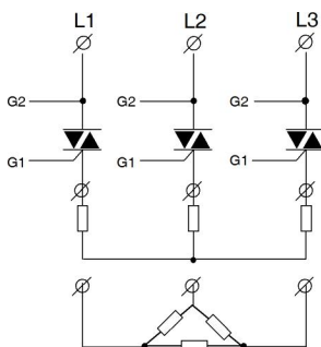
K3 三相三线星型、 三角形接线图（双向可控硅）
