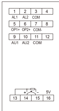
D71接线图
