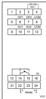
E7接线
