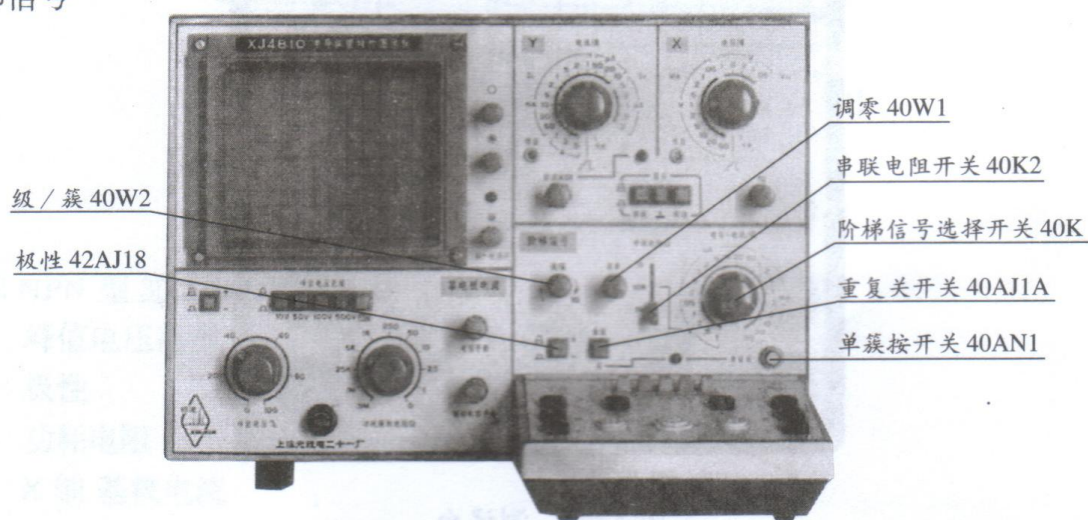
图 4—7 阶梯信号
