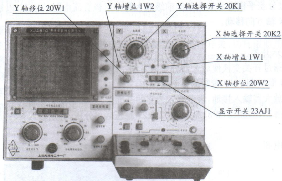
图 4-5 Y轴、X轴作用选择
