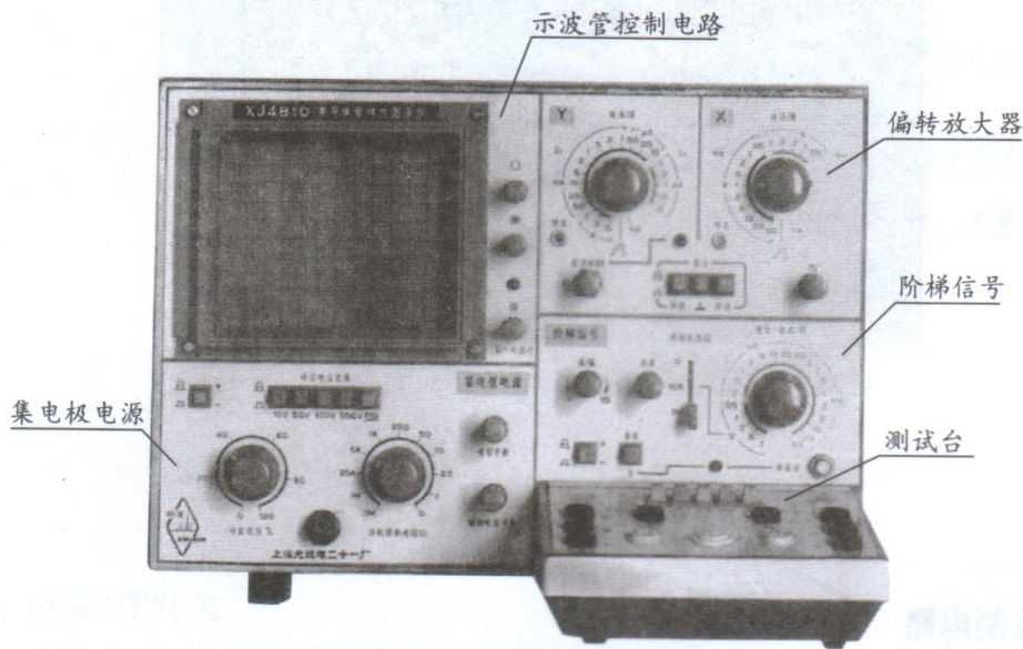
图 4-1 前面板单元划分图
