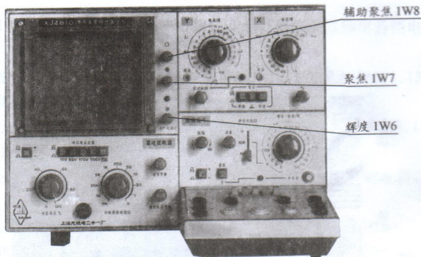
图 4-4 示波管及其控制电路
