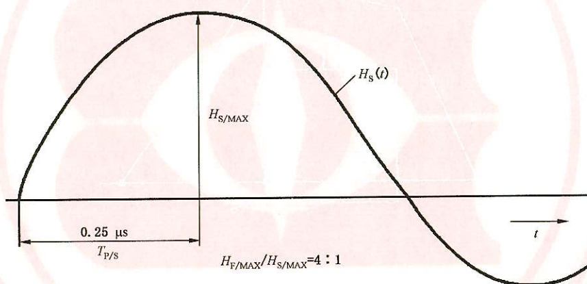
图 H.2 模拟首次正雷击(10/350 \mu s)的磁场上升沿
