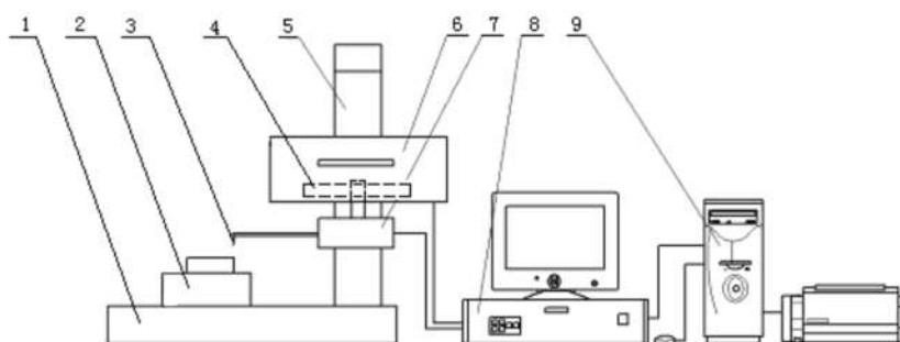
1—底座；2—工作台；3—触针；4—基准导轨；5—立柱； 6—驱动箱；7—传感器；8—电子信号处理装置；9—计算机系统。
