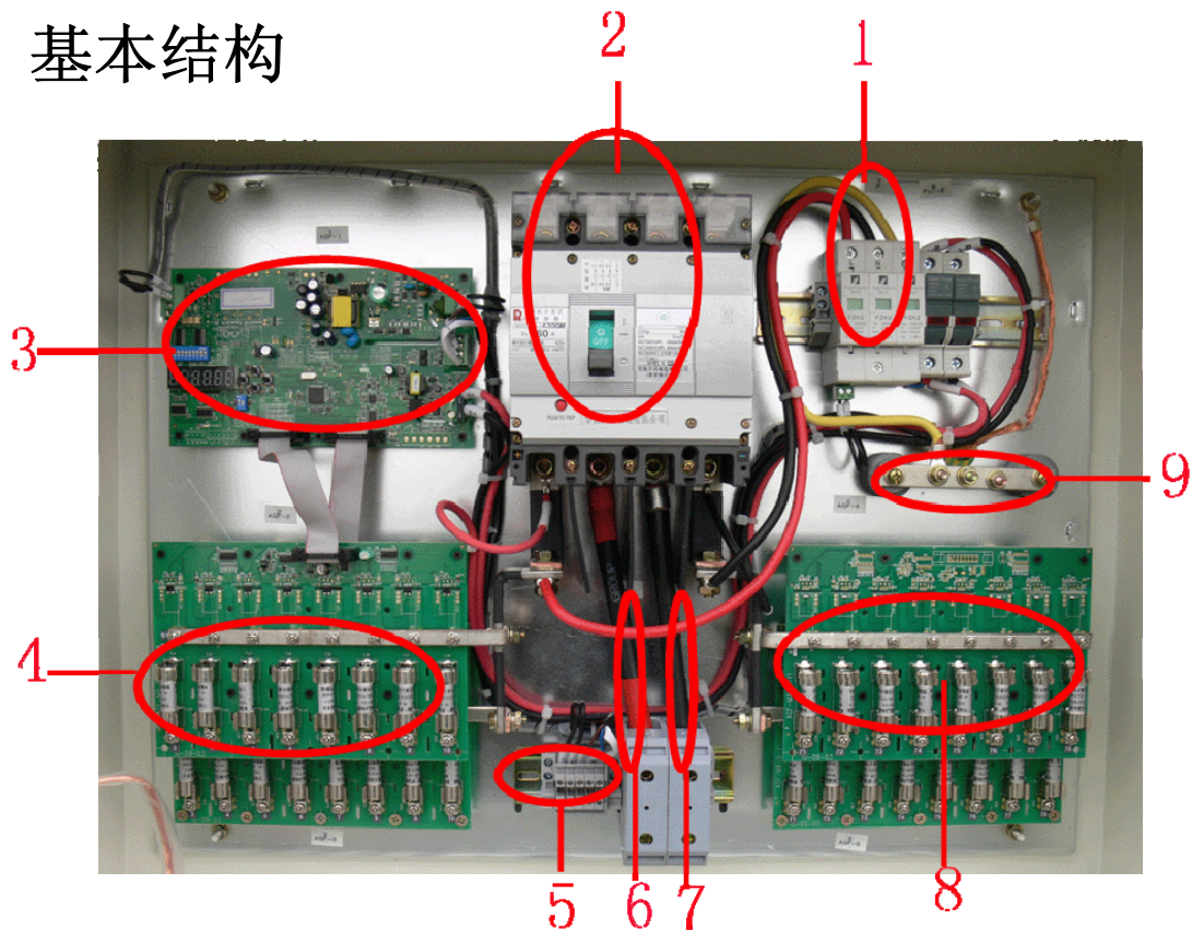
图 1 内部实物图(裸板式)
