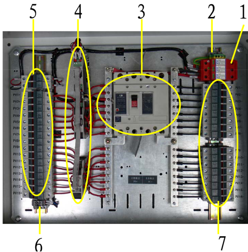
图 3 内部实物图(穿孔式)
