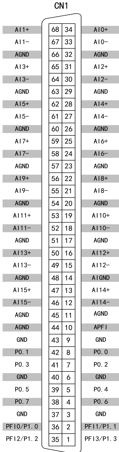
图 3-2-1 PCI9009\A/B 管脚定义图
