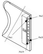
图 3-2-2 RTSI 的 Pinout 图
