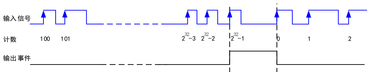
图 5-10-1 脉冲方式输出
