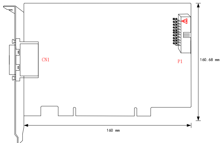
图 3-1-1 PCI9009\A\B 板卡尺寸图
