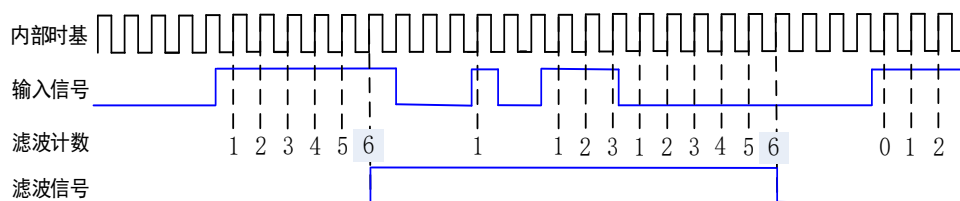
图 5-9-1 数字滤波示例
