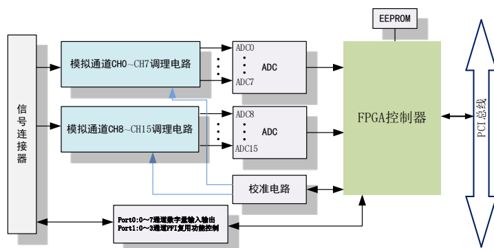
图2-2-1 PCI9009\A\B系统框图
