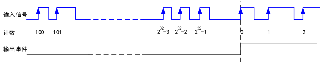
图 5-10-2 反转方式输出
