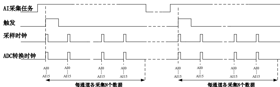
图 4-7-2 有限点采样
