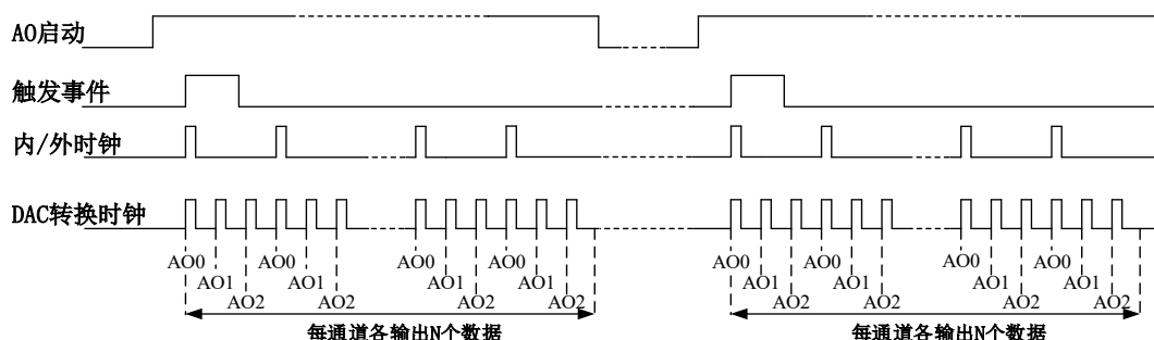
图4-6-2 内/外时钟有限点采样
