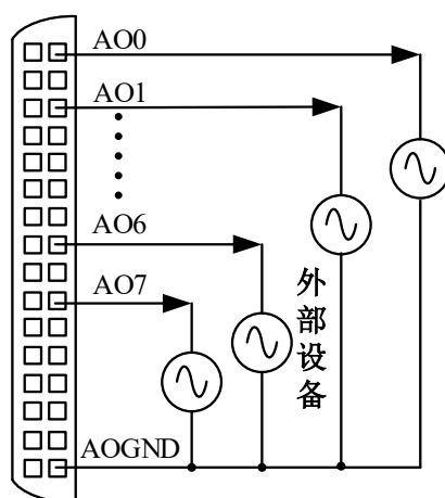
图4-2-1 DA模拟量输出连接
