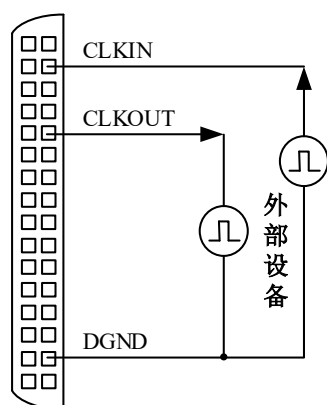
图 4-5-3 时钟输入输出的连接
