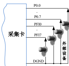
图6-2-1 DI 数字量输入的连接
