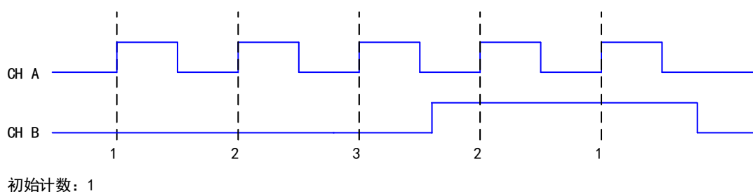
图 5-6-5 单脉冲编码
