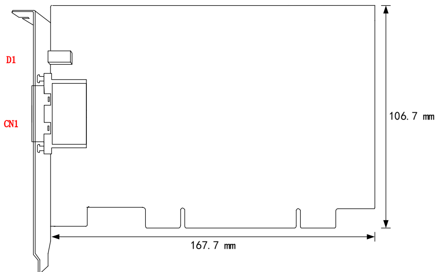
图 3-2-1 尺寸图
