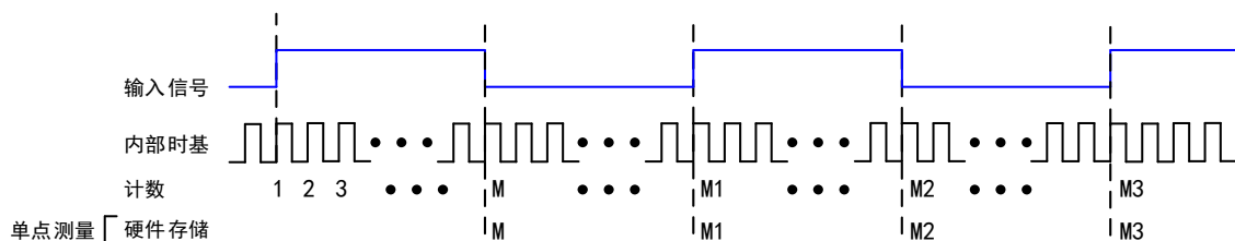
图 5-3-1 半周期示意图
