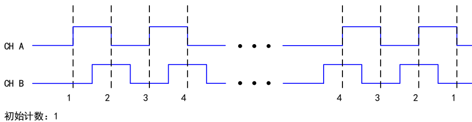
图 5-6-2 X2 编码
