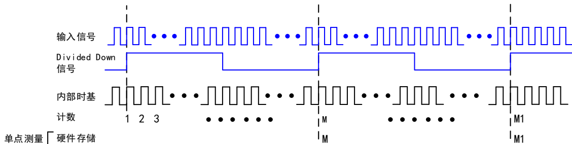
图 5-2-3 大范围信号频率测量上升沿有效示意图
