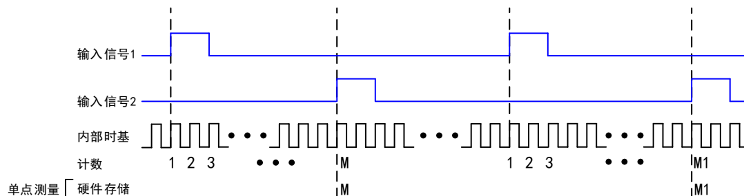
图 5-5-1 两边沿均上升沿有效示意图
