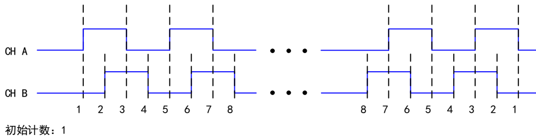
图 5-6-3 X4 编码
