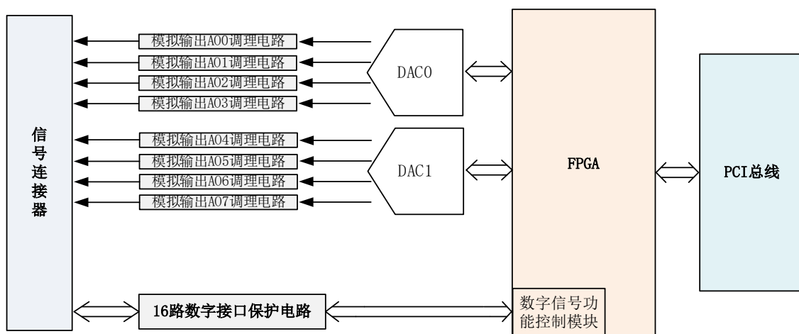
图 2-2-1 PCI9312 系统框图
