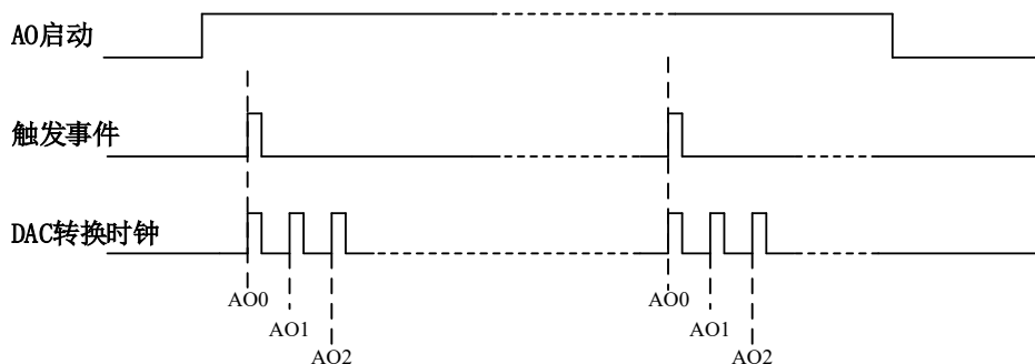
图4-6-1 按需单点采集
