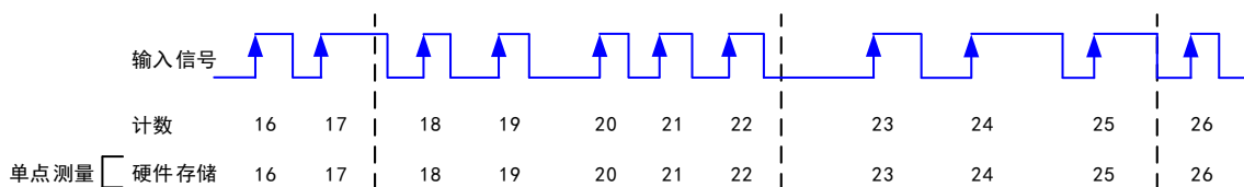
图 5-1-1 边沿加计数上升沿有效示意图
