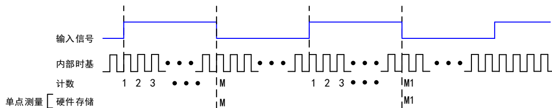
图 5-4-1 脉宽测量上升沿有效示意图
