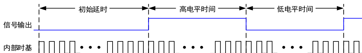
图 5-7-1 脉冲输出方式为时间输出
