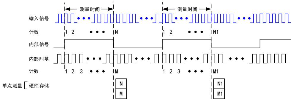
图 5-2-2 高频信号频率测量上升沿有效示意图
