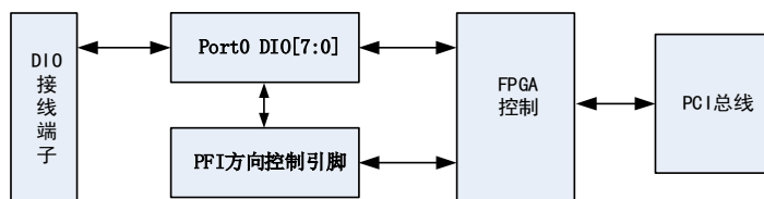
图6-1-1 DIO功能框图
