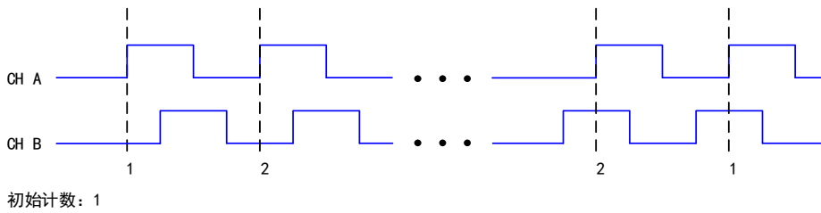
图 5-6-1 X1 编码
