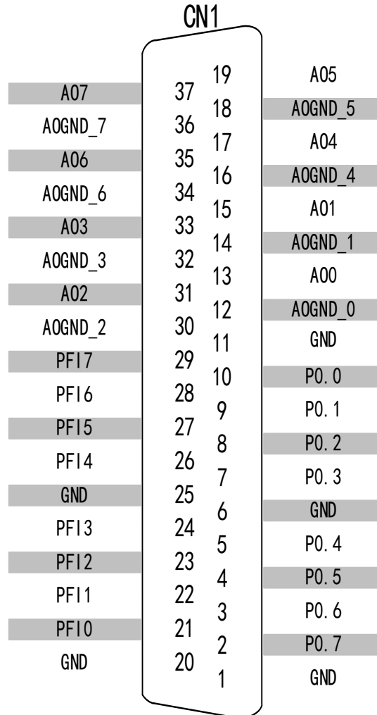
图 3-3-2 连接器引脚定义
