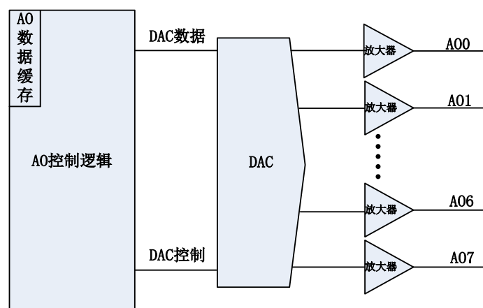
图 4-1-1 DA 功能框图
