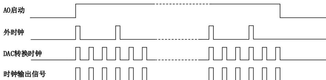
图 4-5-2 外时钟时序图
