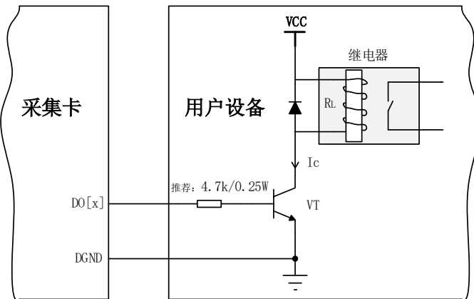
图 6-3-1 DO 数字量控制继电器电路
