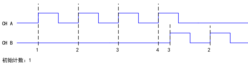
图 5-6-4 双脉冲编码
