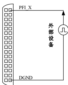
图 4-7-1 触发信号连接
