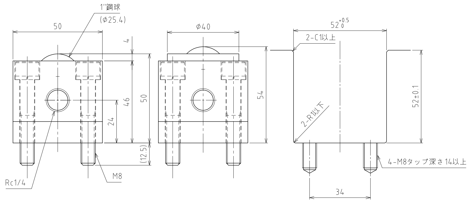
A矢視図
