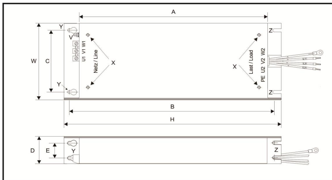
附图 3 EMC 滤波器外形尺寸
