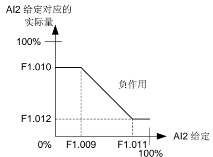
图 5-9 模拟输入 AI2 给定反作用特性
