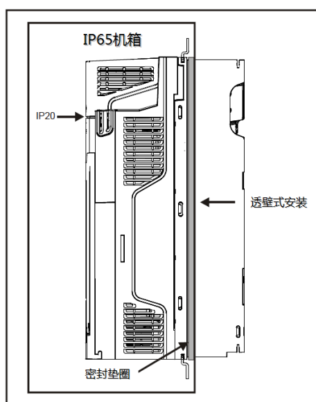
图 3-14 IP65 等级的柜内安装图
