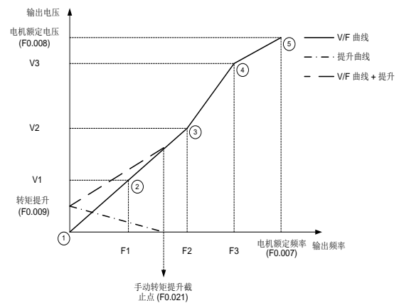
图 5-3 自定义 V/F 曲线
