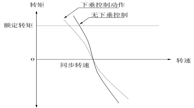
图 5-53 下垂控制电机特性
