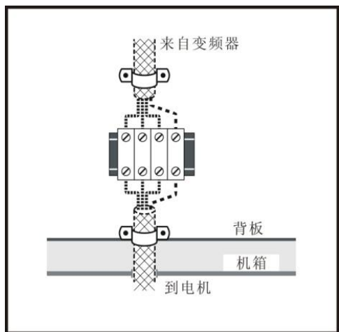
图 3-45 将电机线缆连至柜内接线端子
