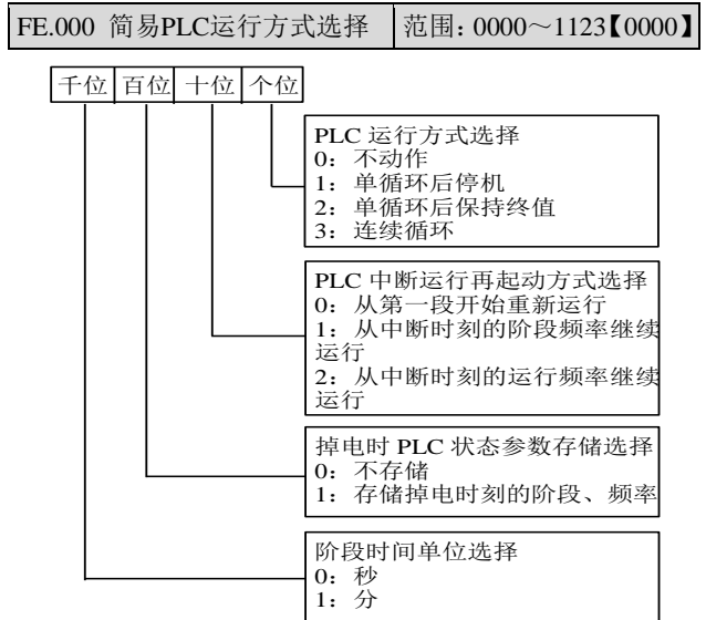
图 5-57 简易 PLC 运行方式选择
