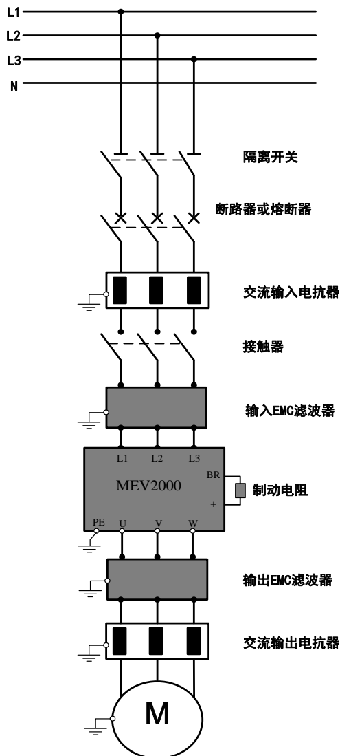
图 3-19 变频器与选配件的连接
