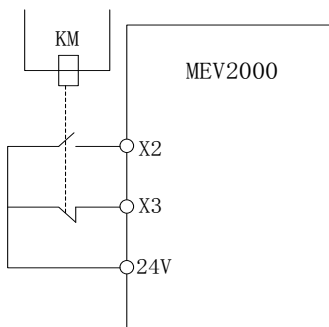
图 5-36 外部设备故障常开/常闭输入示意图
