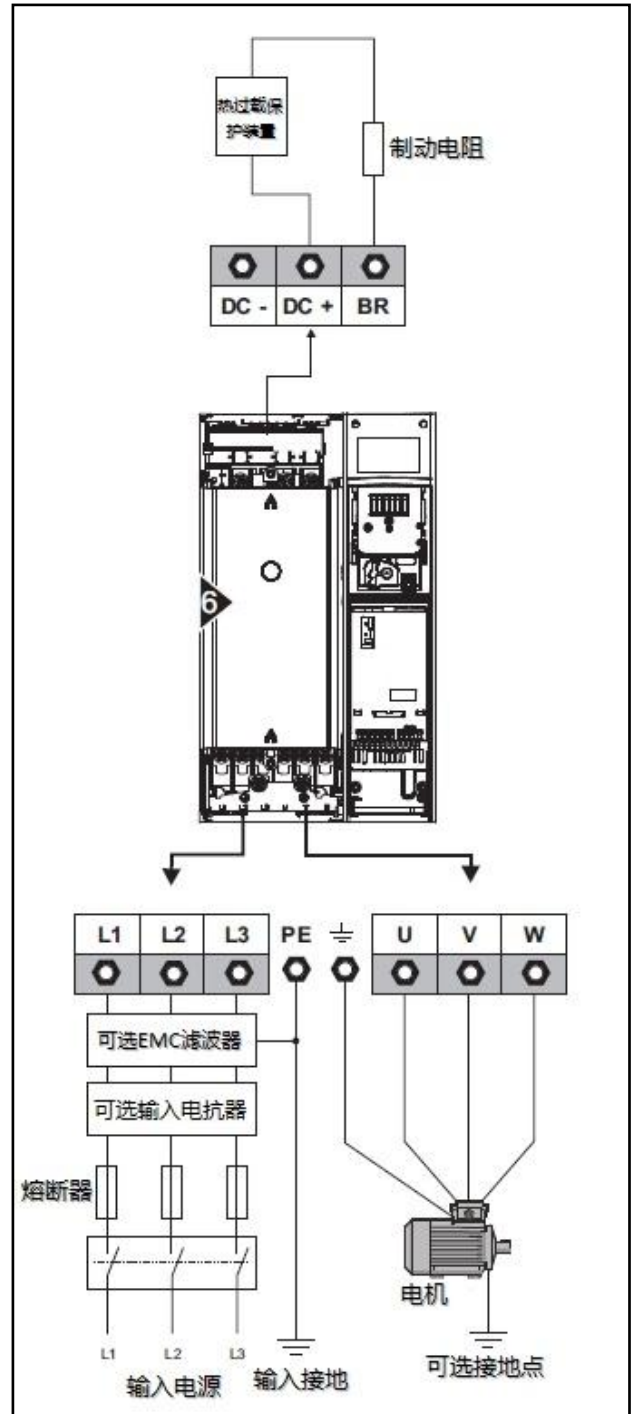
图 3-24 Size6 主回路输入输出连接图
