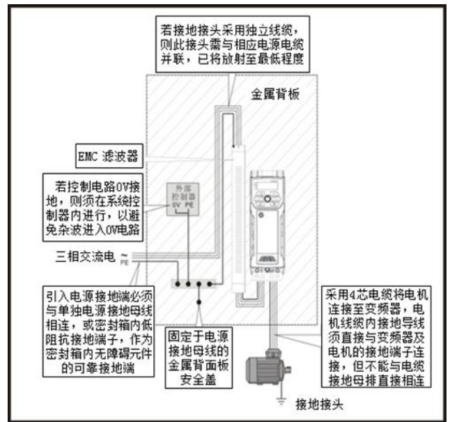
图 3-36 一般 EMC 机壳所示接地连接
