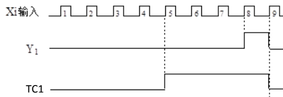
图 5-44 设定计数值给定和指定计数值给定示意图
