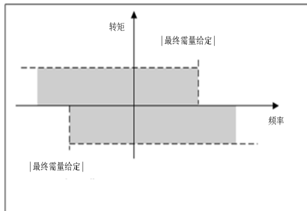
图 5-21 带频率限幅的双向转矩控制
