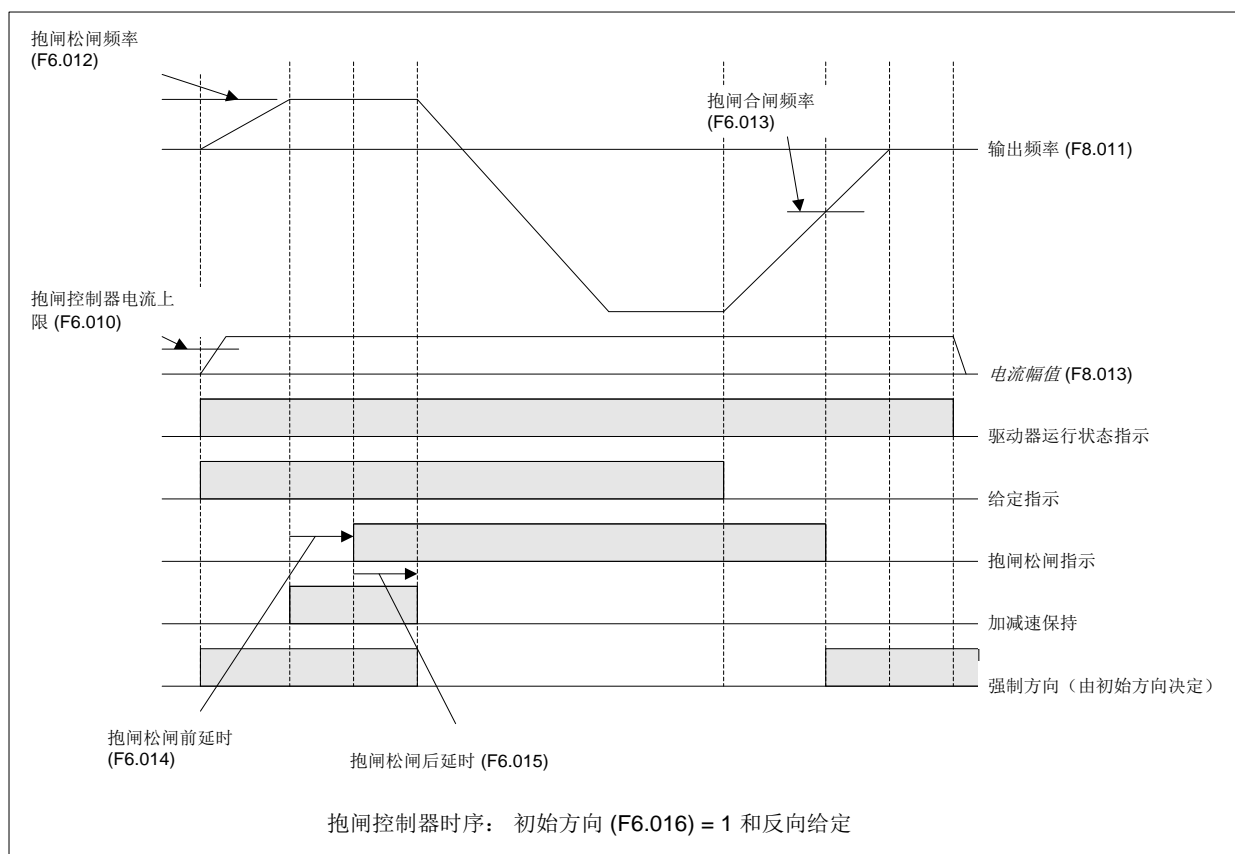
图 5-33 报闸控制器时序：初始方向 (F6.016) =1 和给定方向
