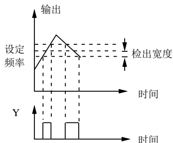
图 5-42 频率到达信号输出示意图
