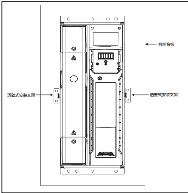
图 3-16 透壁式安装示意图
