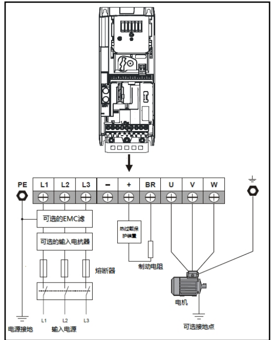
图 3-21 Size3 主回路输入输出连接图
