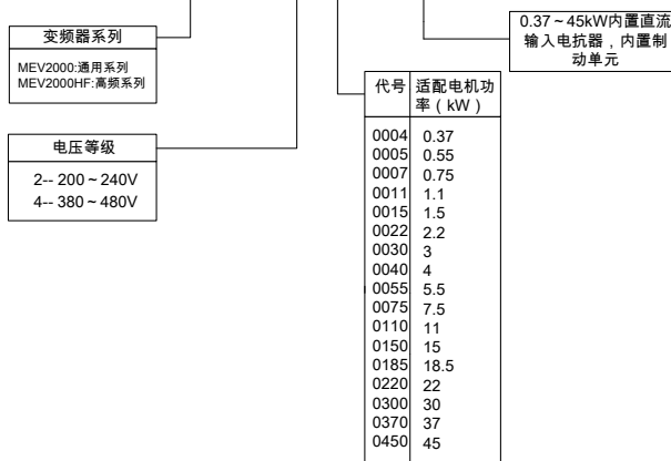
图 A-1 变频器型号说明
