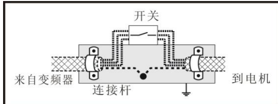
图 3-46 连接机电缆至隔离开关
