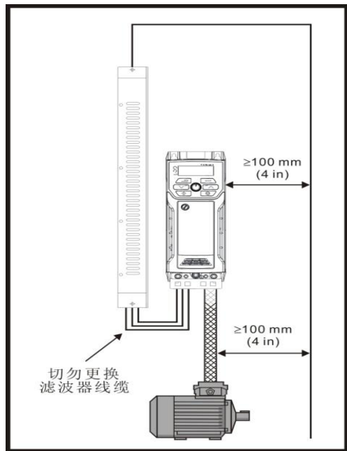
图 3-38 电源及接地线缆间距（Size2-6）
