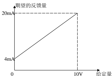
图 5-25 给定量和期望反馈量
