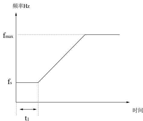
图 5-10 起动频率与起动时间示意图
