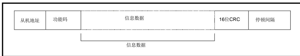
附图 5 帧格式
