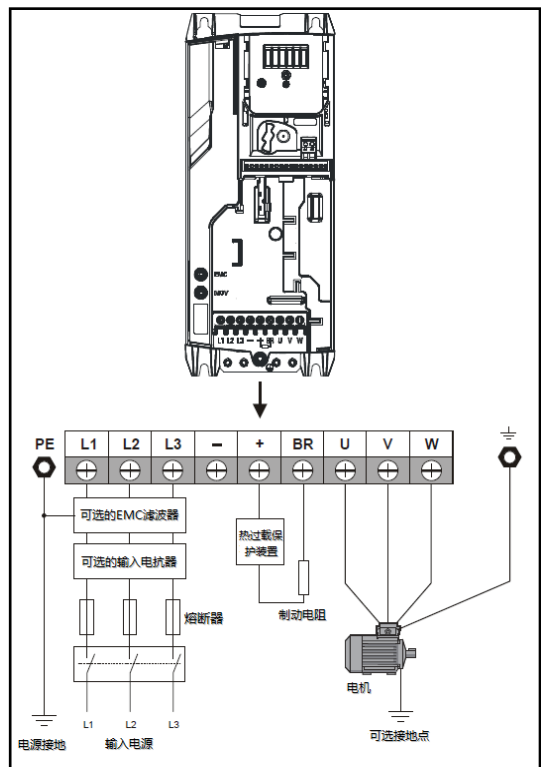
图 3-22 Size4 主回路输入输出连接图
