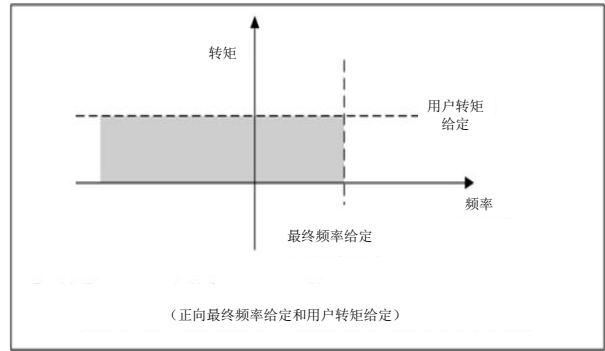
图5-17 带频率限幅的速度控制
