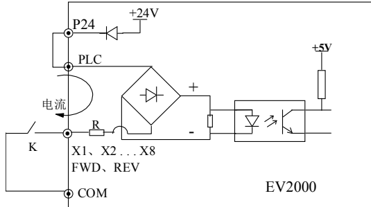
图3-22 使用内部24V电源的接线方式
