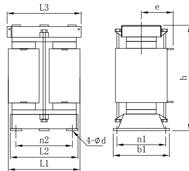
附图5 直流电抗器外形图b
