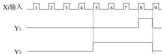
图5-50 设定计数值给定和指定计数值给定示意图
