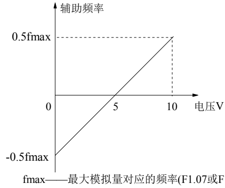
图5-61 VCI-5或CCI-5作为辅助频率给定通道
