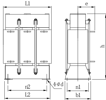
附图2 三相交流输入、输出电抗器外形图b
