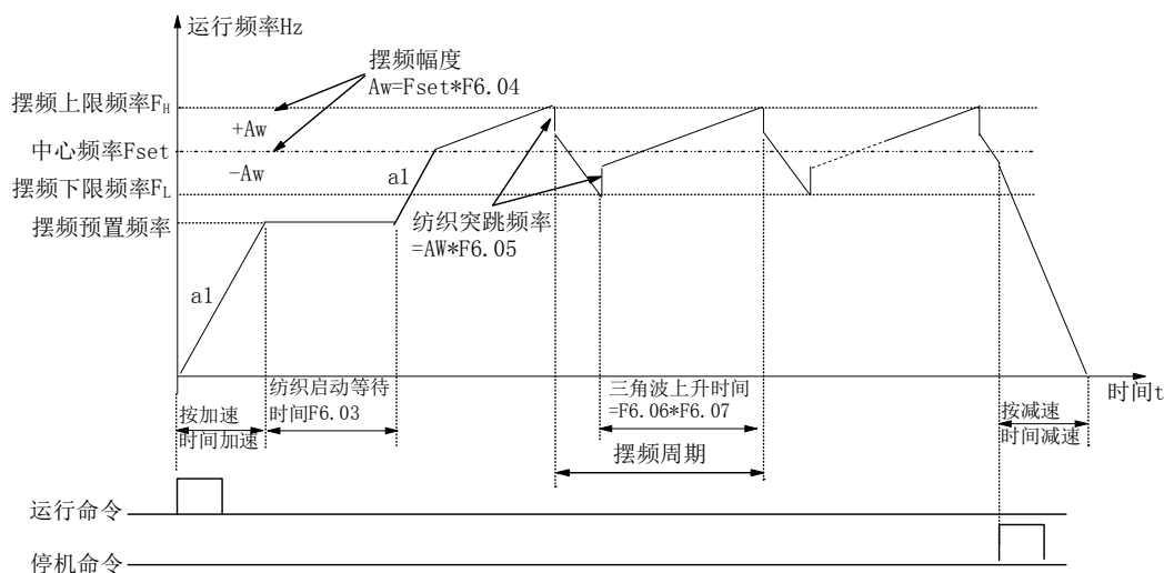
图5-37 摆频示意图
