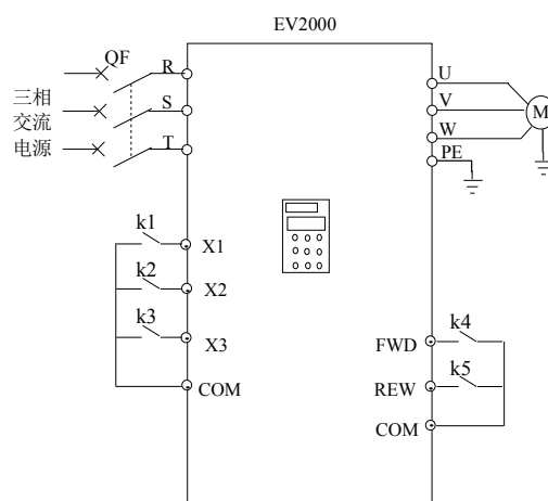
图5-40 多段速度运行接线图
