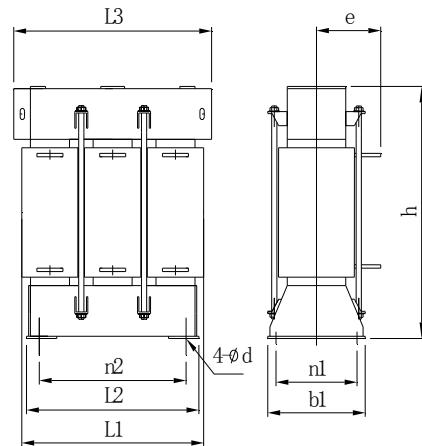
附图3 三相交流输入、输出电抗器外形图c
