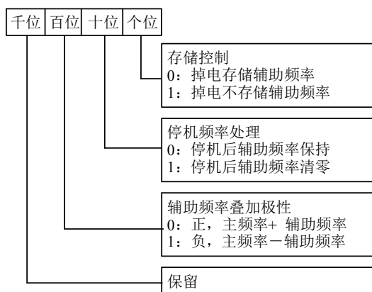
图5-63 数字辅助频率控制设定
