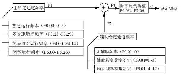
图5-59 给定频率合成示意图
