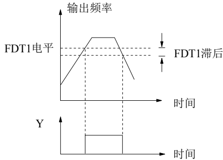
图5-48 频率水平检测示意图
