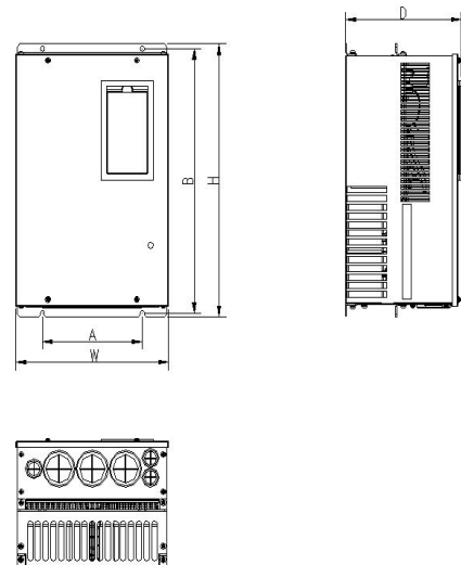
图b EV2000-4T0185G1/0220P1~
