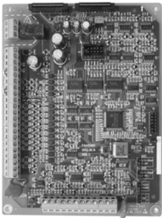
图3-13 控制板照片
