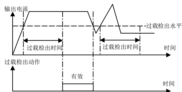
图5-74 过载预警检出功能示意图
