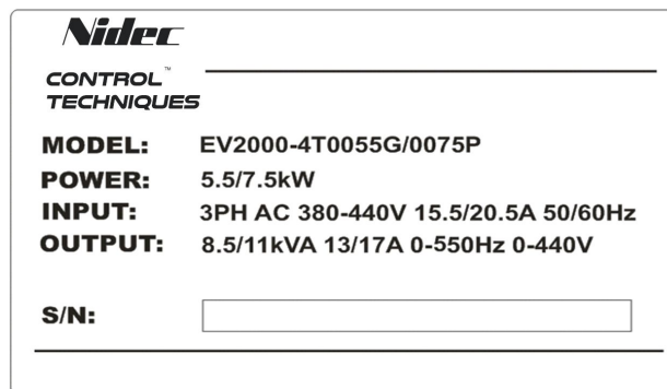
图A-2 变频器铭牌
