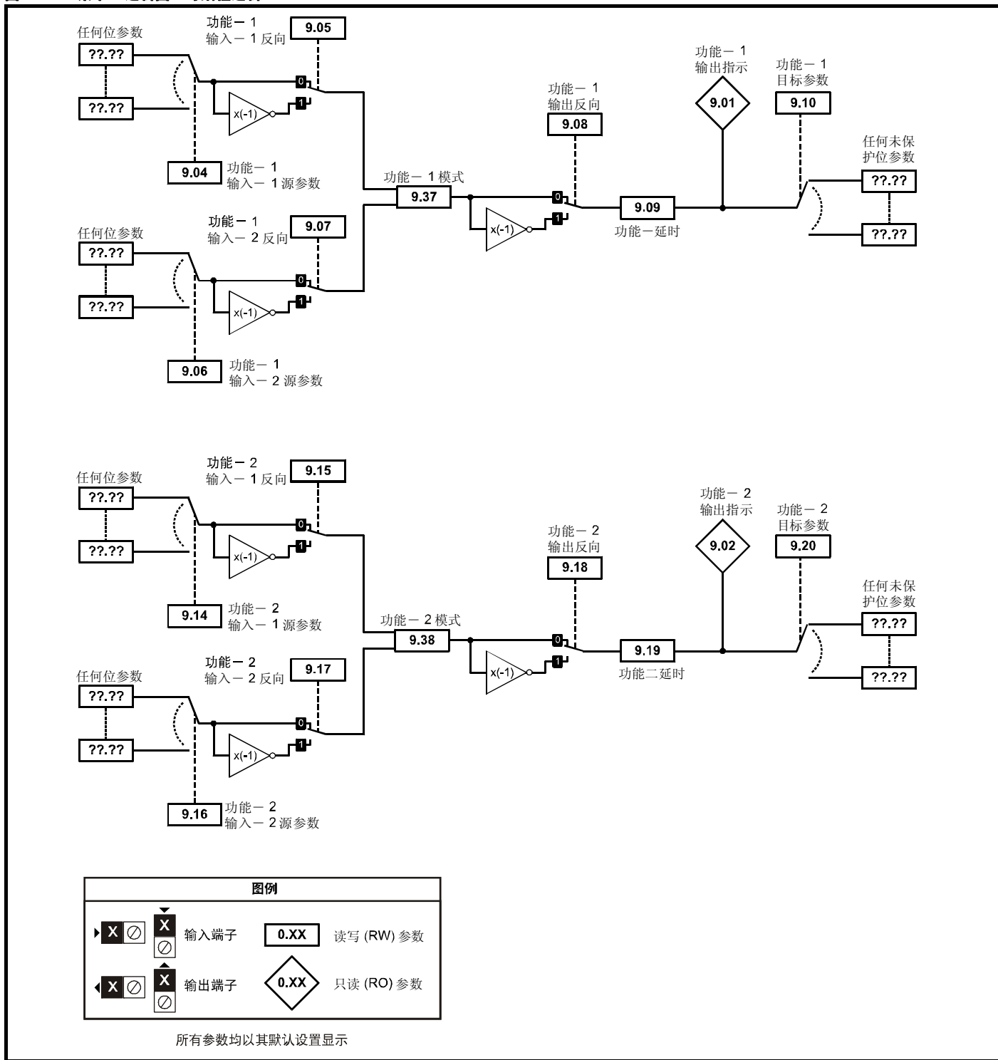
图 11-12 菜单 9 逻辑图: 可编程逻辑
