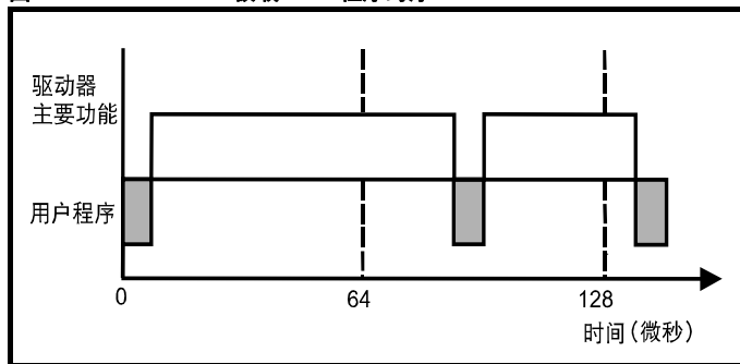
图 10-1 Mentor MP 板载 PLC 程序时序
