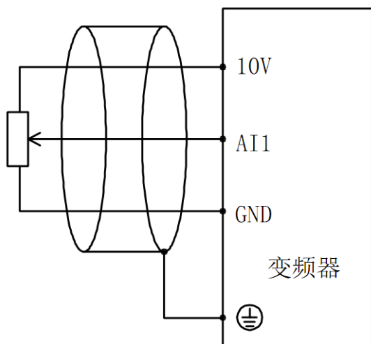
图 3-14 模拟量输入的连接方式
