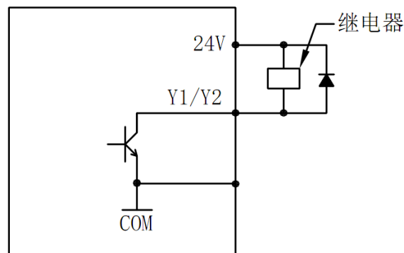
图 3-12 内部 24V 电源连接方式
