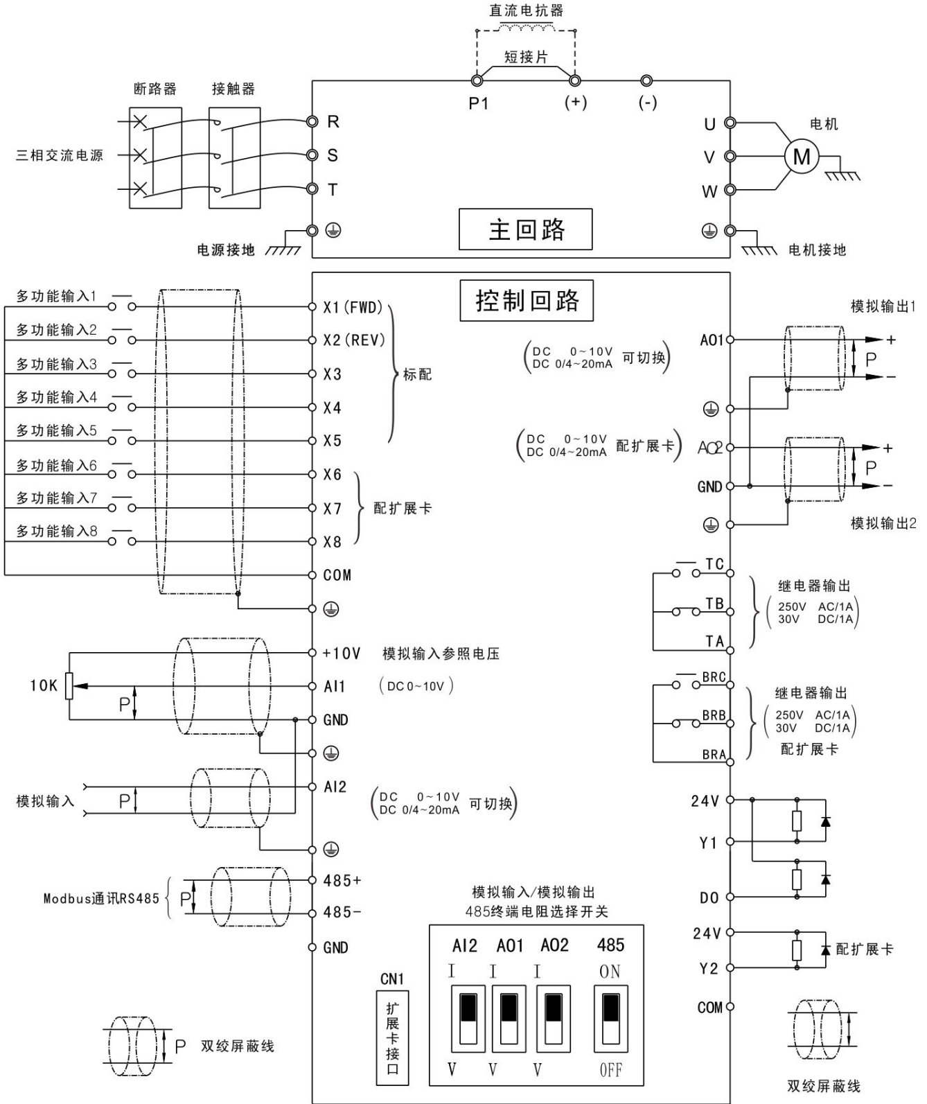
图 3-8 端子配线图 (以 NE300-4T0300G/0370P 及以上型举例)
