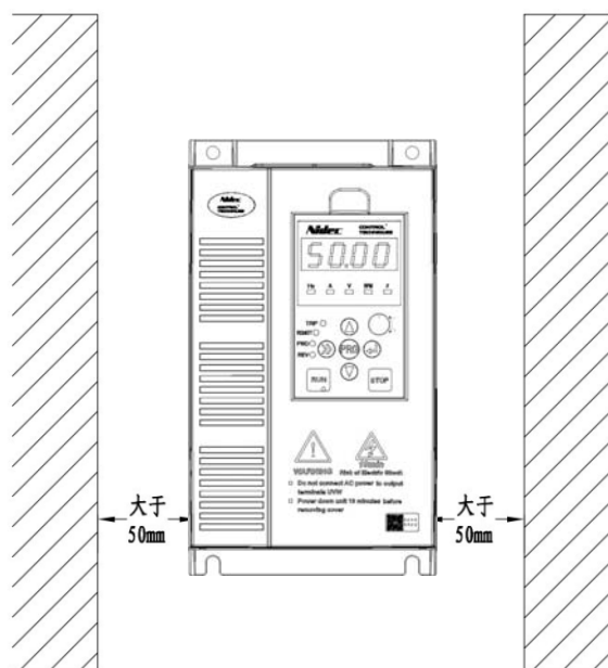
图 2-1 NE300 安装方向和空间
