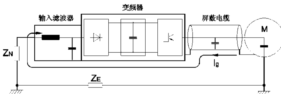
图 3-6 传导和辐射干扰的对策
