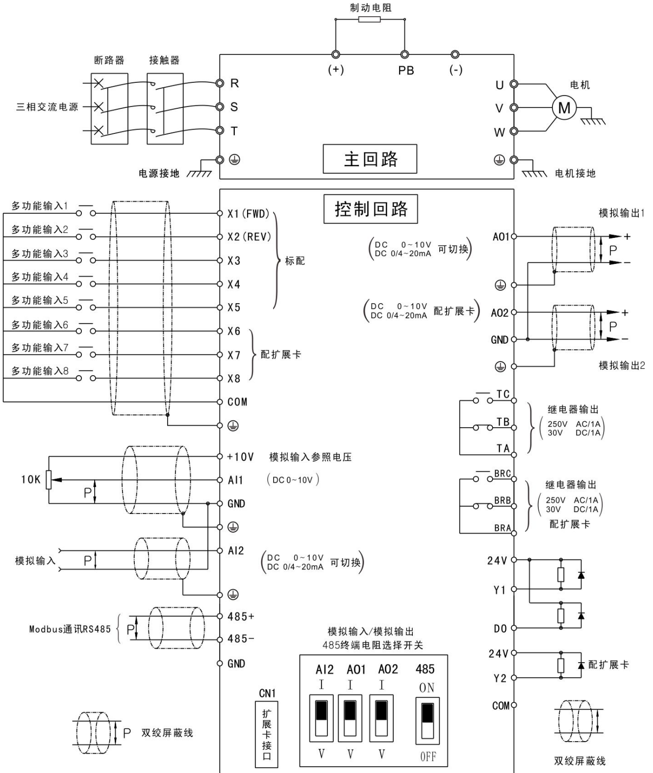
图 3-7 端子配线图 (以 NE300-4T0220G/0300PB 及以下型举例)
