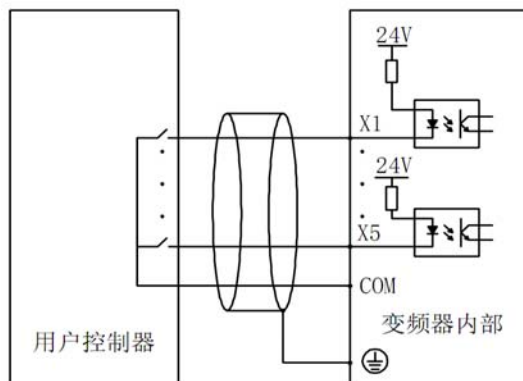
图 3-10 控制回路端子接线说明
