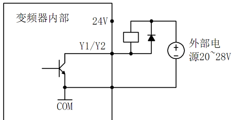
图 3-13 外部电源连接方式
