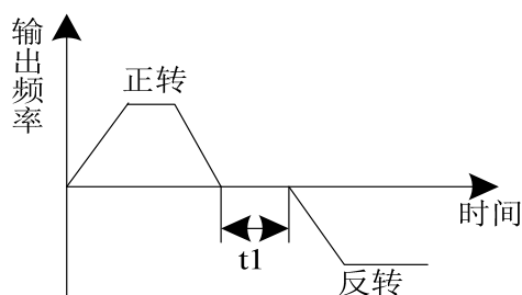
图6-6 正反转切换
