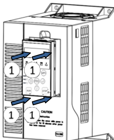
图 2-4 操作面板的安装
