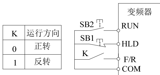
图6-16 三线式2
