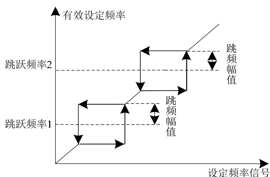
图6-5 跳跃频率
