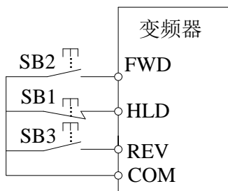
图6-15 三线式1
