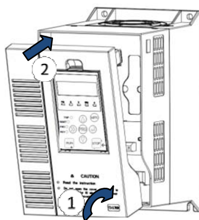
图 2-6 上盖板的拆卸
