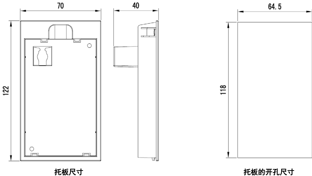
图 1-5 托板的外形和安装尺寸
