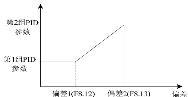
图 6-23 PID 参数自动切换
