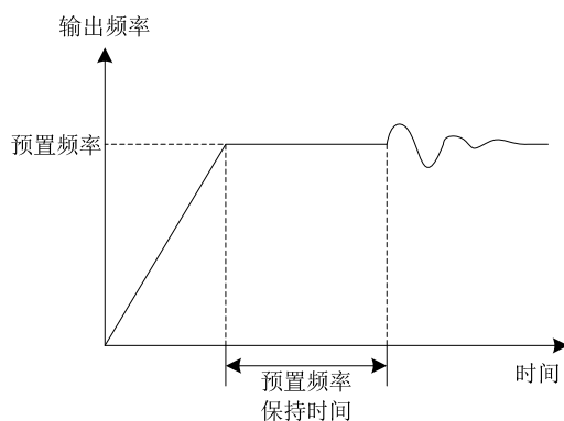
图 6-24 预置频率保持示意图
