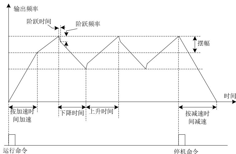
图6-26 摆频运行示意图
