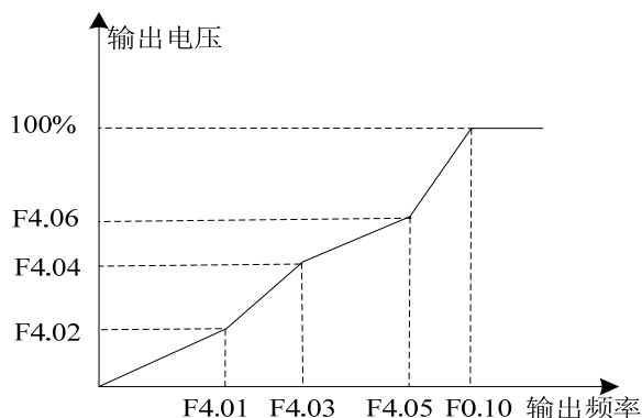
图 6-9 多点 V/F 曲线
