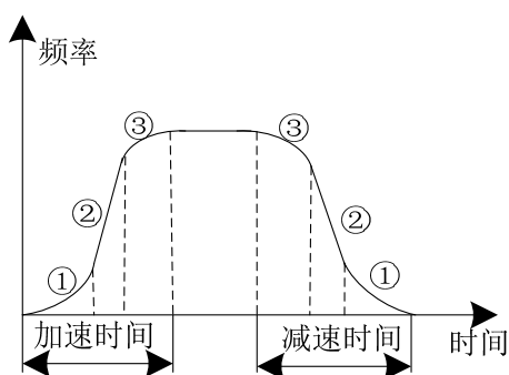
图6-4 S曲线加减速
