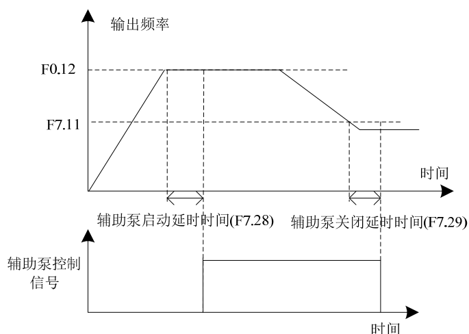
图6-22 恒压供水辅助泵控制信号
