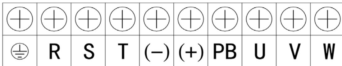
图 3-2 三相 400V 输入 0015G/0022PB~0220G/0300PB 主回路接线端子
