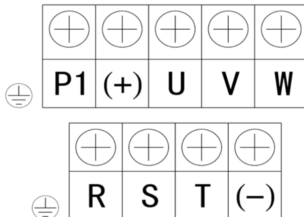
图 3-4 三相 400V 输入 1600G/2000P~8000G/9000P-F 主回路接线端子
