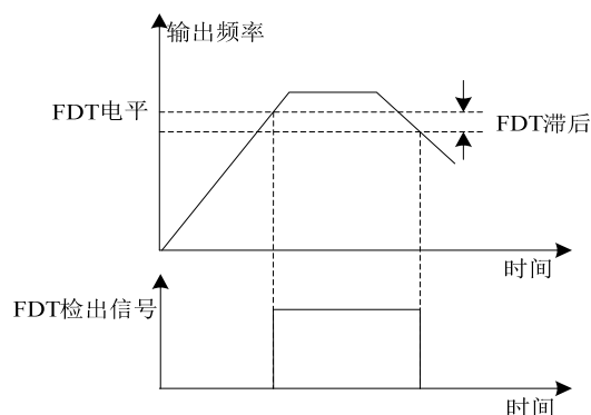
图6-21 FDT电平示意图
