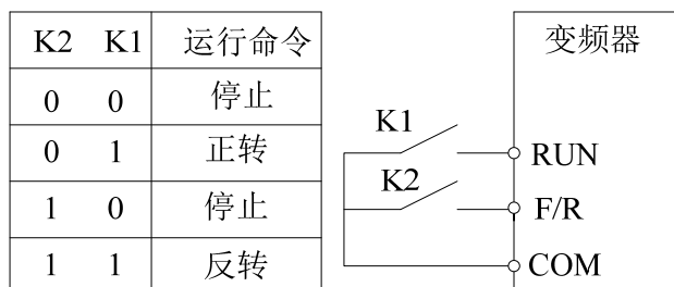
图 6-14 两线式 2
