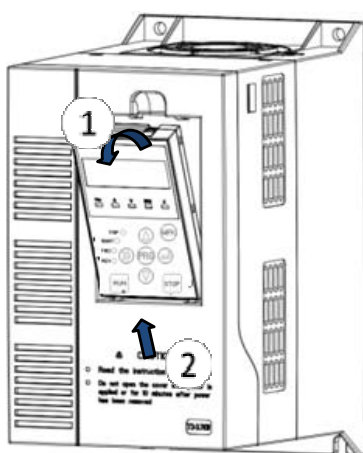
图 2-3 操作面板的拆卸
