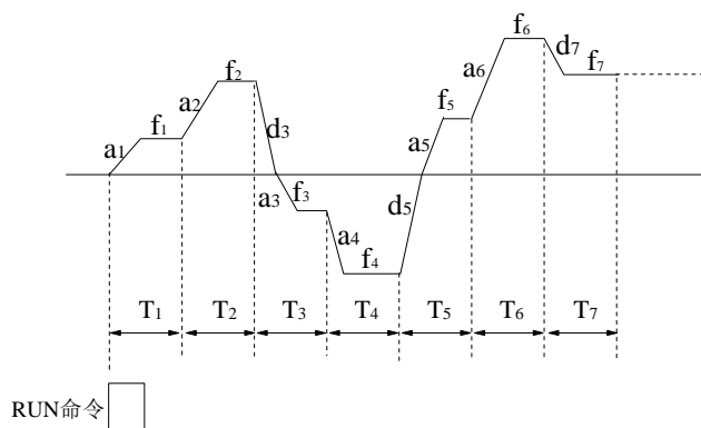
图 6-25 PLC 运行示意图
