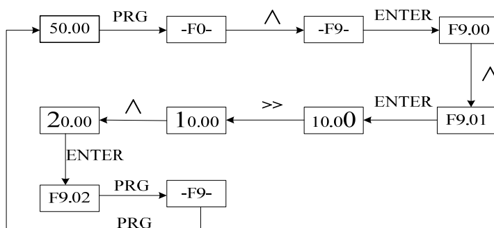
图 4-2 三级菜单操作流程图
