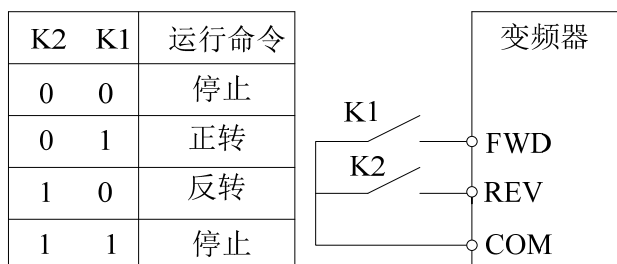
图 6-13 两线式 1
