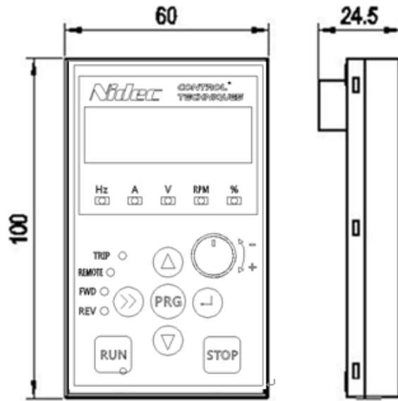
图 1-4 大、小操作面板的外形和安装尺寸（单位：mm）
