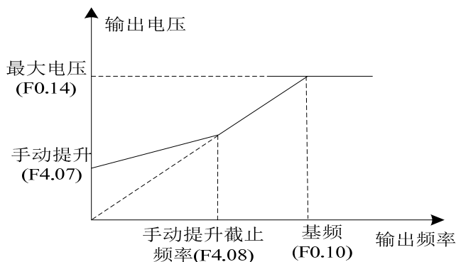
图6-10 转矩提升
