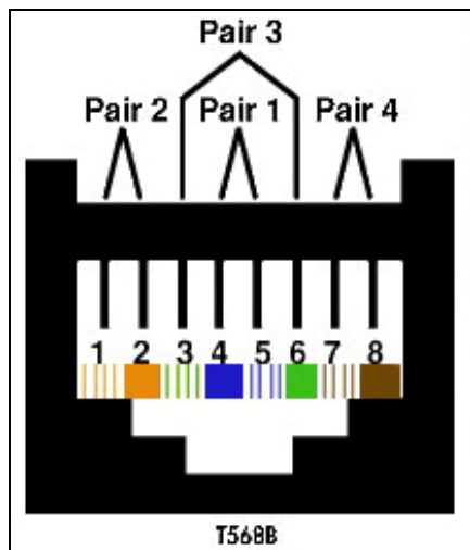
图 3-15 T568B 标准
