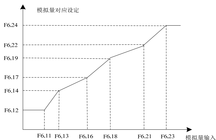
图 6-17 模拟输入非线性曲线
