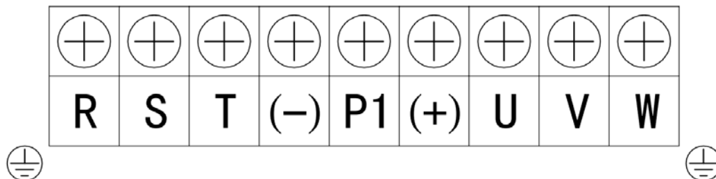
图 3-3 三相 400V 输入 0300G/0370P~1100G/1320P 主回路接线端子
