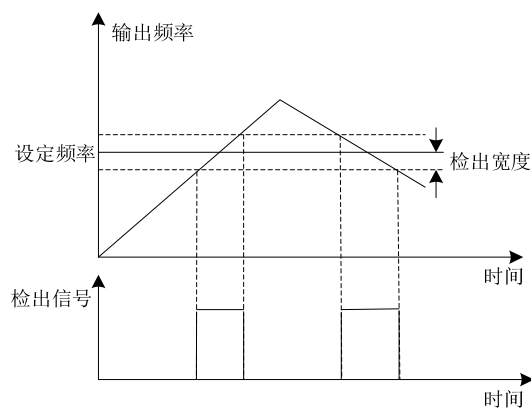
图 6-20 频率到达检出宽度示意图
