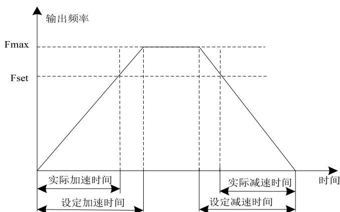
图6-2 加减速时间示意图
