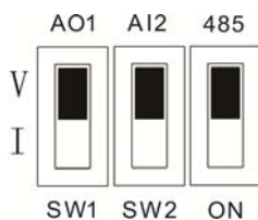
图 3-17 跳线功能说明
