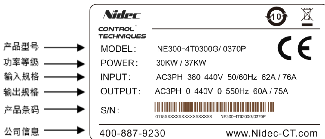
图 1-2 产品铭牌说明
