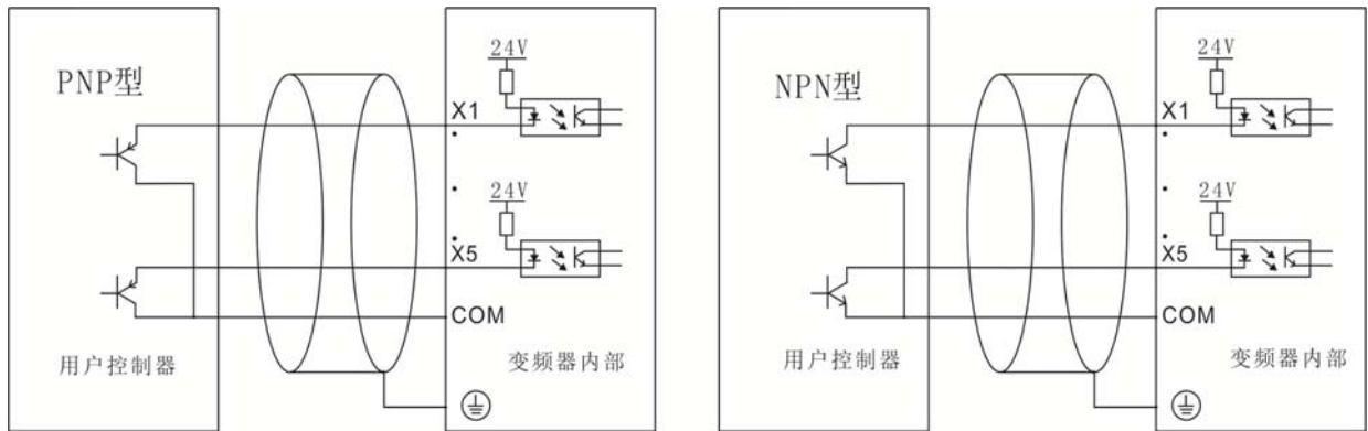
图 3-11 NPN、PNP 型共发射极连接方式
