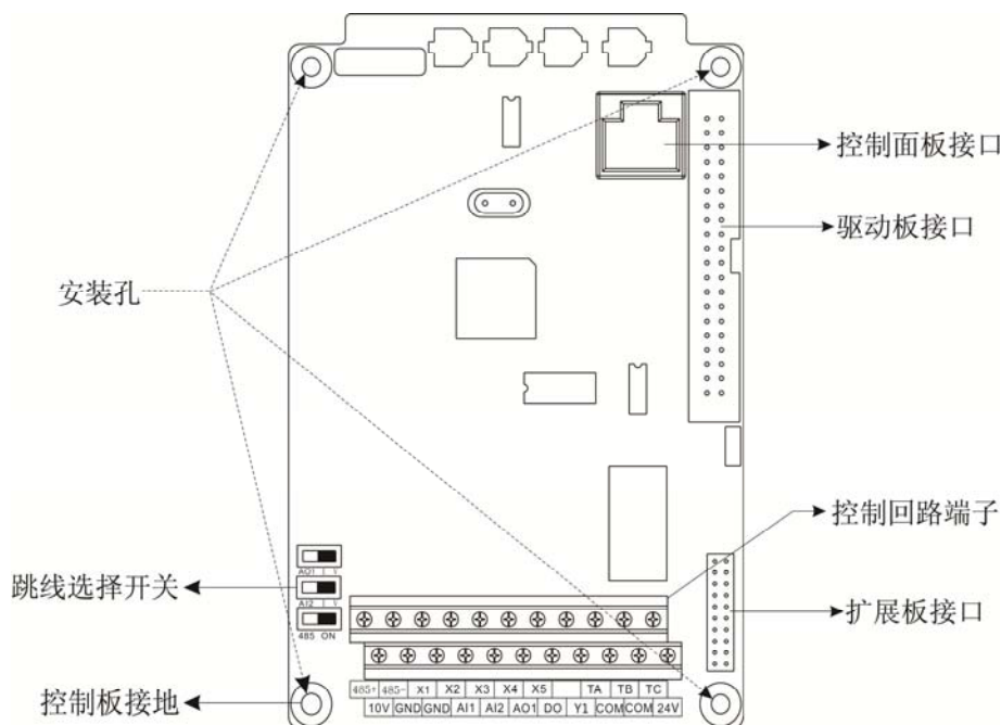
图 3-16 控制板示意图
