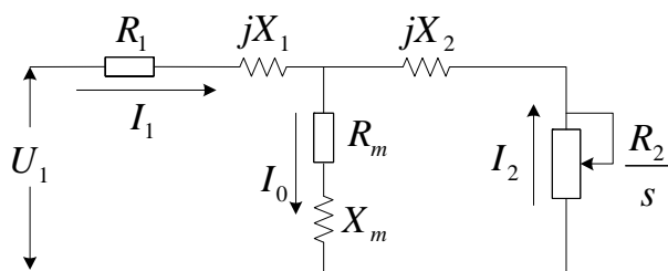
图6-12 异步电机稳态等效电路图
