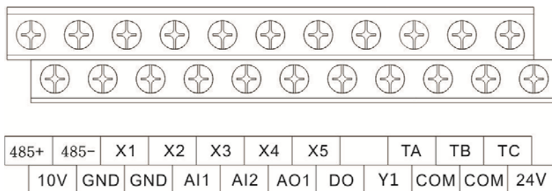
图 3-9 标配控制回路端子排列顺序
