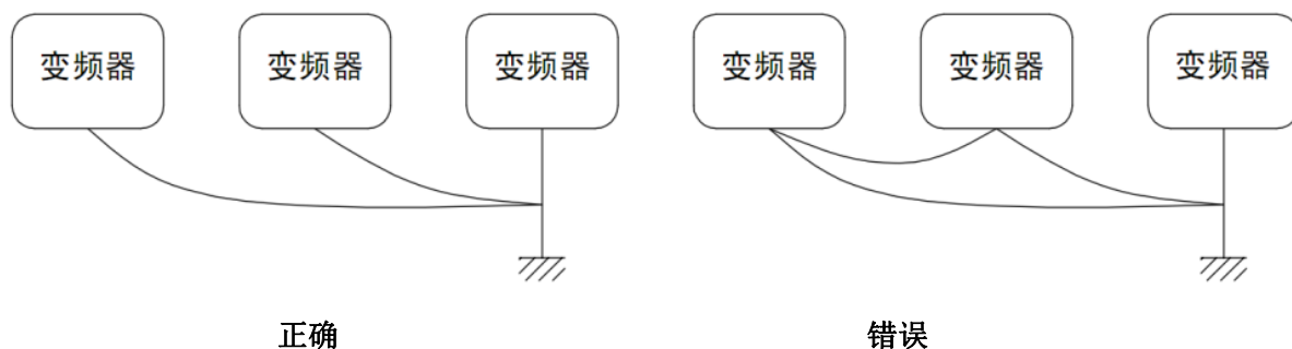
图 3-5 接地线配线
