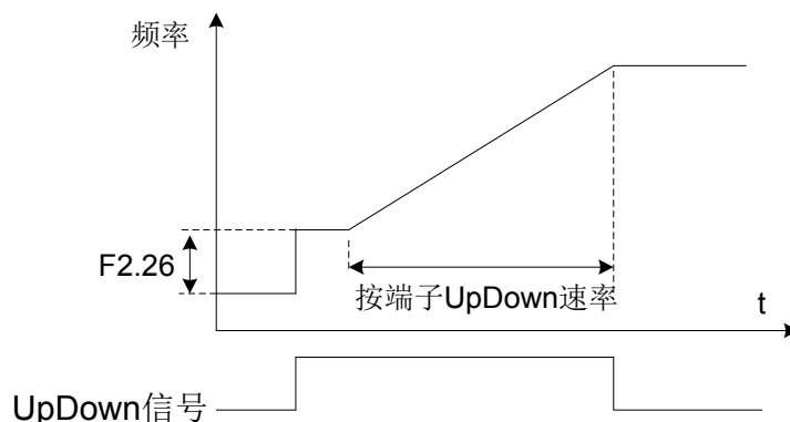
图6-19端子UpDown初始增量
