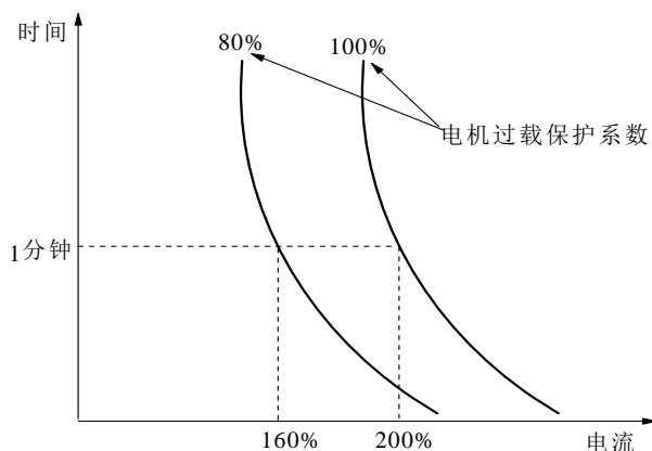
图6-27 电机过载保护系数设定
