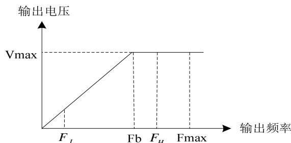
图6-1 输出频率与输出电压关系图
