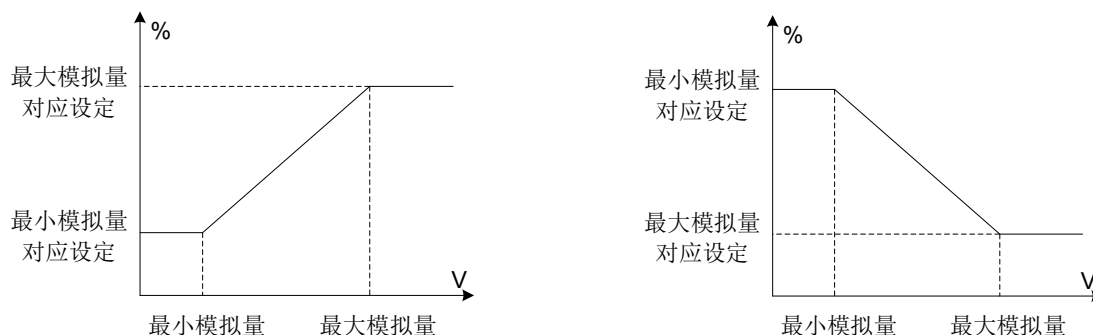
图6-18 模拟输入线性曲线
