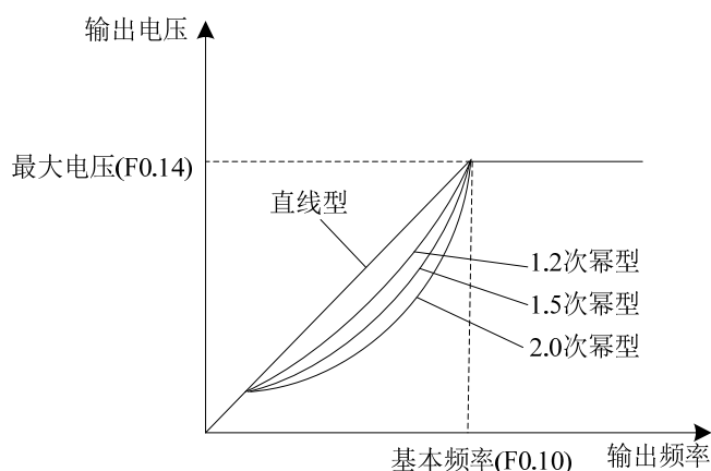
图6-8 V/F曲线示意图
