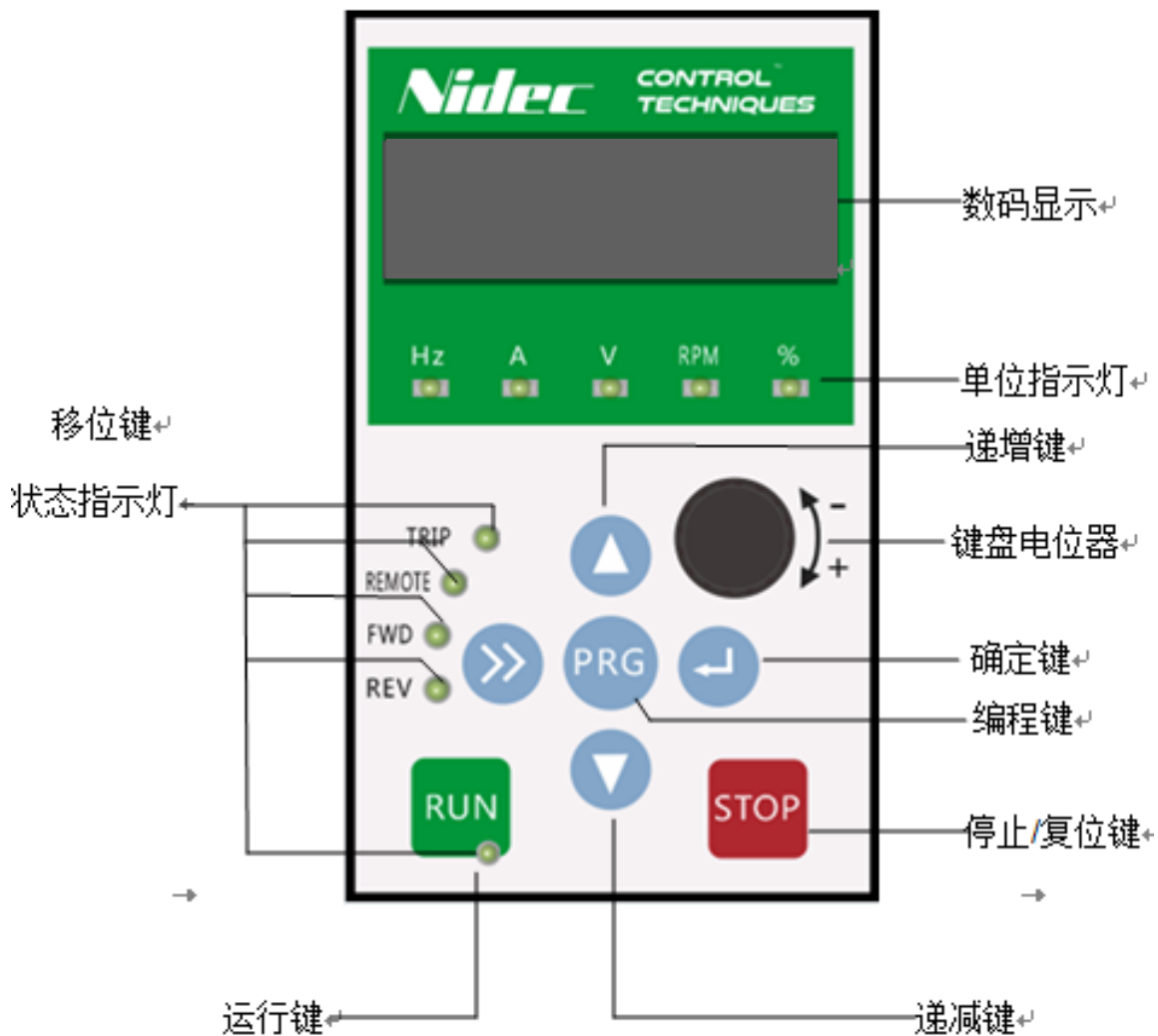
图 4-1 操作面板示意图
