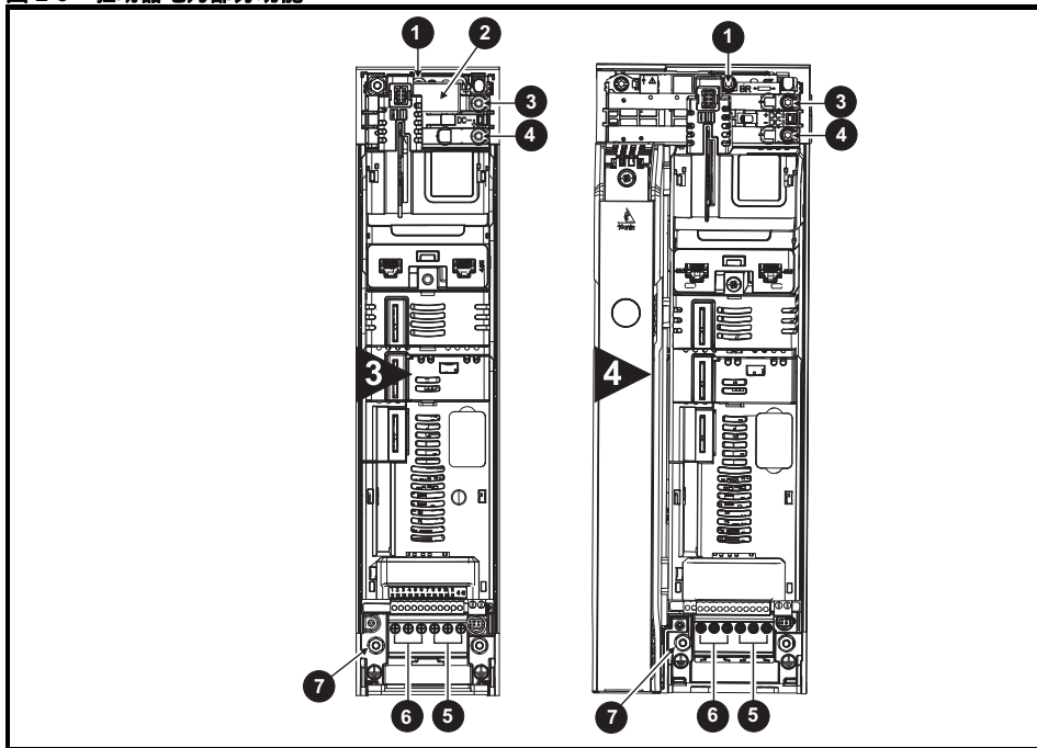
图 2-3 驱动器电力部分功能
