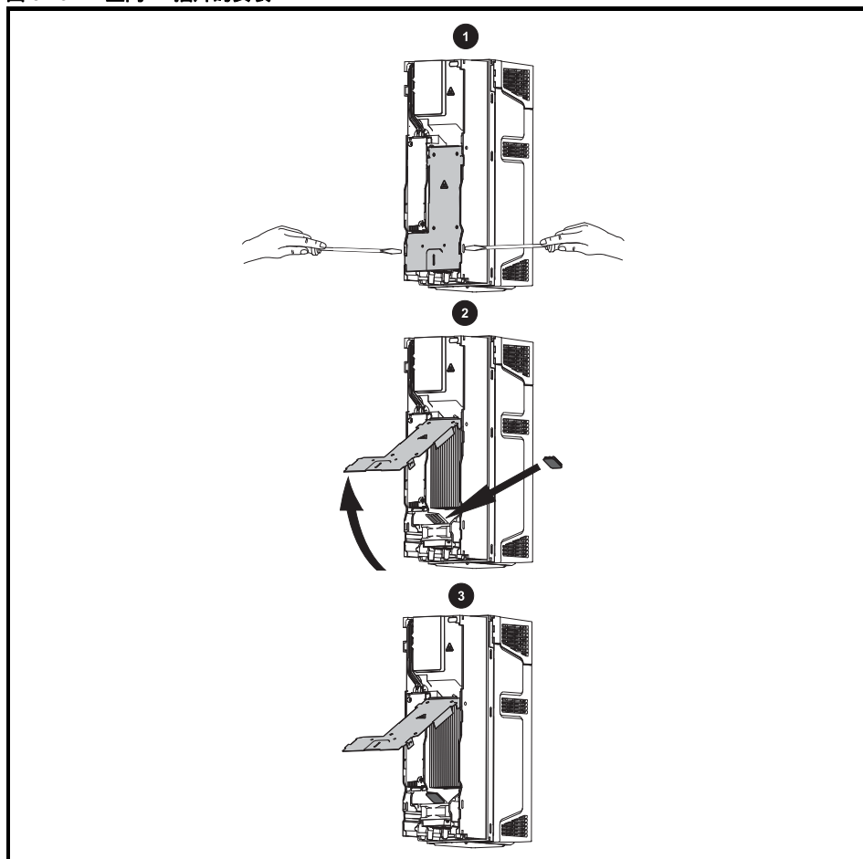
图 3-19 4 型高 IP 插片的安装
