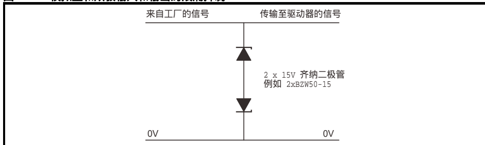
图 4-24 模拟量和双极输入和输出的浪涌抑制
