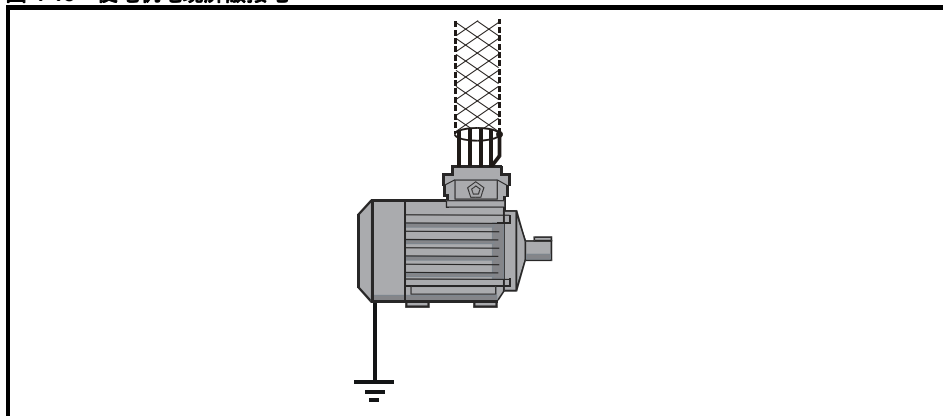
图 4-18 使电机电缆屏蔽接地
