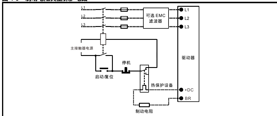
图 4-8 制动电阻典型保护电路
