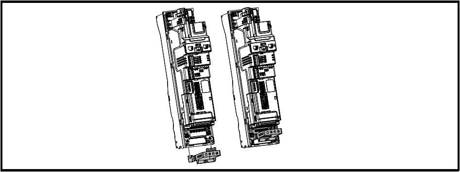
图 4-10 接地支架的安装（所有型号——所示为 3 型）
