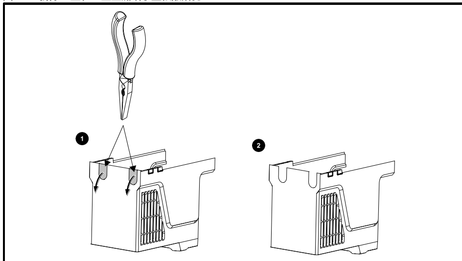
图 3-7 拆除 3 型和 4 型直流端子盖板敲落孔
