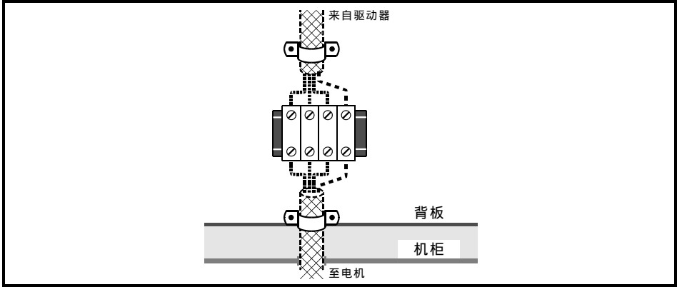
图 4-21 连接电机电缆至驱动器机柜内的端子排
