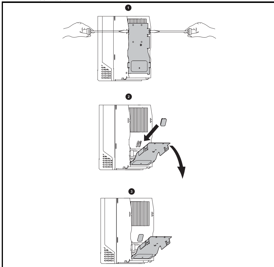
图 3-18 3 型高 IP 插片的安装
