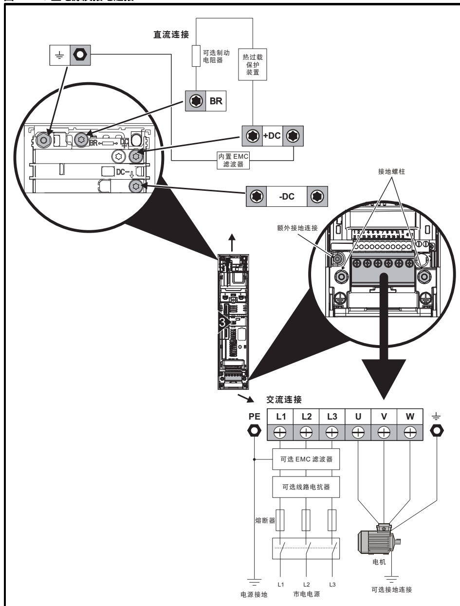
图 4-1 3 型电源及接地连接
