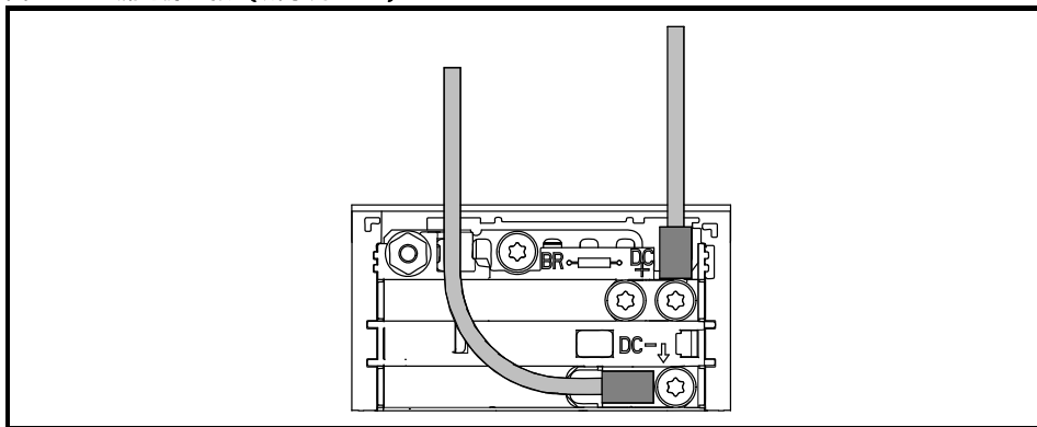
图 4-3 直流电源连接（所示为 3 型）
