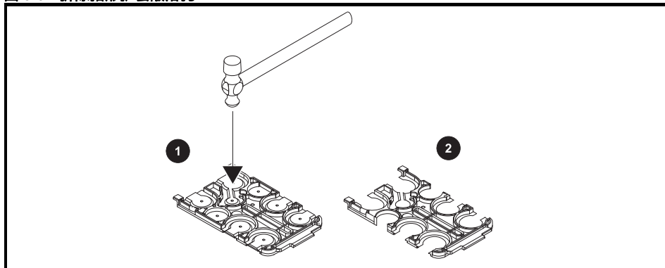
图 3-6 拆除指形护套敲落孔
