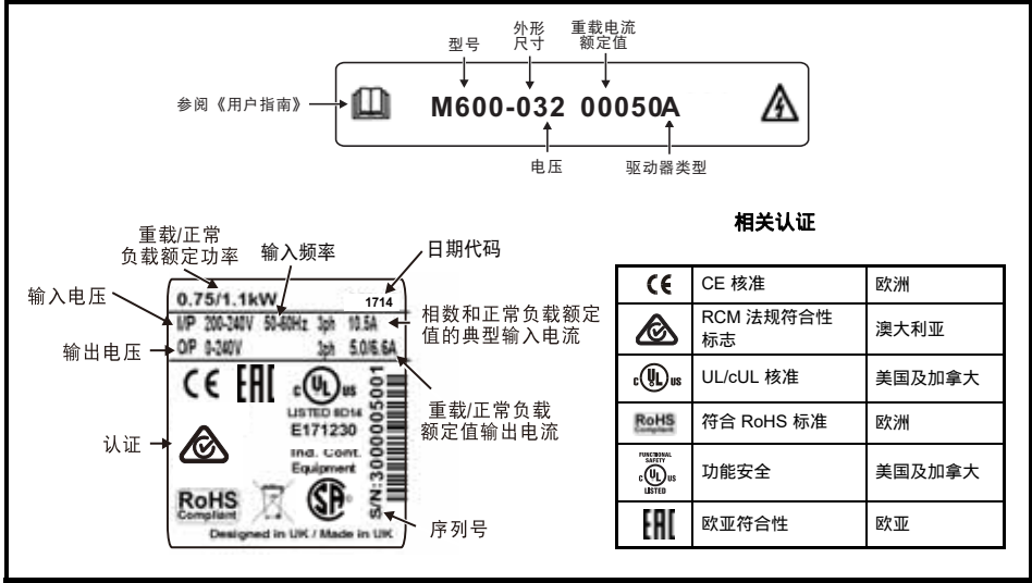
图 2-2 典型驱动器额定值标签
