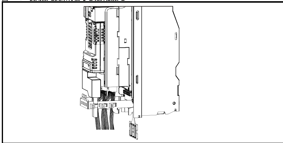
图 4-20 使用接地支架将信号电缆屏蔽接地
