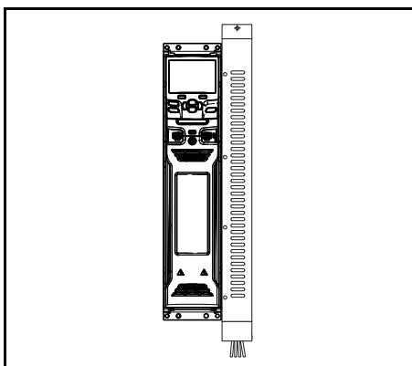
图 3-26 书架式安装 EMC 滤波器
