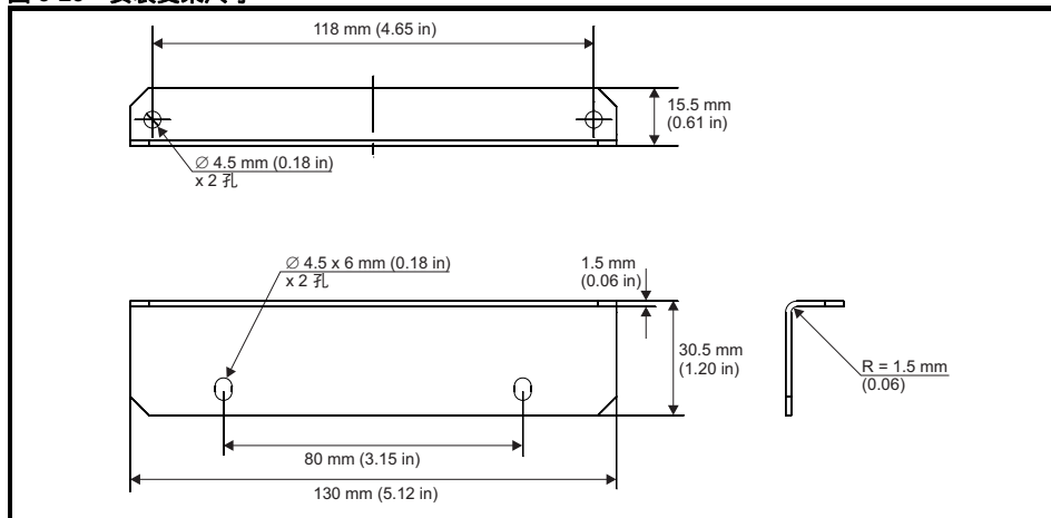
图 3-23 安装支架尺寸
