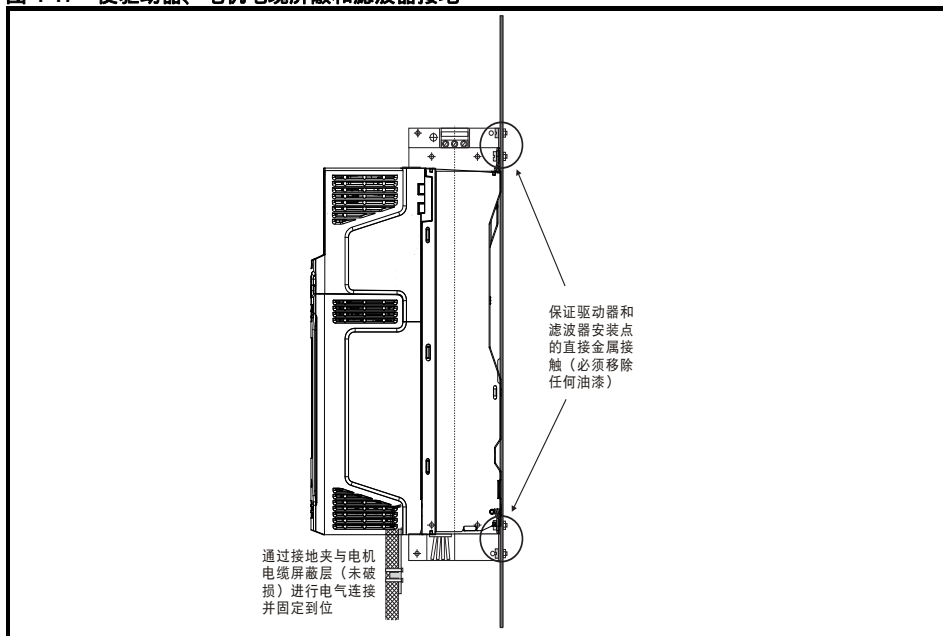
图 4-17 使驱动器、电机电缆屏蔽和滤波器接地
