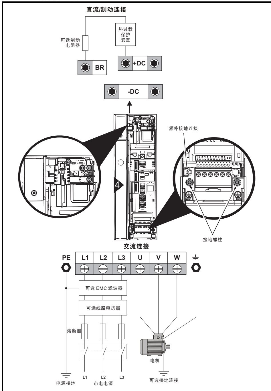
图 4-2 4 型电源及接地连接
