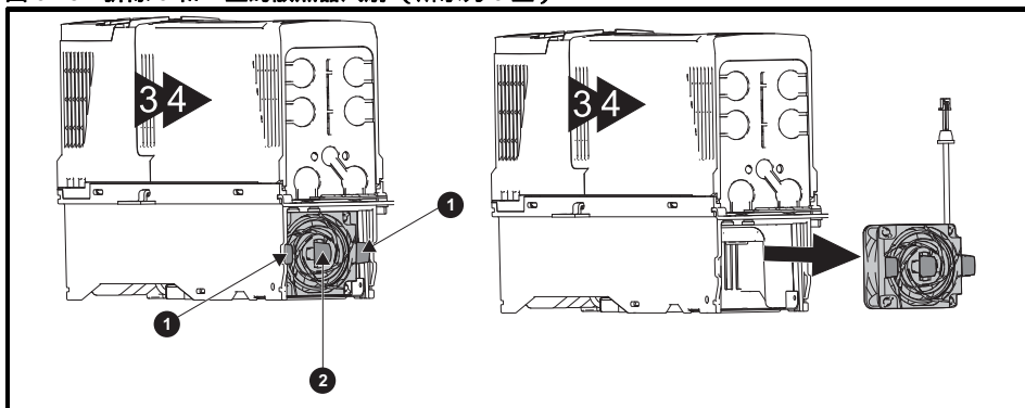
图 3-28 拆除 3 和 4 型的散热器风扇（所示为 3 型）
