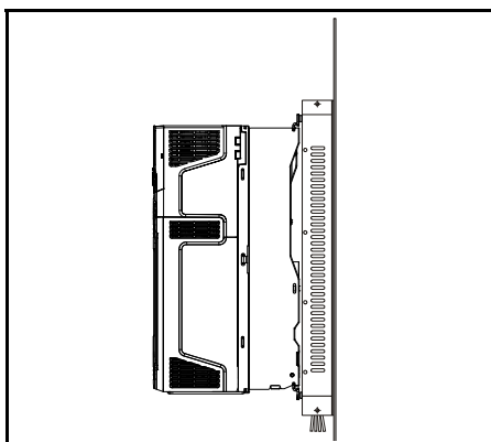
图 3-25 脚架式安装 EMC 滤波器
