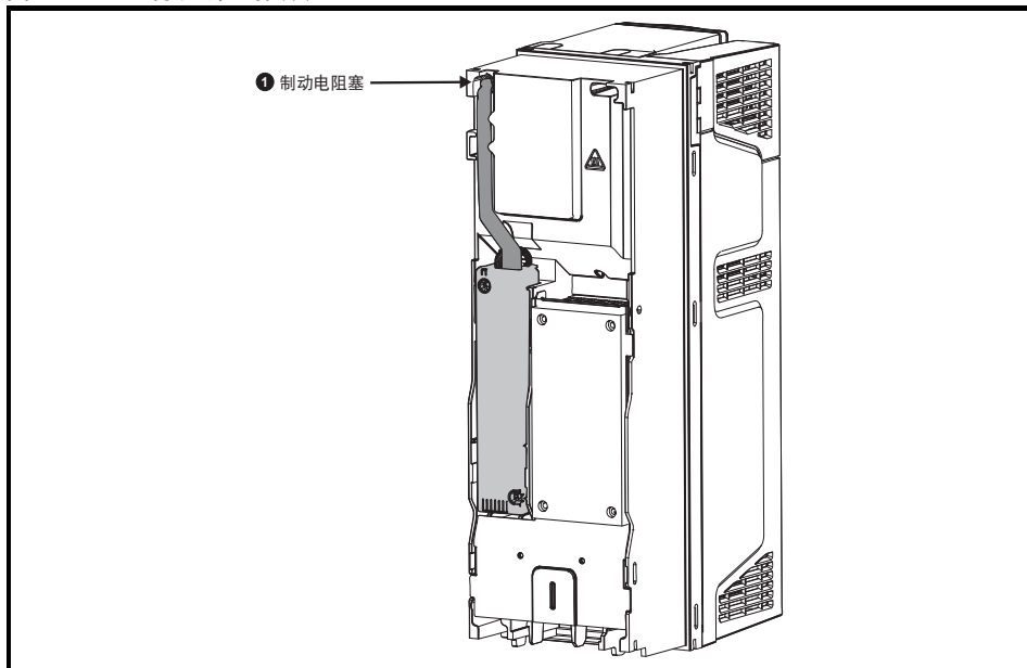
图 3-21 4 型制动电阻的安装
