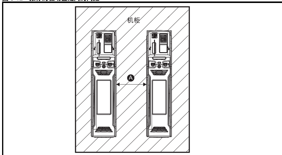
图 3-12 推荐的驱动器之间的间距
