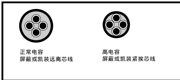
图 4-5 影响电容的电缆结构
