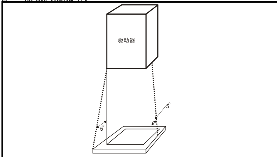
图 3-1 防火防护机柜底部布局
