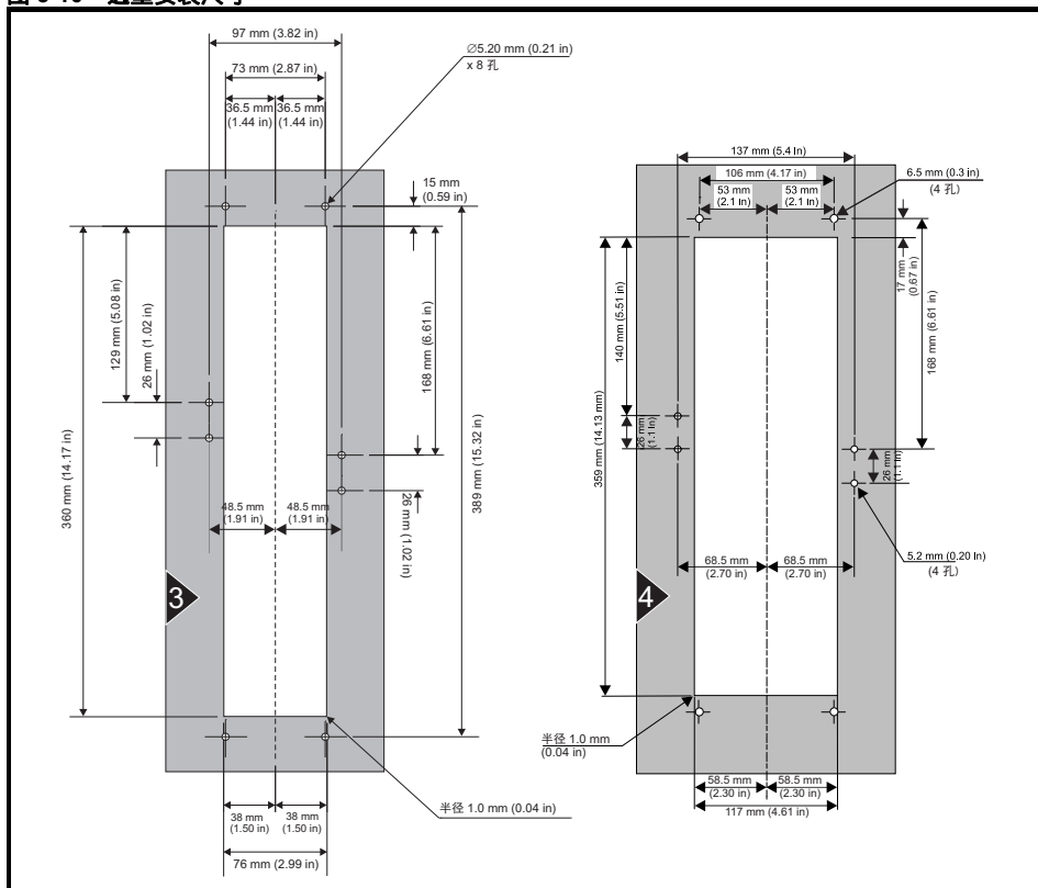
图 3-10 透壁安装尺寸
