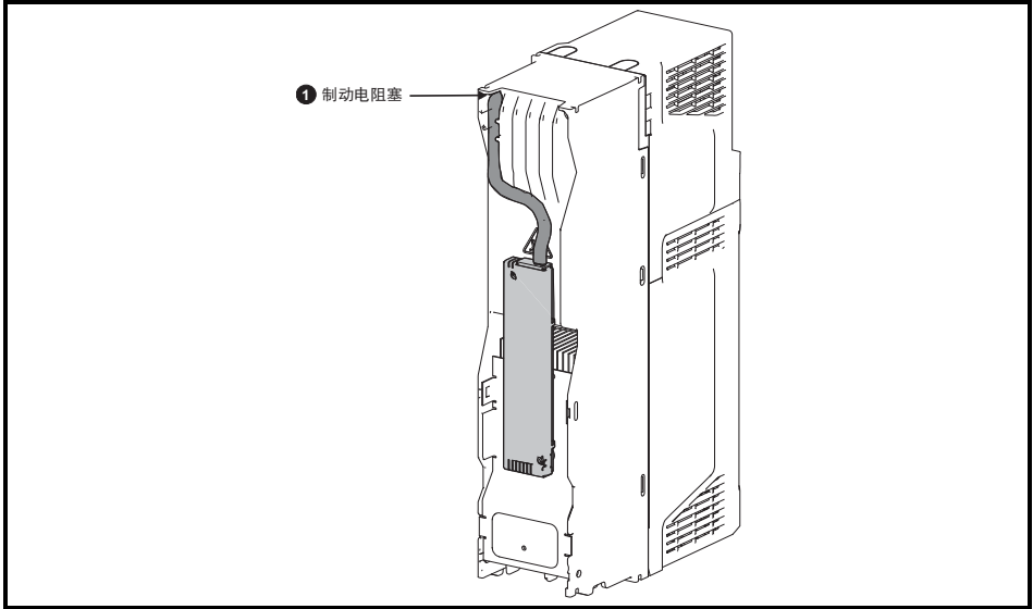
图 3-20 3 型制动电阻的安装
