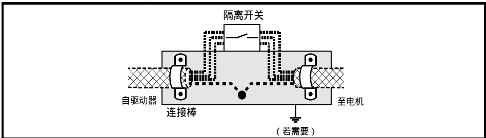
图 4-22 将电机电缆连接到隔离 / 断路器
