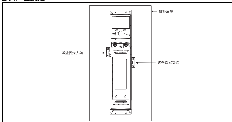
图 3-17 透壁安装
