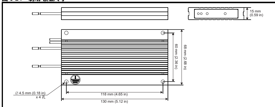
图 3-24 制动电阻尺寸
