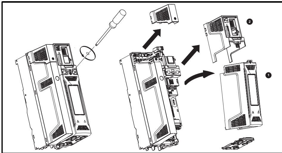
图 3-5 拆除 4 型端子盖板
