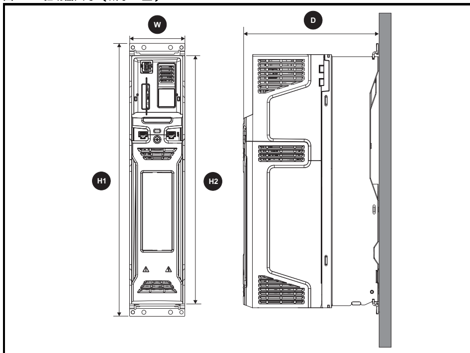
图 3-8 驱动器尺寸（所示 3 型）
