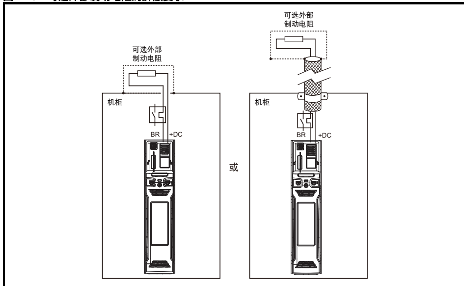
图 4-19 可选外部制动电阻的屏蔽要求
