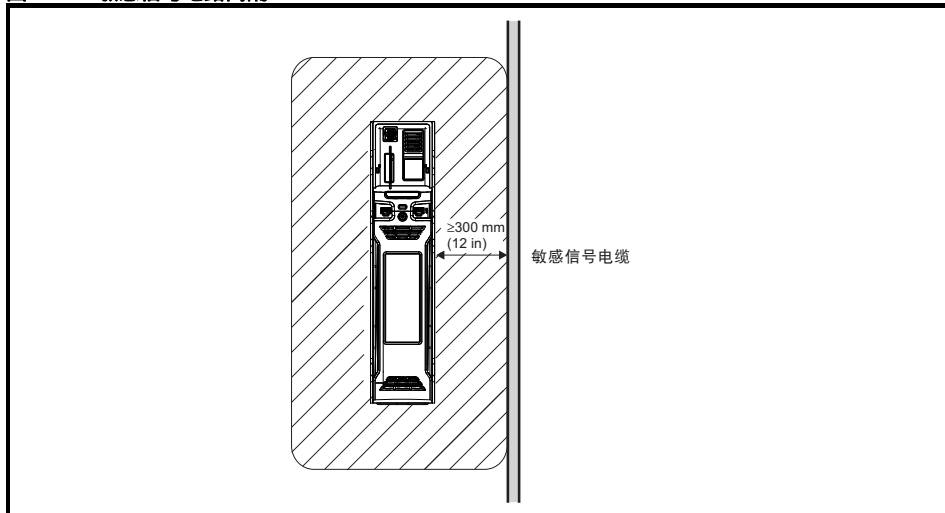
图 4-16 敏感信号电路间隔
