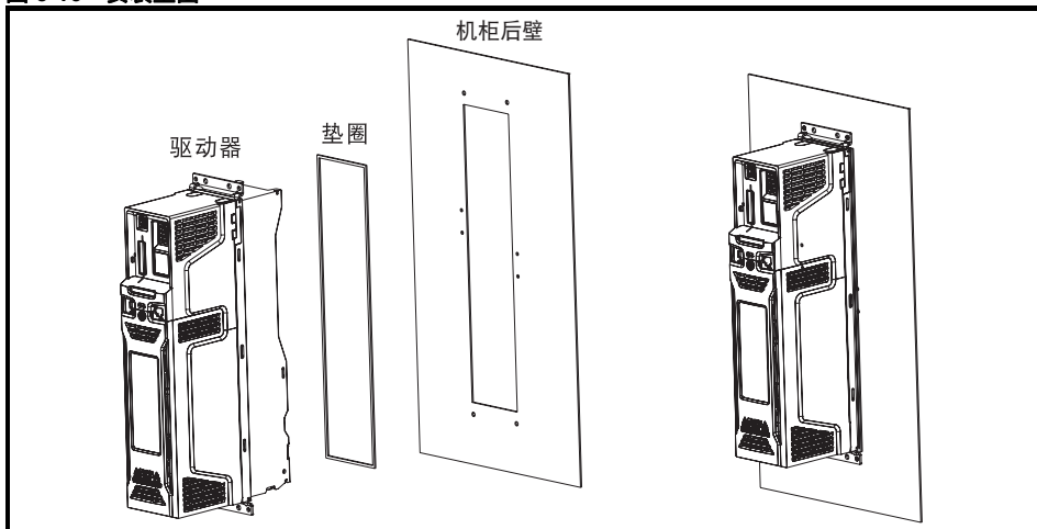
图 3-16 安装垫圈
