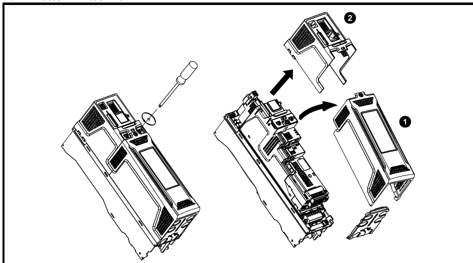
图 3-4 拆除 3 型端子盖板
