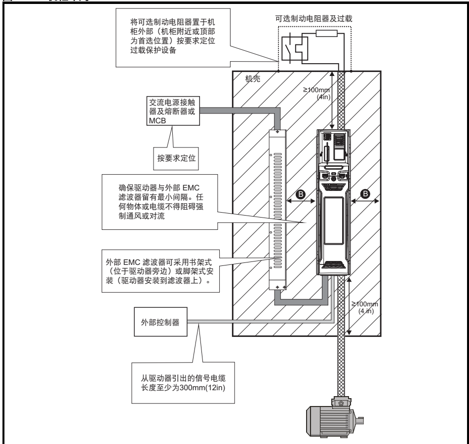
图 3-13 机柜布局
