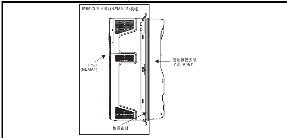
图 3-15 IP65 示例 (3 至 4 型) (NEMA 12) 通孔布局
