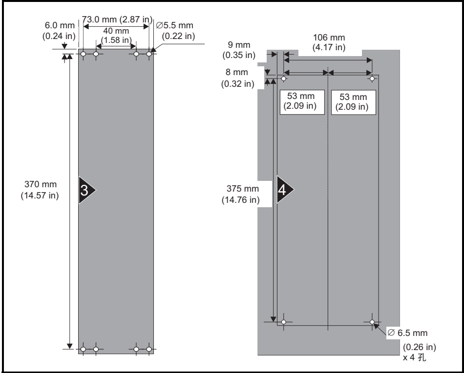
图 3-9 表面安装尺寸
