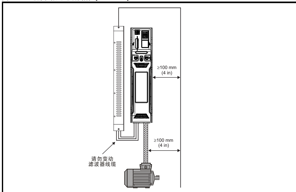
图 4-15 电源和接地电缆间隔（3 至 4 型）
