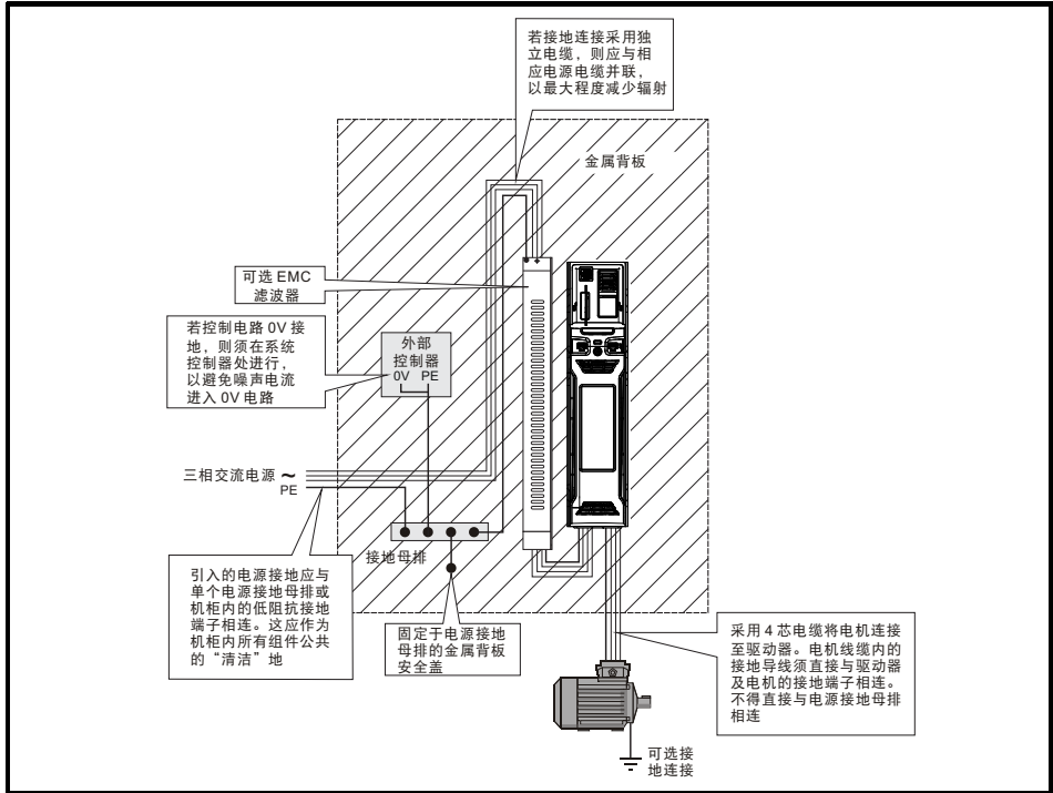
图 4-13 一般 EMC 机柜布局显示接地连接
