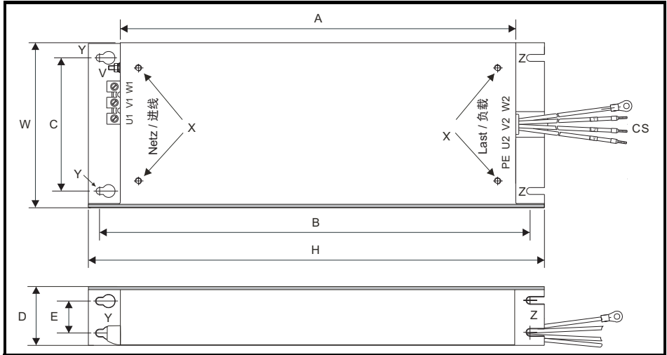
图 3-27 外部 EMC 滤波器
