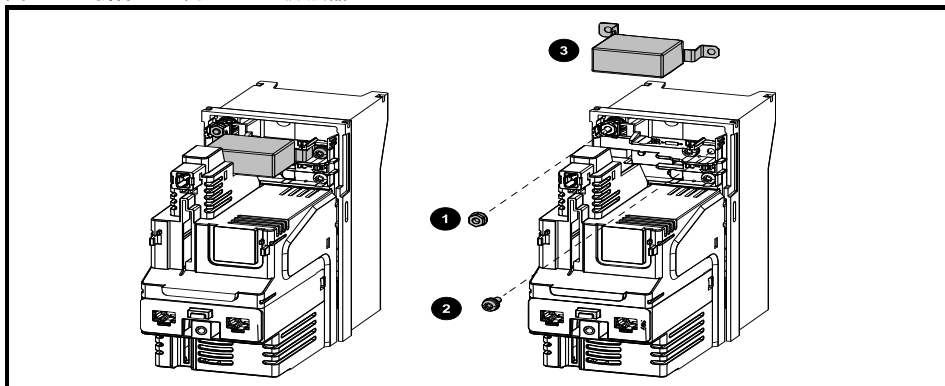
图 4-11 拆除 3 型内置 EMC 滤波器
