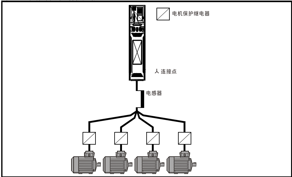
图 4-7 针对多台电机的备用连接
