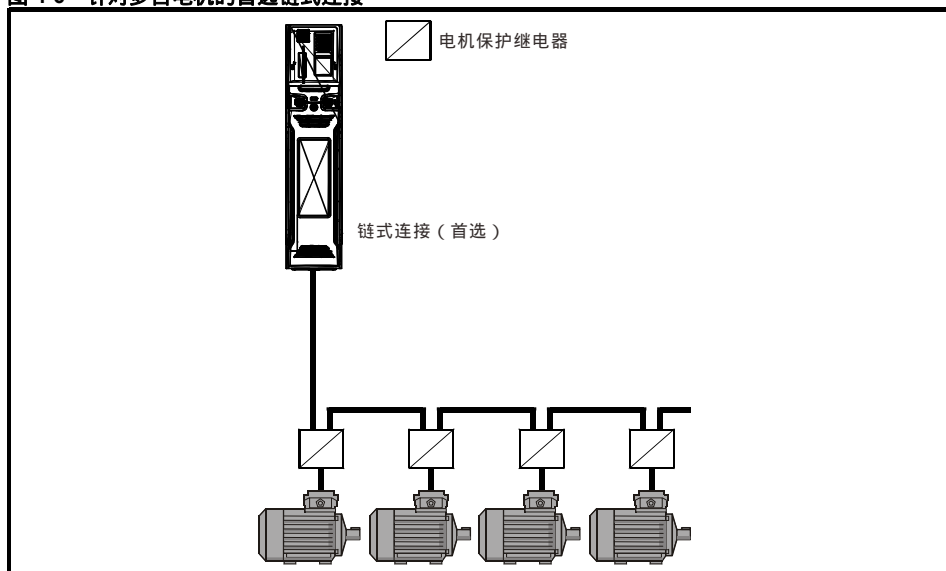
图 4-6 针对多台电机的首选链式连接
