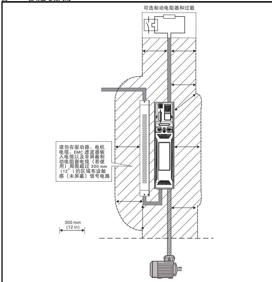
图 4-14 驱动器电缆间隔
