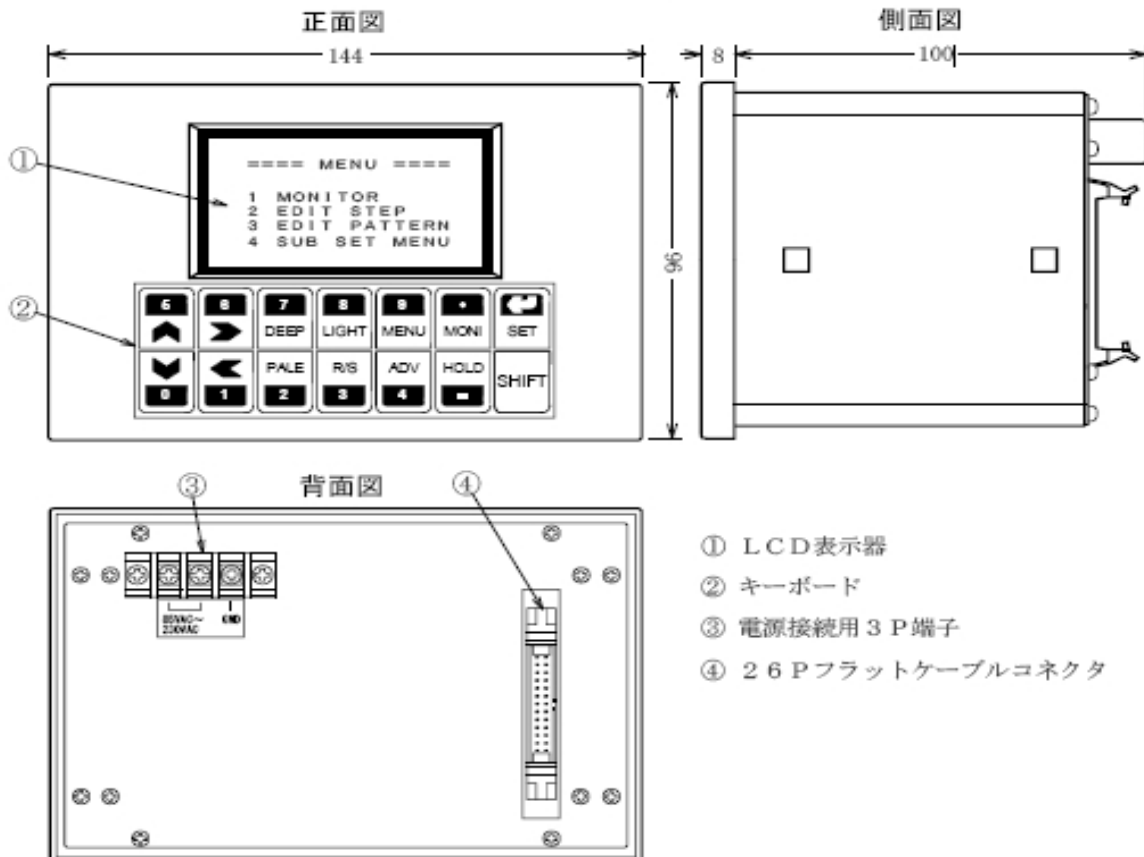
①.LCD顯示器 ②.按鍵 ③.電源端子 ④.26PIN排線插座
