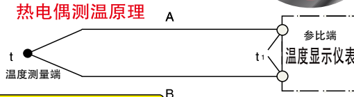
热电偶测温原理
