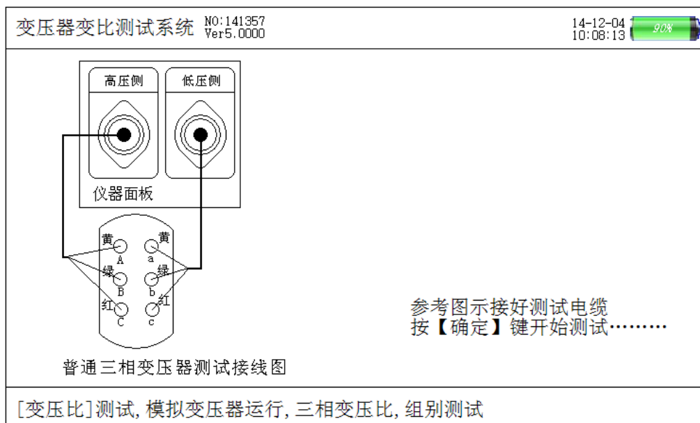
图五、三相变压比测试接线提示屏
