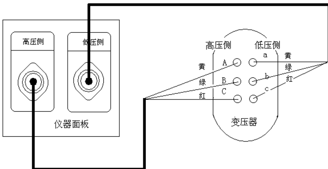
图十八、三相变压器的测试接线
