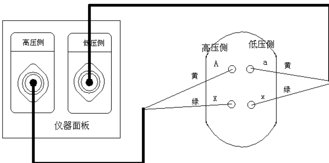
图十九、单相变压器的测试接线
