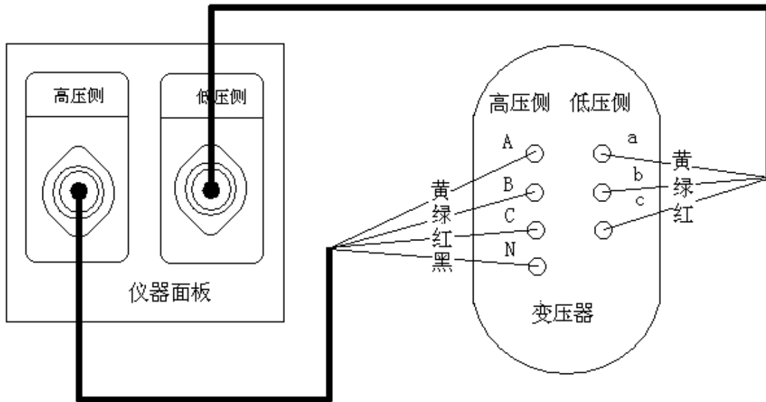
图二十二、Z 型变的测试接线
