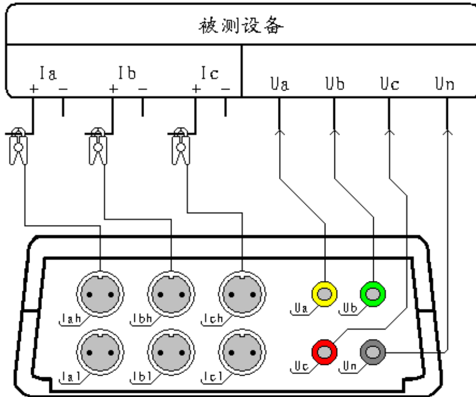
图二十五、谐波测试接线图
