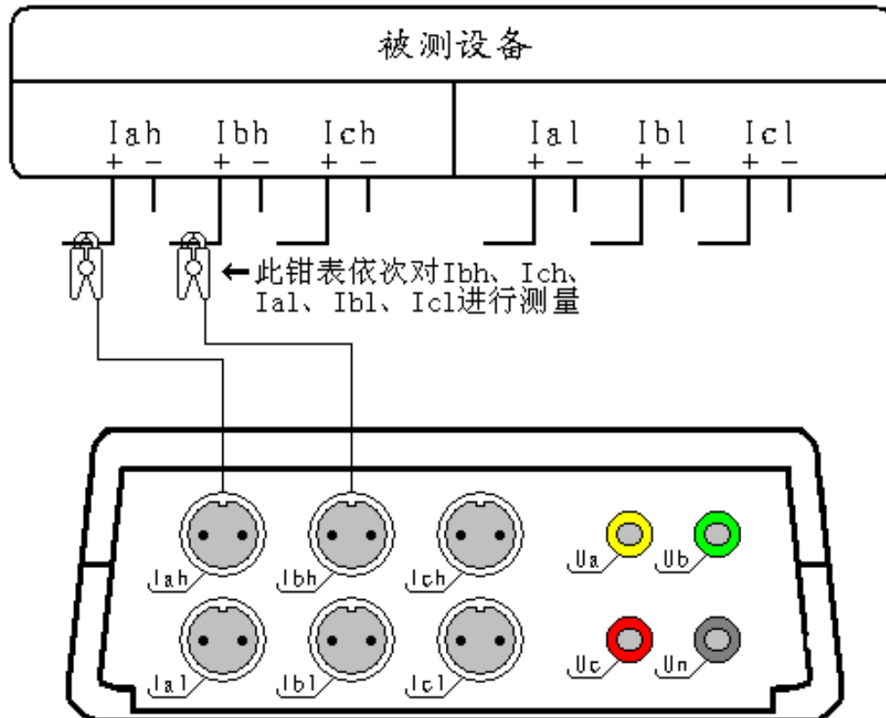
图二十一、双钳差动接线
