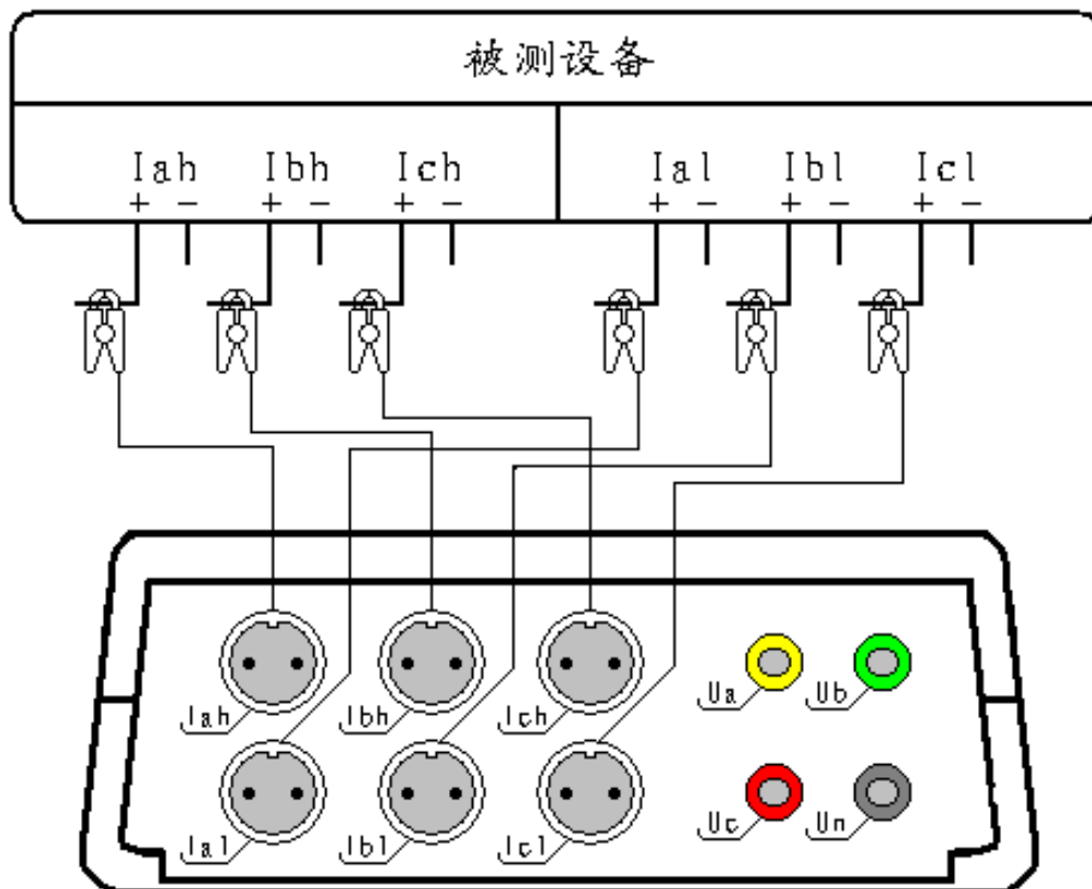
图二十、六钳差动接线
