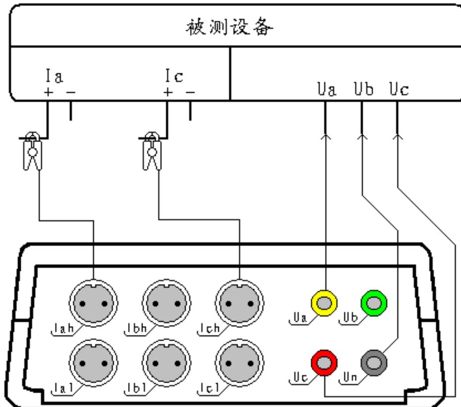
图二十二、三线计量矢量测试
