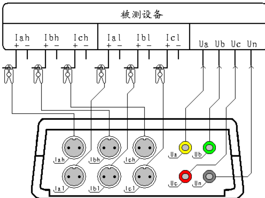
图二十三、波形显示接线图
