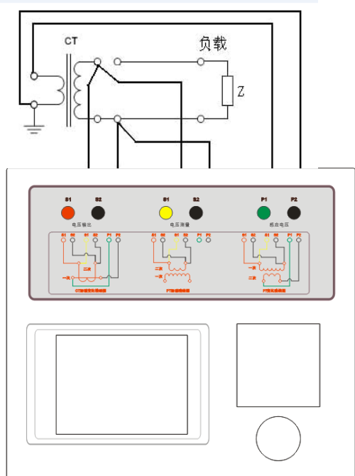
图 2.1 CT 直阻、励磁、变比试验接线方式
