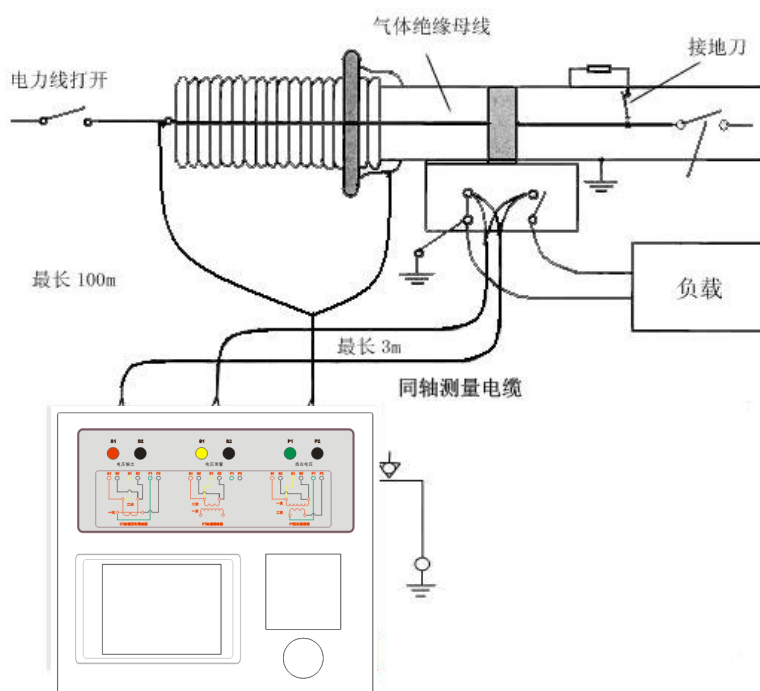
图 C.4 测试仪对 GIS (SF6) 开关上的 CT 测试时的接线方式
