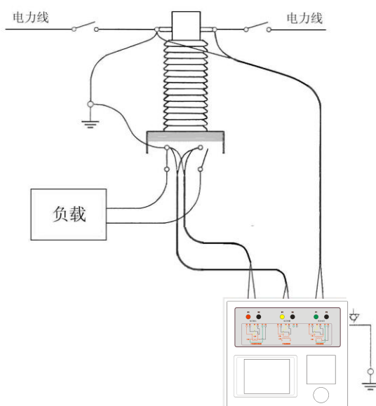
图 C.1 典型接线方式
