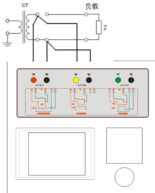
图 2.2 CT 二次负荷试验接线方式
