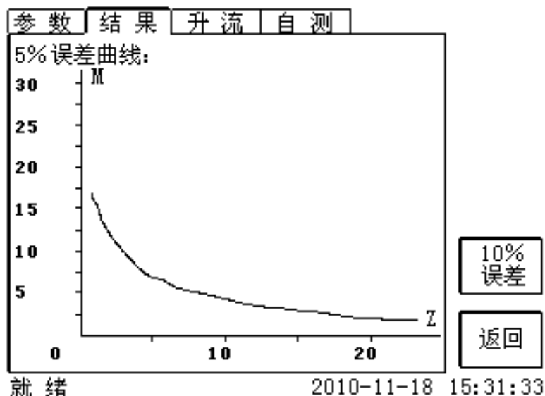
图 2.14 5%误差曲线界面
