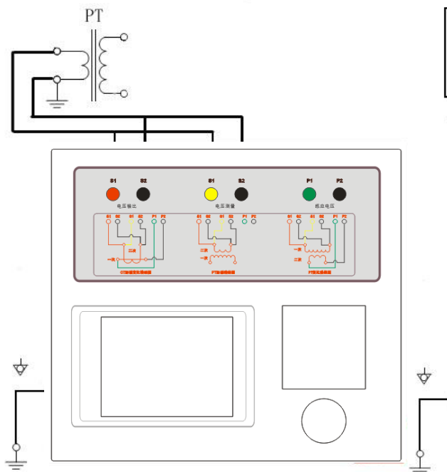
图 2.7 PT 直阻、励磁试验接线方式
