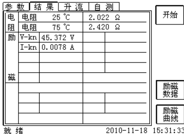
图 2.6 P 级 PT 的试验结果界面
