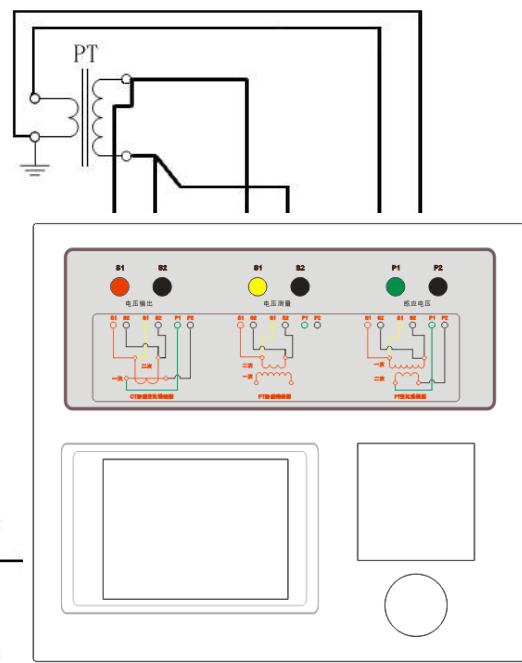
图 2.8 PT 变比、极性试验接线方式
