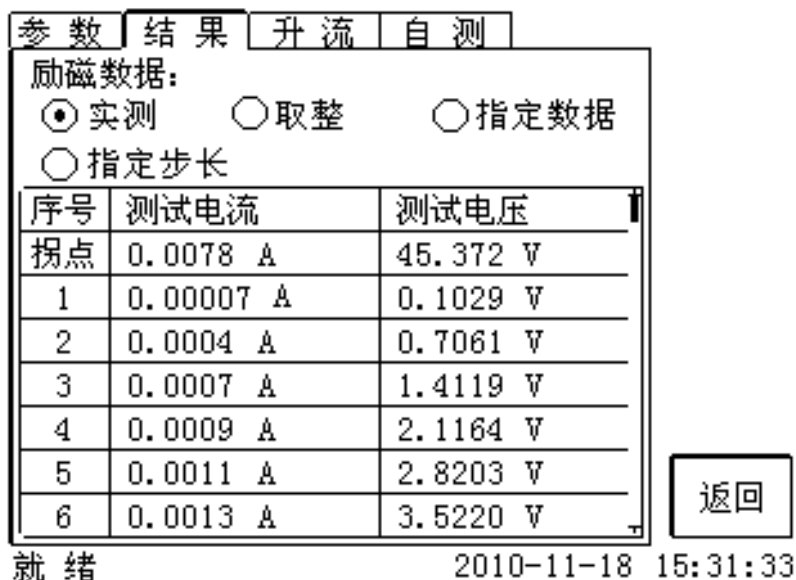
图 2.15 励磁数据界面
