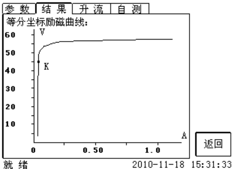
图 2.16 励磁曲线界面
