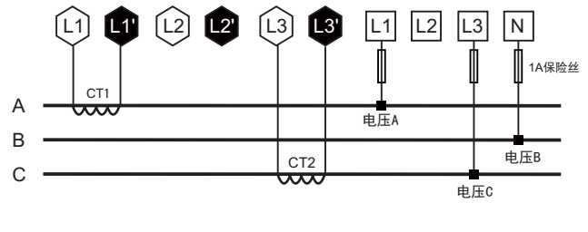
三相三线
