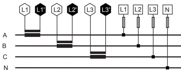
三相四线
