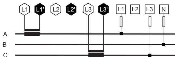
三相三线
