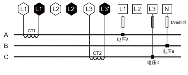
三相三线
