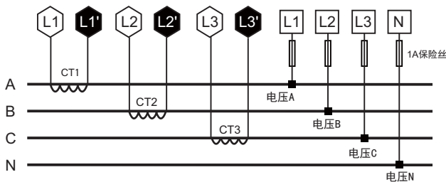
三相四线
