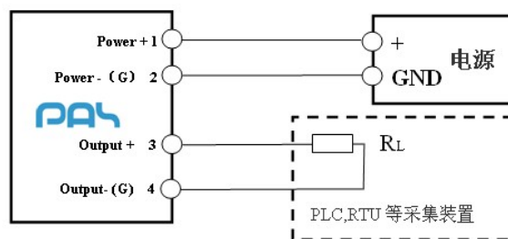
接线示意图
