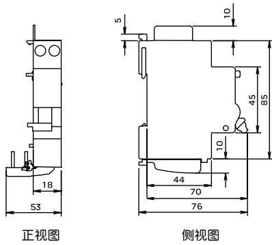
正视图
