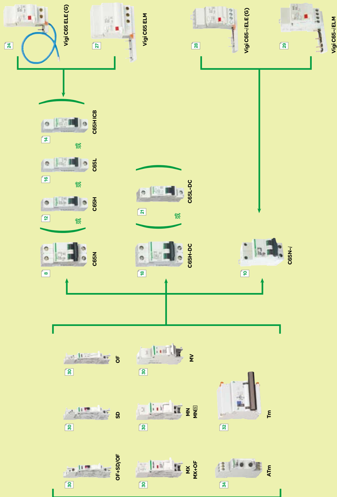
附件拼装示意图
