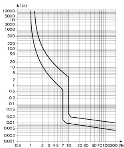
C65H-DC / C65L-DC C型脱扣曲线
