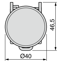
正视图
