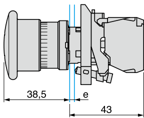
蘑菇头按钮, 弹簧返回 XB4-BC21
