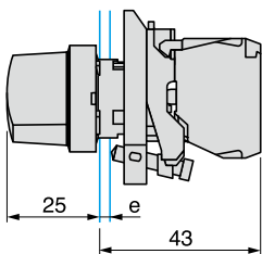
选择开关 标准操作手柄 XB4-BD
