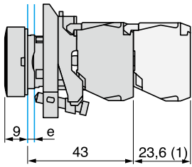
按钮, 弹簧返回 XB4-BA**
