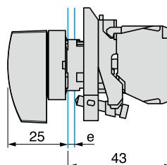
长操作手柄 XB4-BJ
