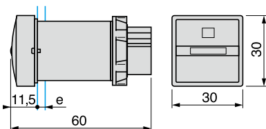
小时计数器 XB5-DS..
