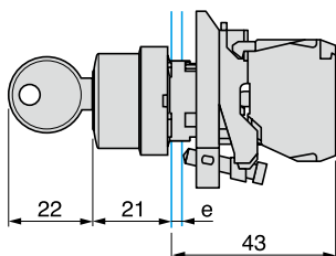
钥匙开关 XB4-BG
