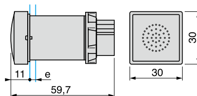
报警器 XB5-KS..
