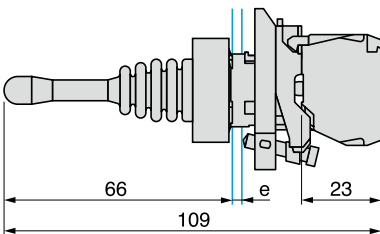
操作杆 XD4-PA..2
