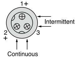
接线图 XB5-KS..
