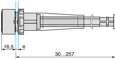
手动过载复位按钮 XB4-BA9..
