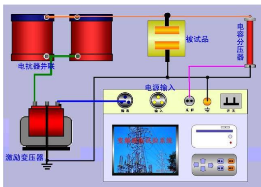
接线示意图：
