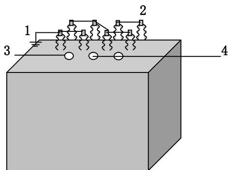
二串二并 1 \times 2 \mu \times 2
