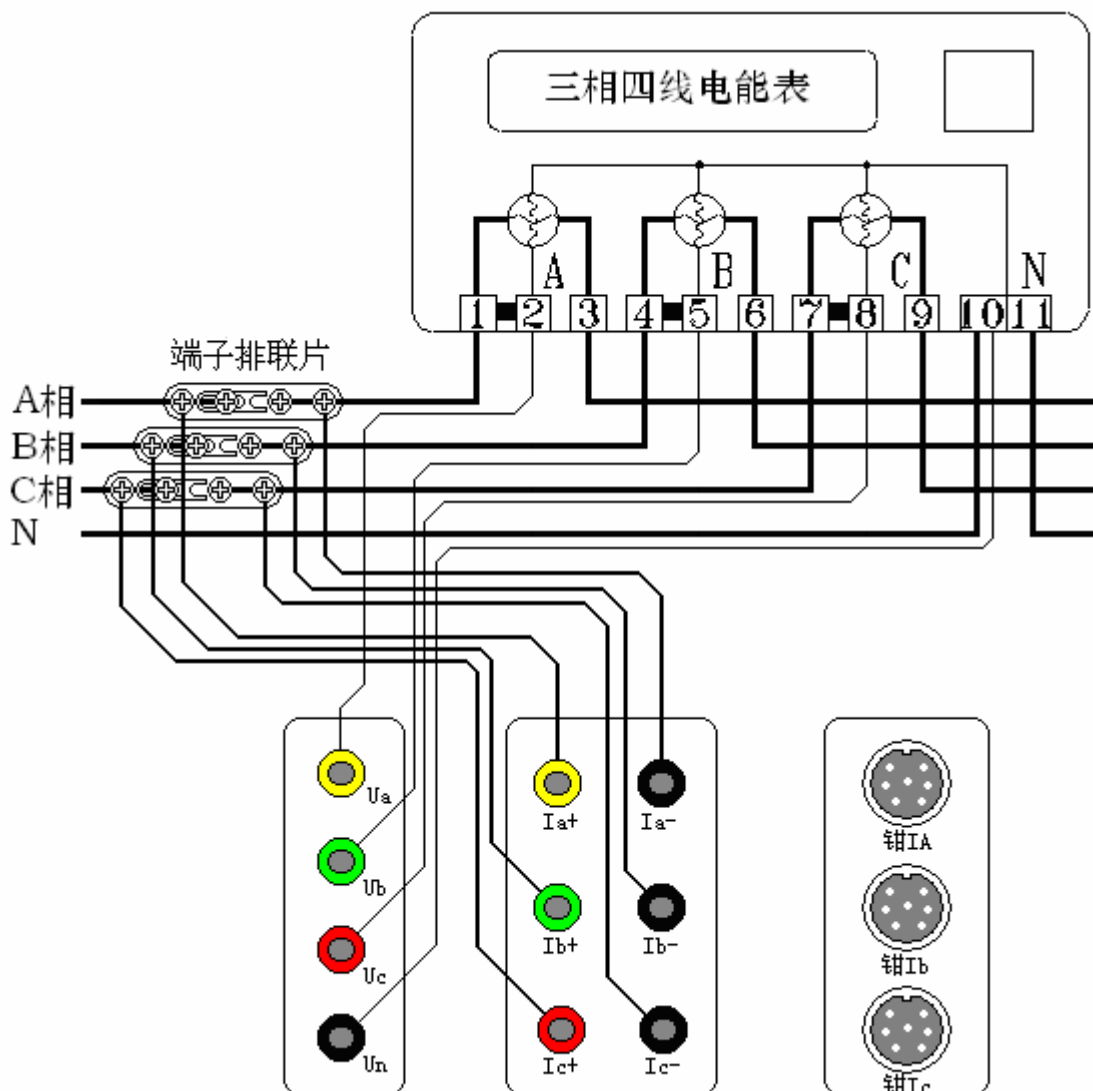
图二十二、三相四线直接接入测试
