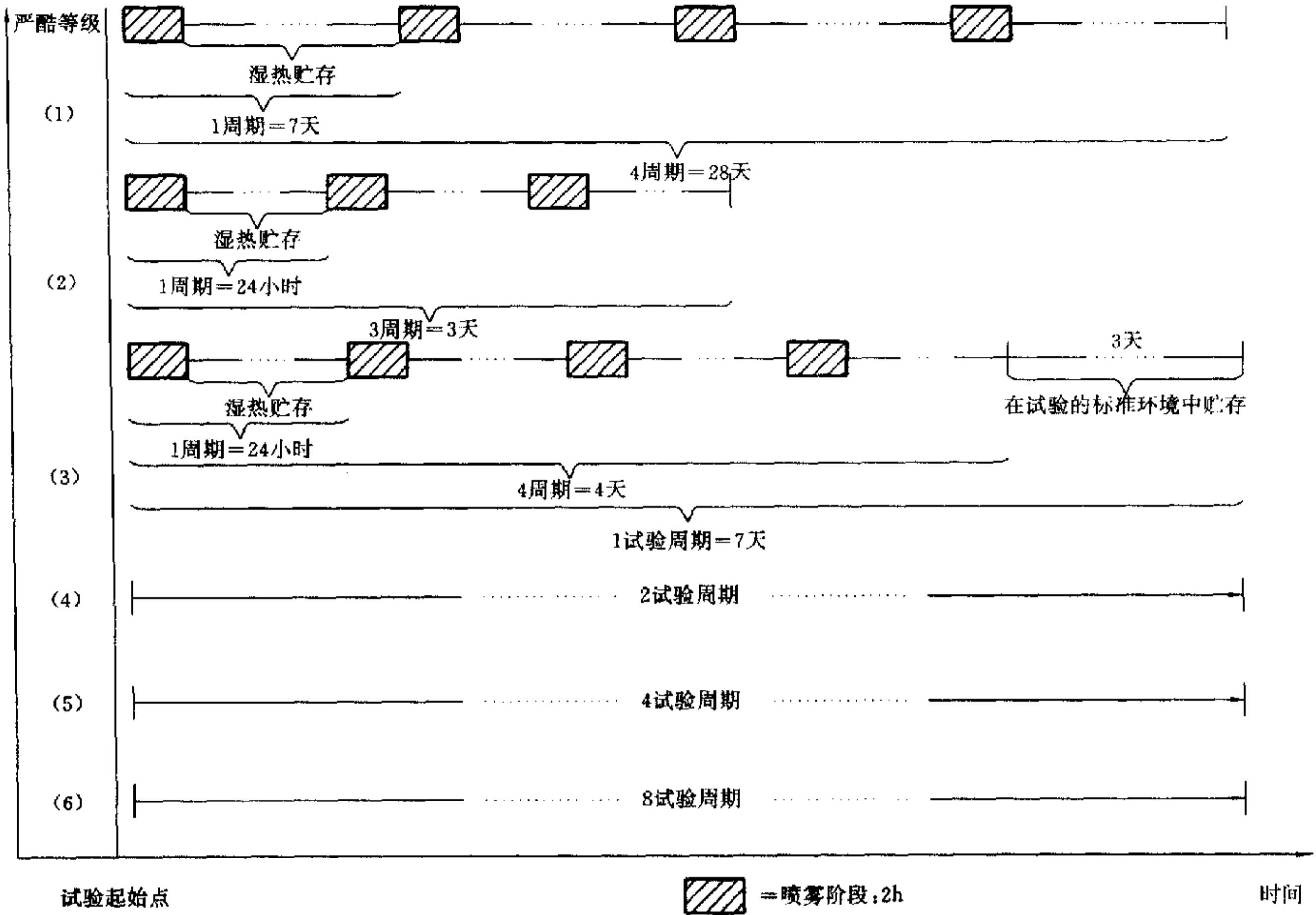
图 1 不同试验严酷等级(1)~(6)的时标示意图
