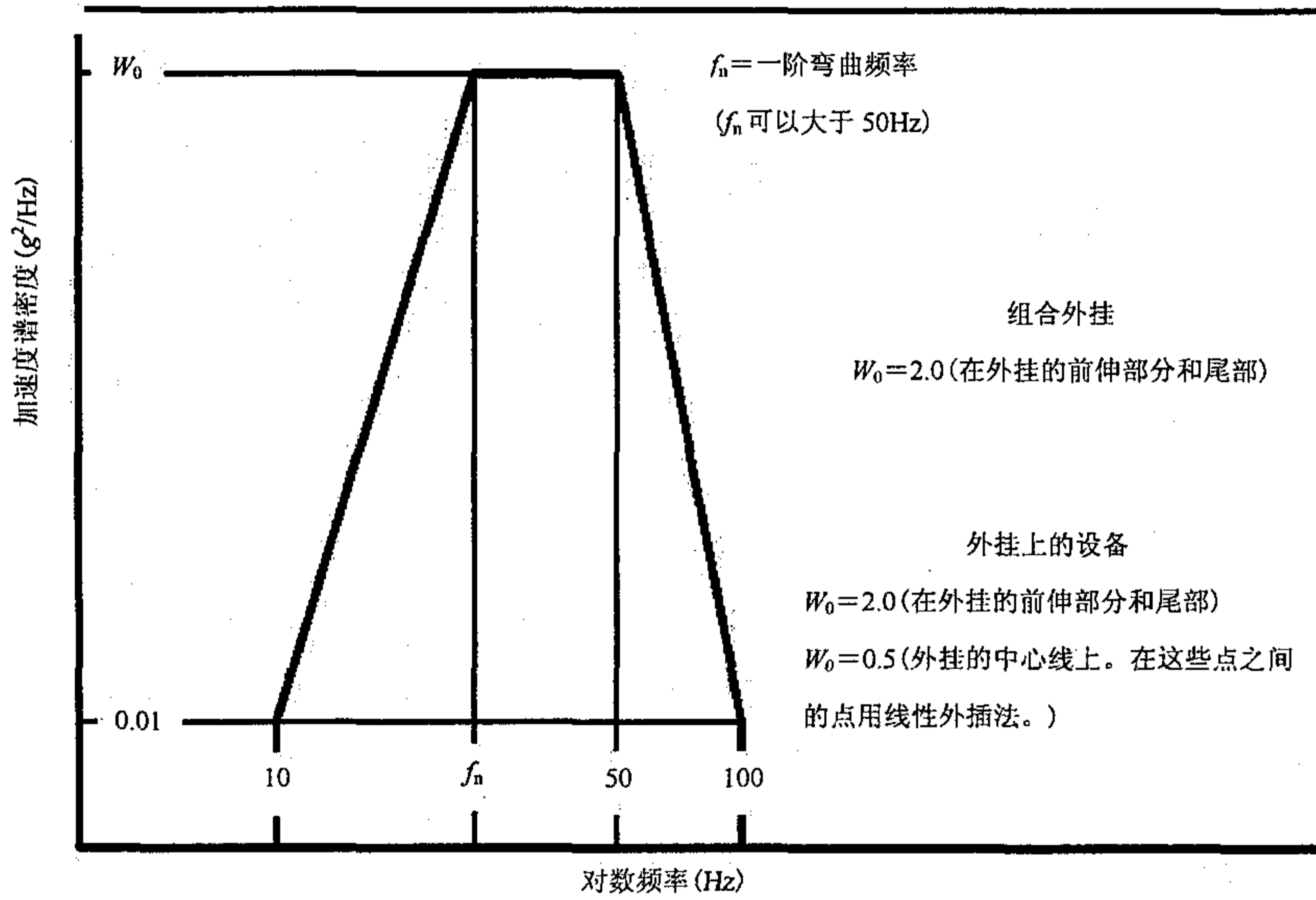
图 C.13 喷气式飞机外挂抖振响应
